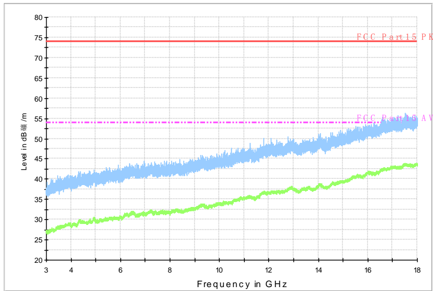
RE - 3GHz-18GHz
