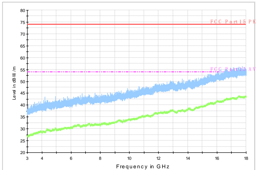
RE - 3GHz-18GHz
