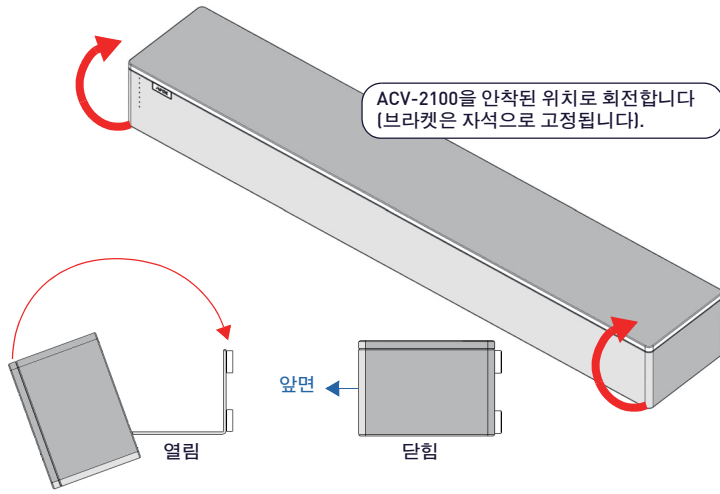
그림 6 ACV-2100을 안착된 위치로 회전
