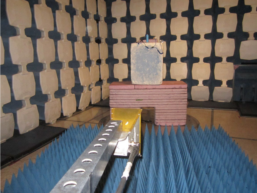
1GHz – 6GHz
