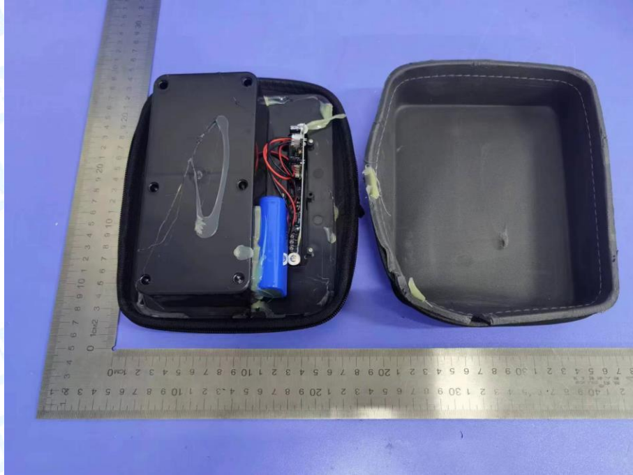
Photo 13 Battery parameters
