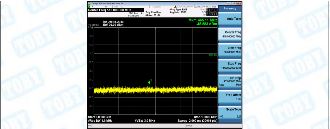
Band4-1413-2-1000~20000MHz
