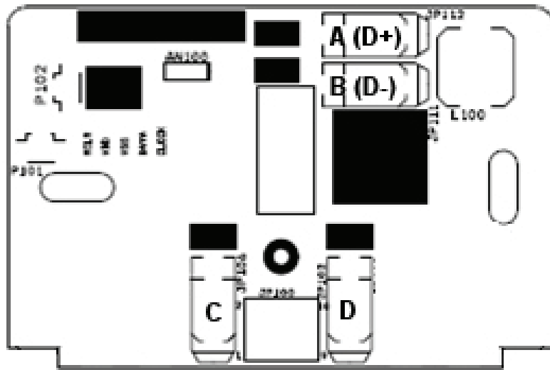
Fig. 3 – Backplate
