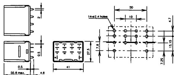
RH4V2-U/RH4V2-UL/RH4V2-UD
