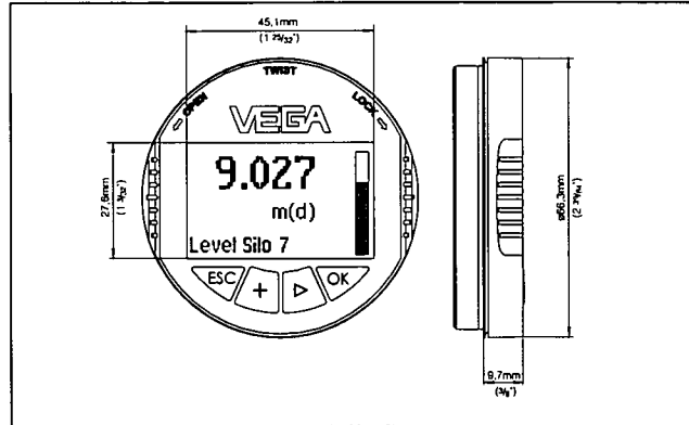
Fig. 28: PLICSCOM
