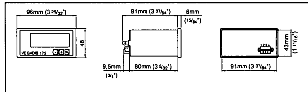
Fig. 29: VEGADIS 175
