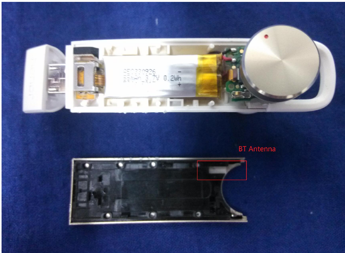
(2) EUT Photo
