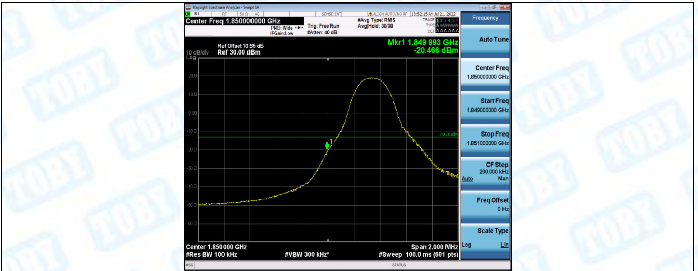
Band2-5MHz-QPSK-18625-1RB#24
