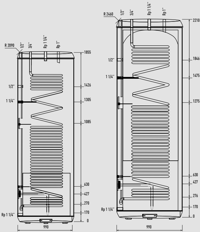
PAW-VP750LDHW-1
