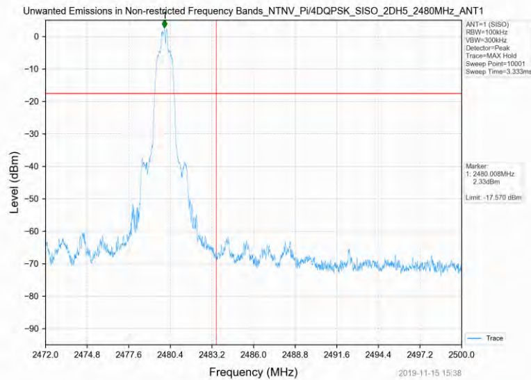
Pi/4DQPSK_2480MHz_2DH5_SISO_ANT1
