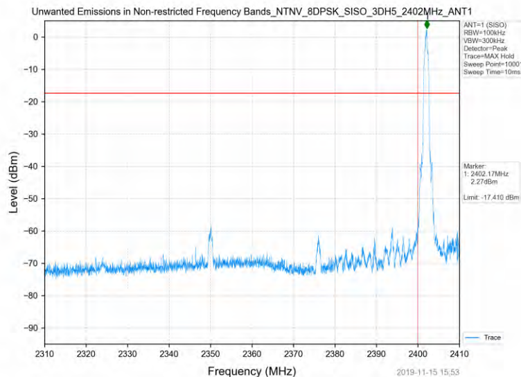
8DPSK_2402MHz_3DH5_SISO_ANT1
