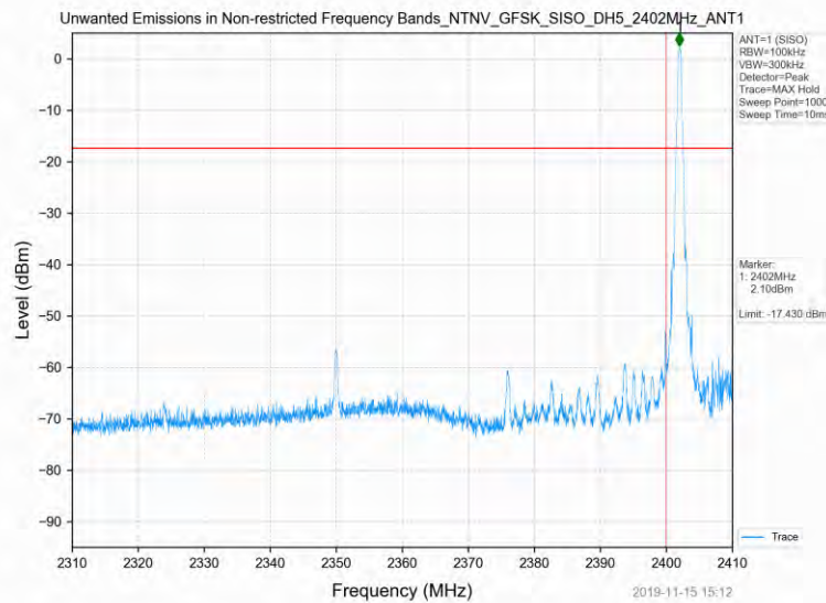
GFSK_2402MHz_DH5_SISO_ANT1
