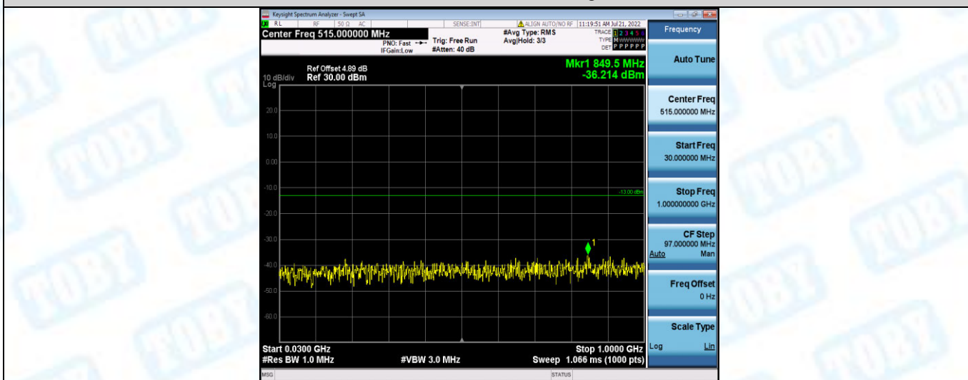
Band2-10MHz-QPSK-19150-1RB#0-Range2:1000~20000MHz
