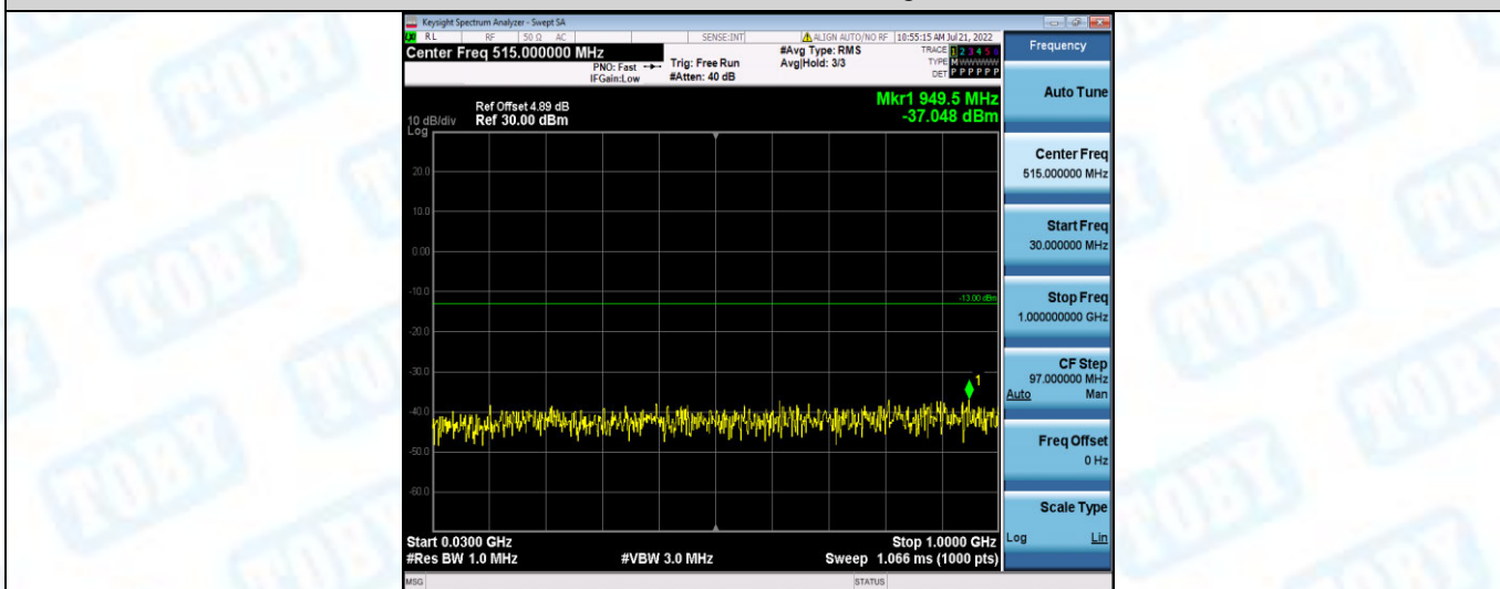
Band2-5MHz-QPSK-18900-1RB#0-Range2: 1000~20000MHz
