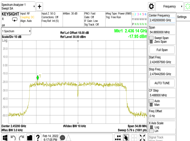
802.11ax_40MHz_Chain1_2452MHz
