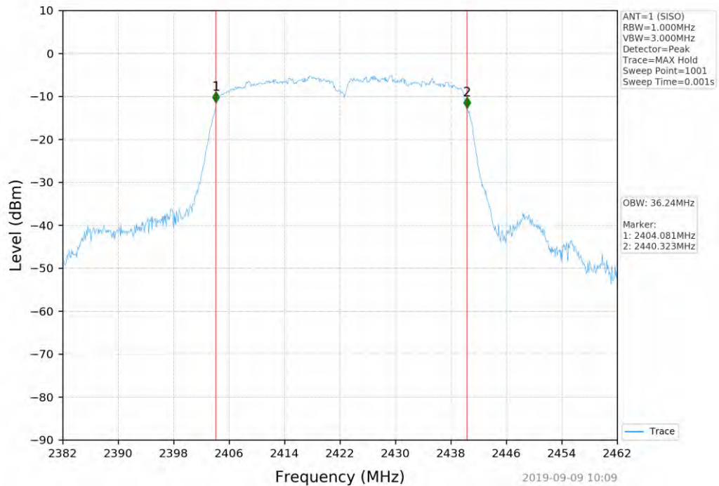
802.11n(HT40)_2422MHz_SISO_ANT1
