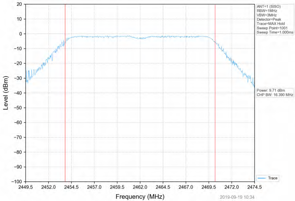
802.11g_2462MHz_SISO_ANT1
