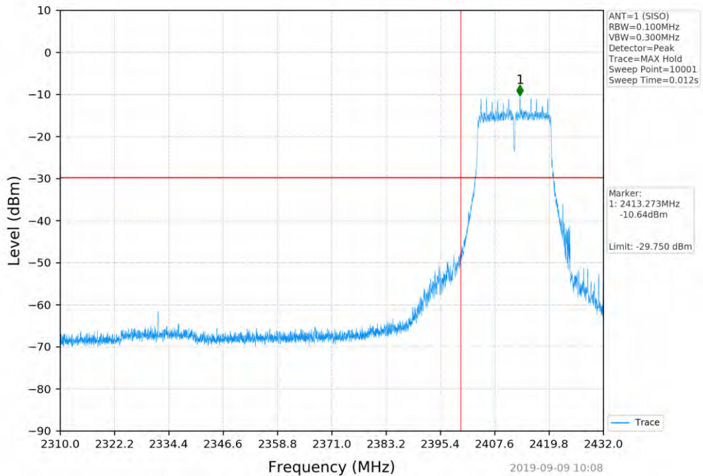
802.11g_2412MHz_SISO_ANT1
