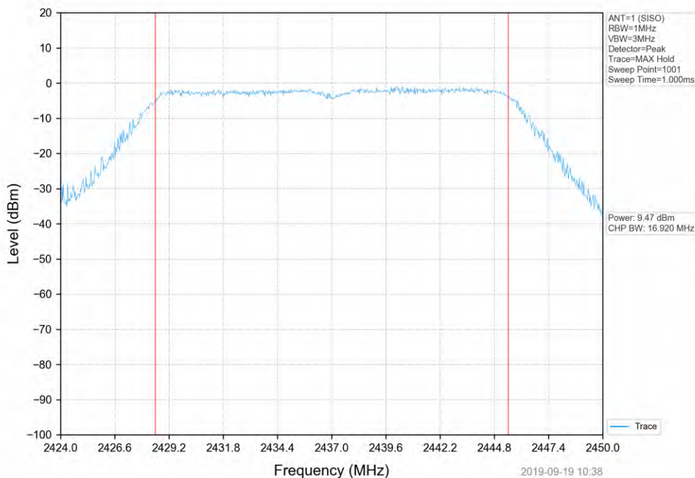
802.11n(HT20)_2437MHz_SISO_ANT1
