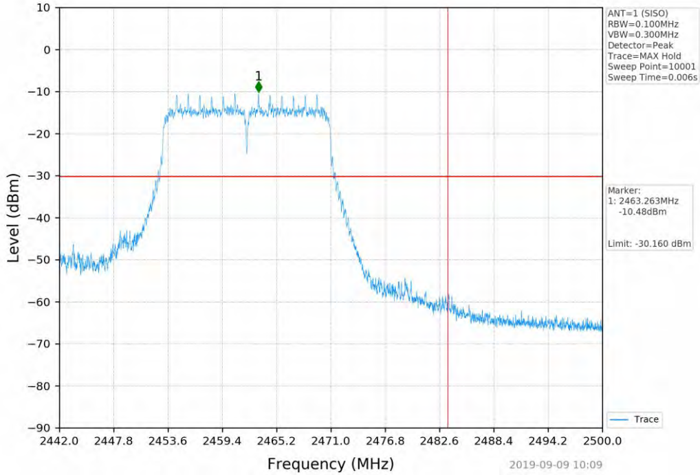
802.11n(HT20)_2462MHz_SISO_ANT1
