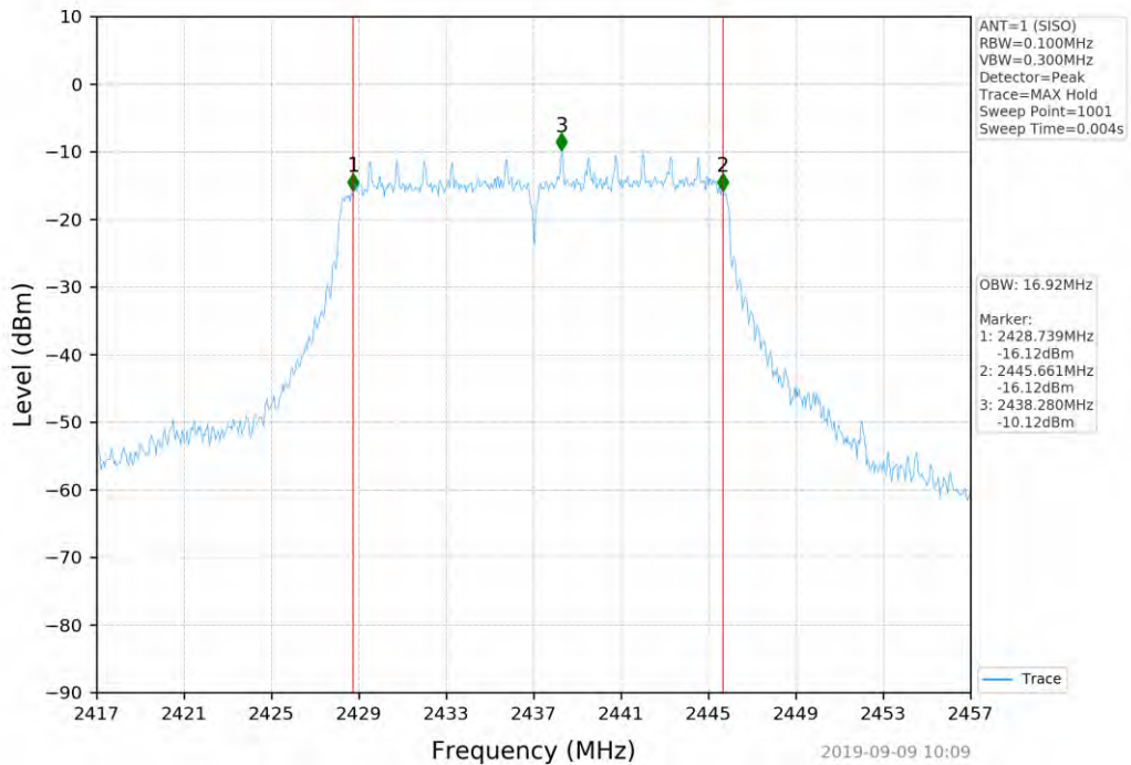
802.11n(HT20)_2437MHz_SISO_ANT1
