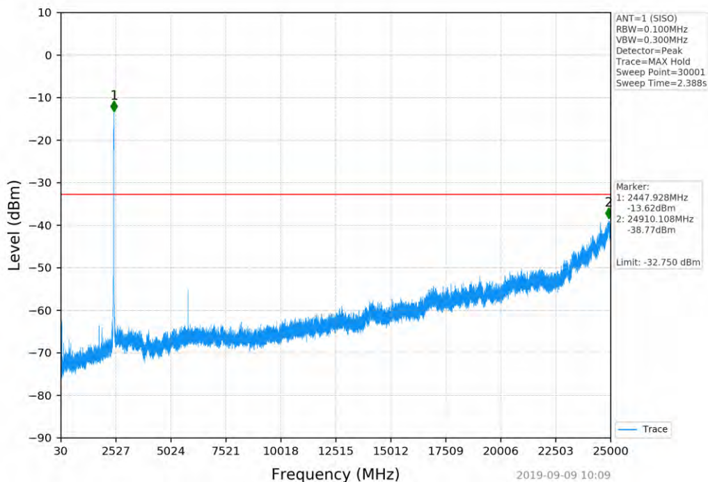
802.11n(HT40)_2437MHz_SISO_ANT1
