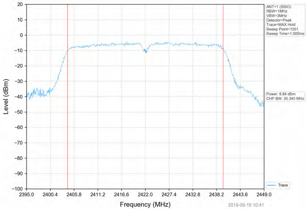
802.11n(HT40)_2422MHz_SISO_ANT1
