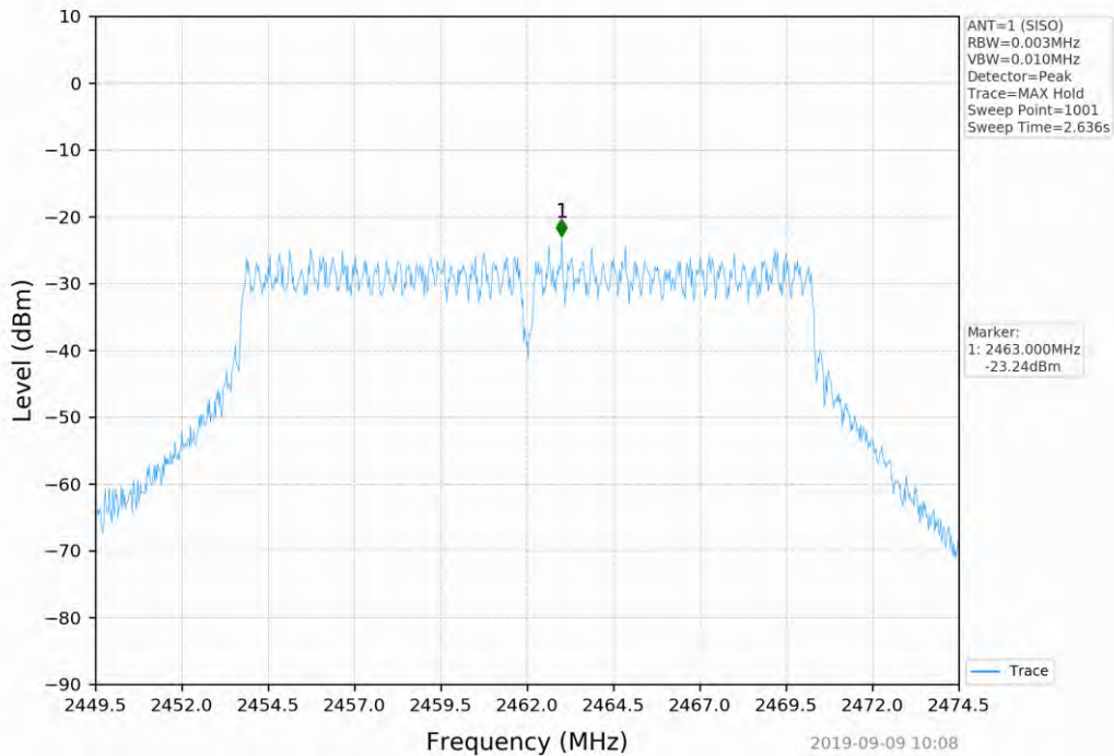
802.11g_2462MHz_SISO_ANT1
