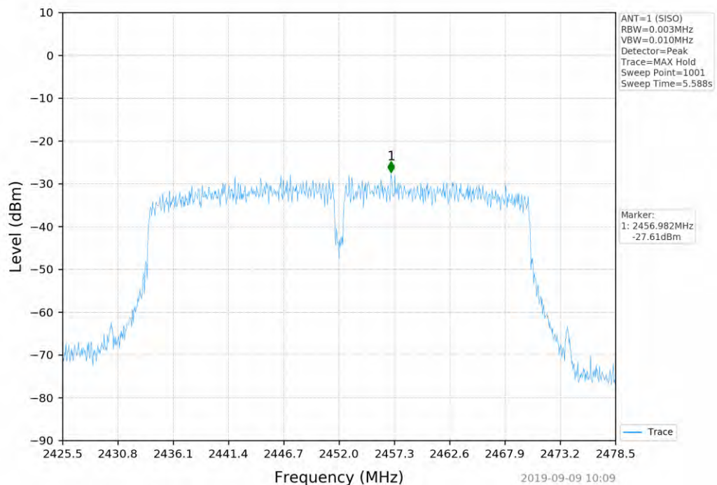
802.11n(HT40)_2452MHz_SISO_ANT1
