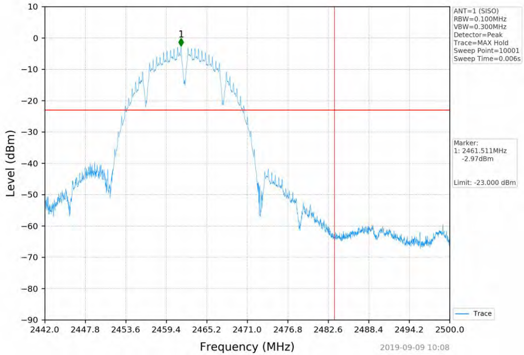
802.11b_2462MHz_SISO_ANT1
