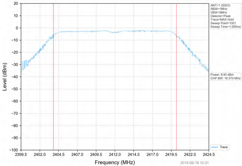
802.11g_2412MHz_SISO_ANT1
