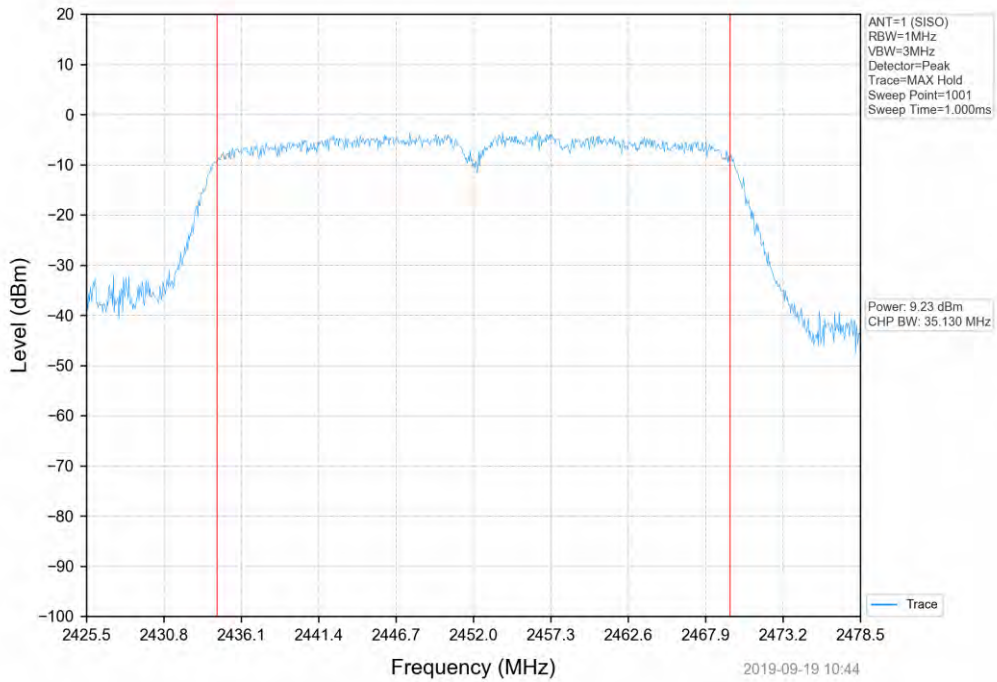
802.11n(HT40)_2452MHz_SISO_ANT1
