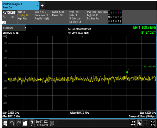
Band4-1.4MHz-QPSK-20175-1RB#0-Range2:1000~20000MHz
