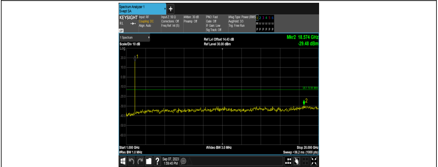
Band2-3MHz-16QAM-18615-1RB#0-Range2:1000~20000MHz
