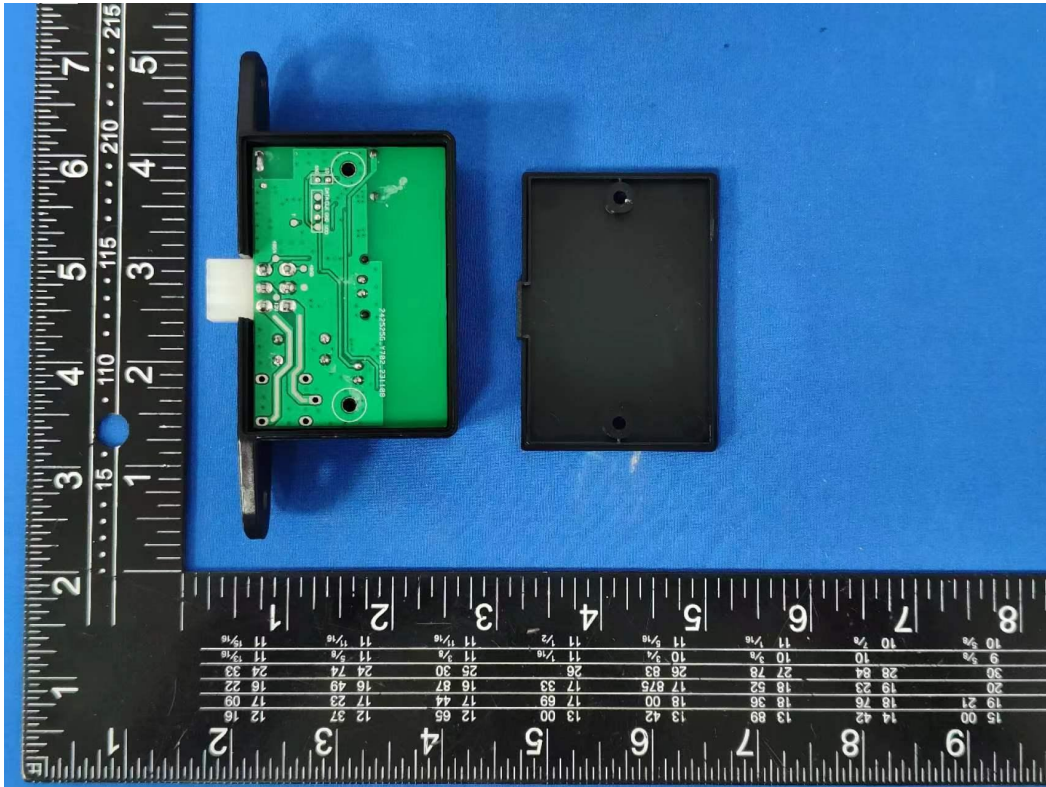
433 RX ANT
