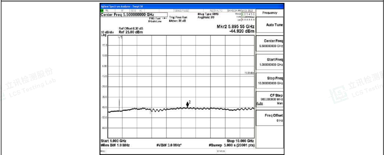
Band4-10MHz-QPSK-20000-1RB#0-Range5:10000~20000MHz
