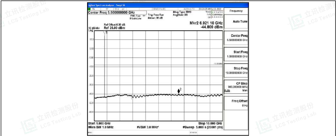
Band4-5MHz-QPSK-20175-1RB#0-Range5:10000~20000MHz
