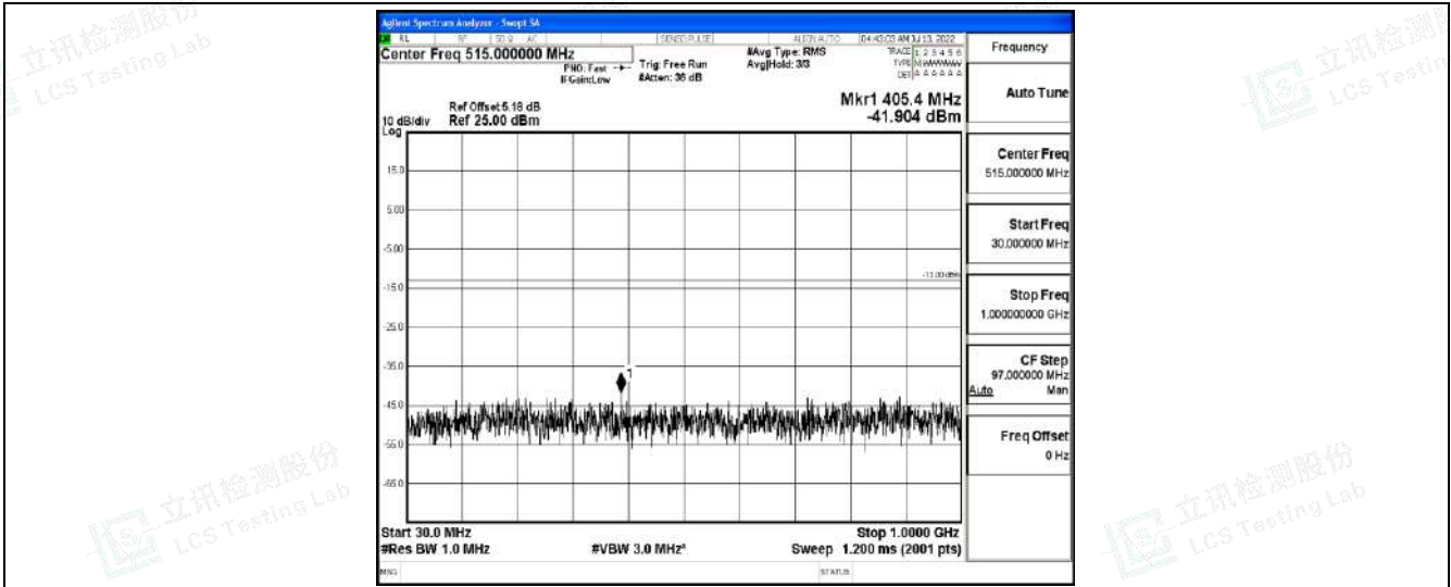
Band4-10MHz-QPSK-20000-1RB#0-Range4:1000~10000MHz
