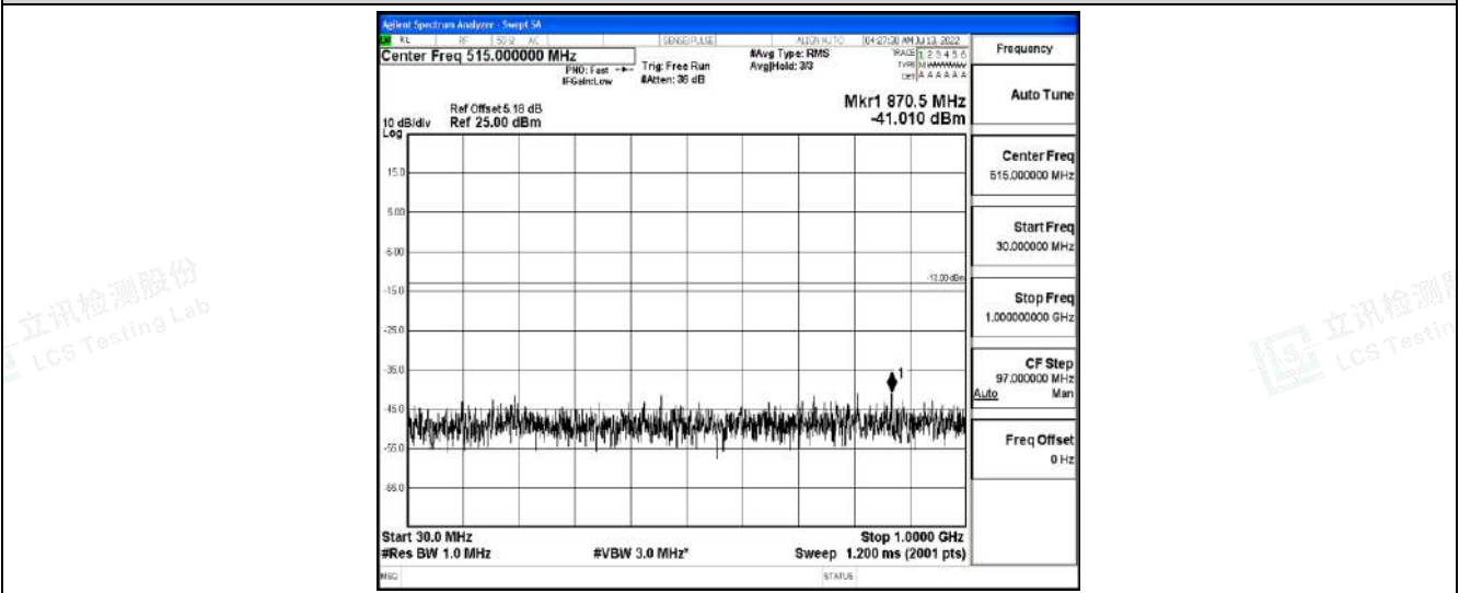
Band4-5MHz-QPSK-20375-1RB#0-Range4:1000~10000MHz
