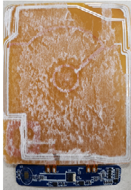
ANT Module(Back)
