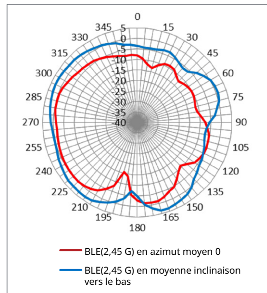
Plan d'élévation (vue de côté) - BLE
