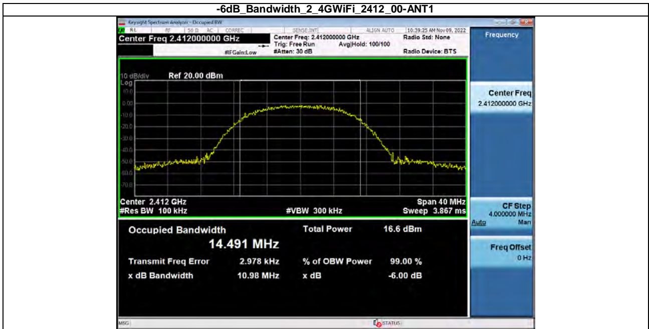
-6dB_Bandwidth_2_4WiFi_2412_00-ANT1
