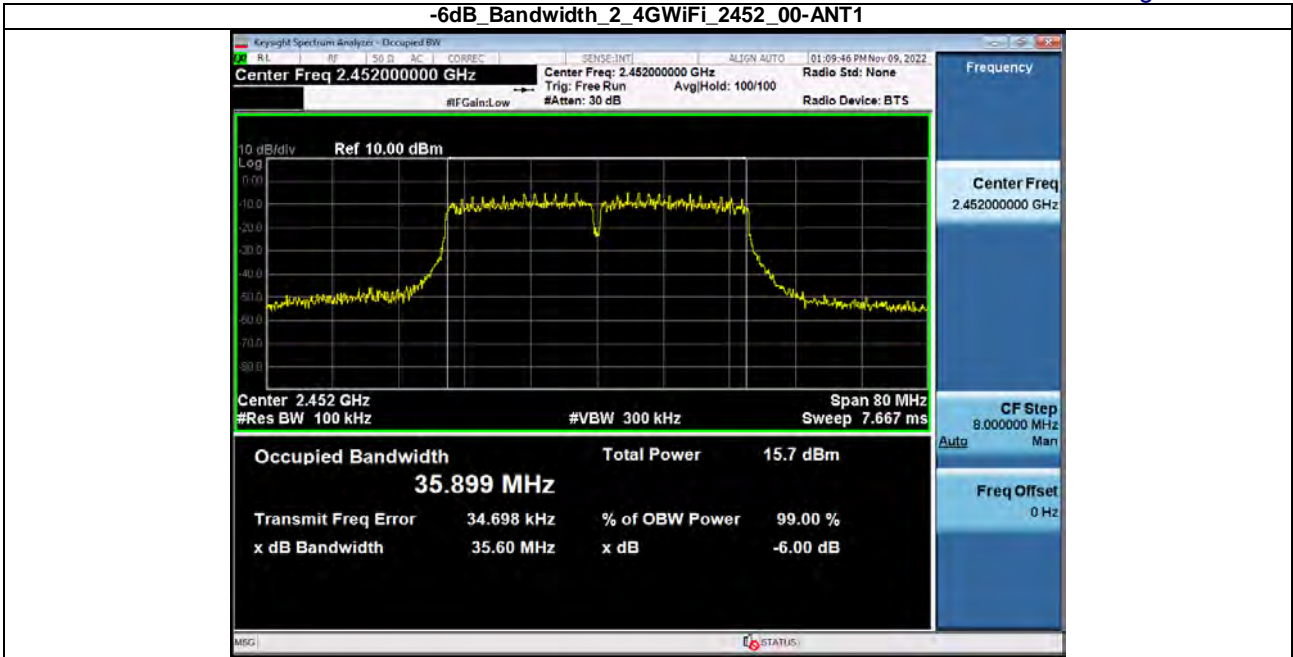
-6dB_Bandwidth_2_4WiFi_2452_00-ANT1
