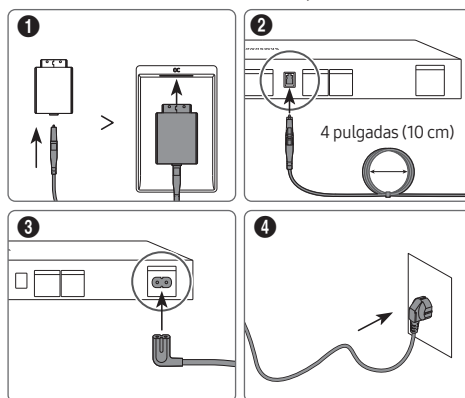
Caja de One Connect
