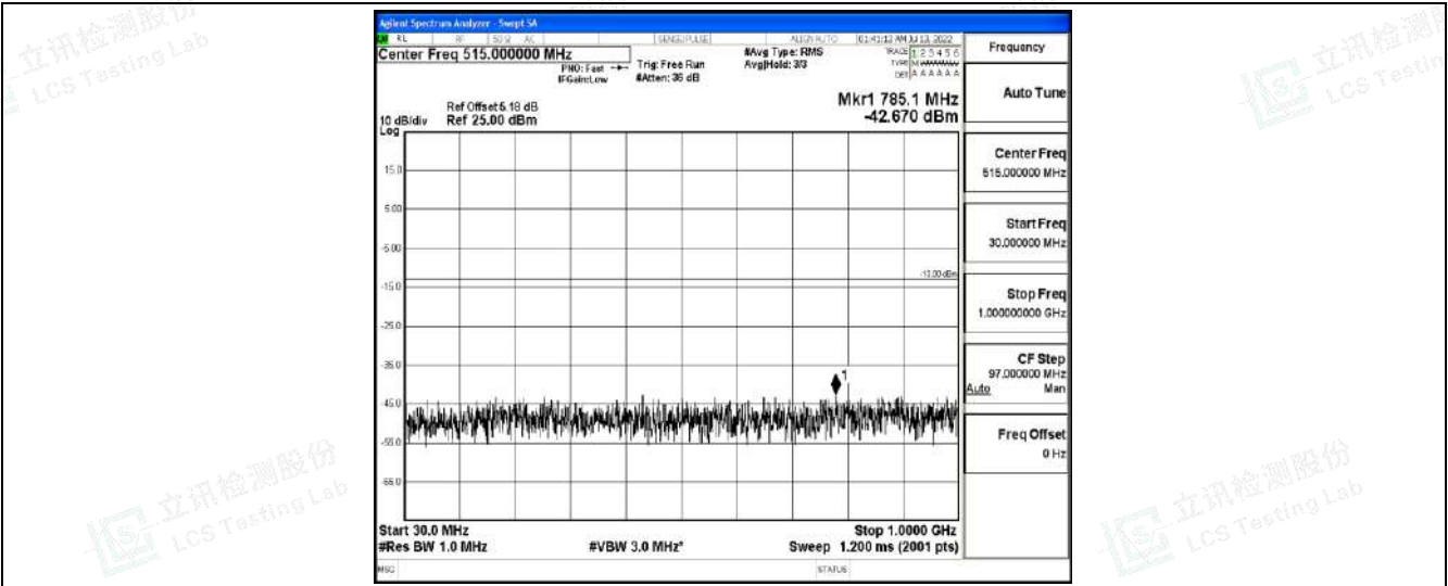
Band2-20MHz-QPSK-18700-1RB#0-Range4:1000~10000MHz
