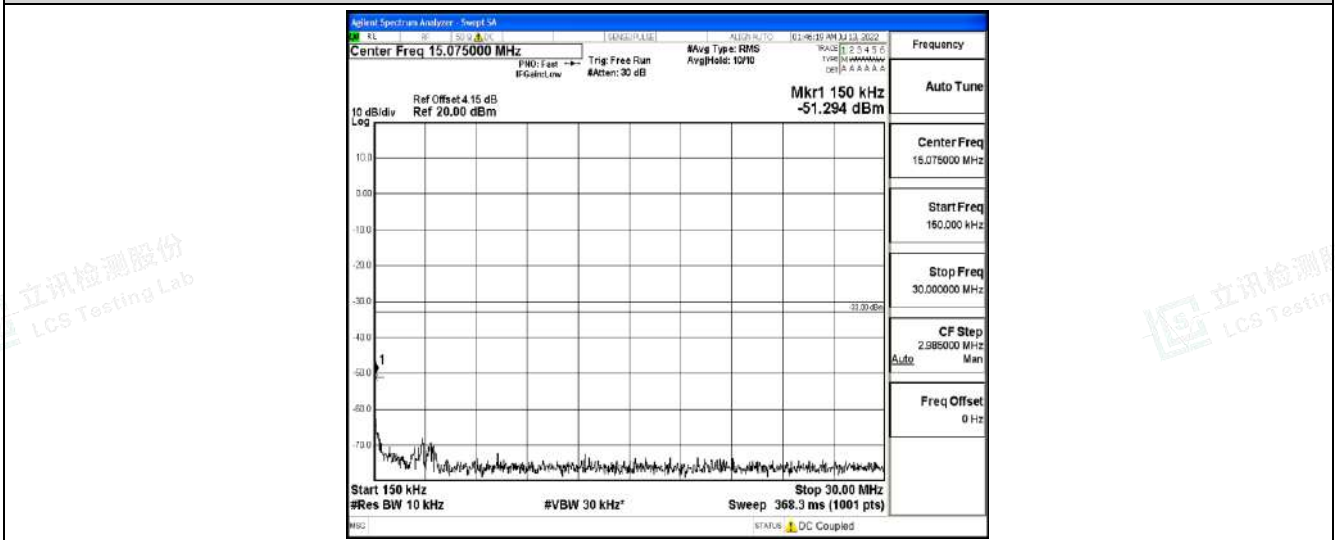
Band2-20MHz-16QAM-18900-1RB#0-Range3:30~1000MHz
