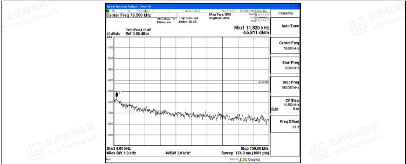
Band2-20MHz-16QAM-18900-1RB#0-Range2:0.15~30MHz
