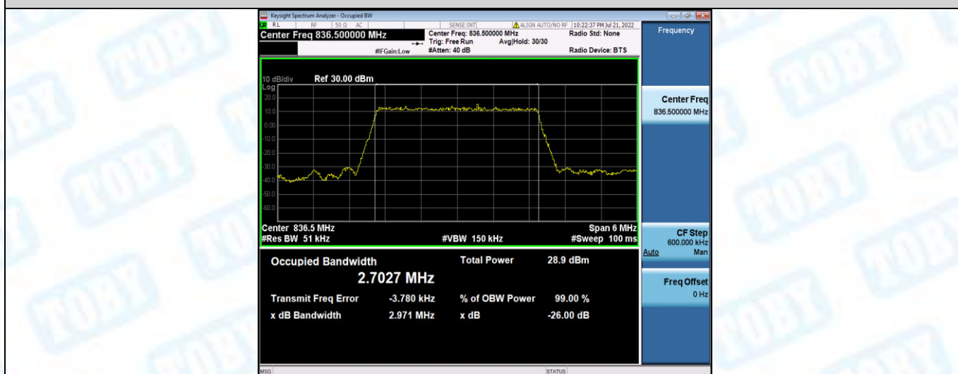
Band5-3MHz-QPSK-20635-15RB#0
