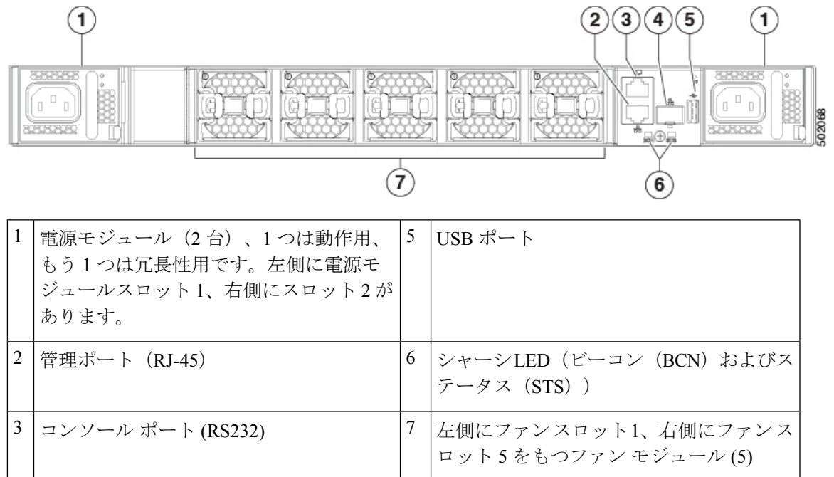
図 2: Cisco Nexus 9332C スイッチの電源側面図
