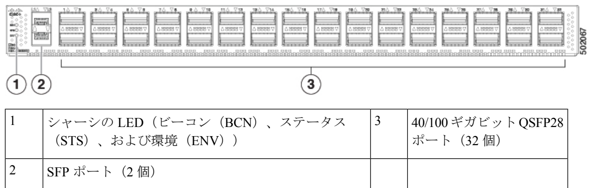
図 1: Cisco Nexus 9332C スイッチのポート側面図
