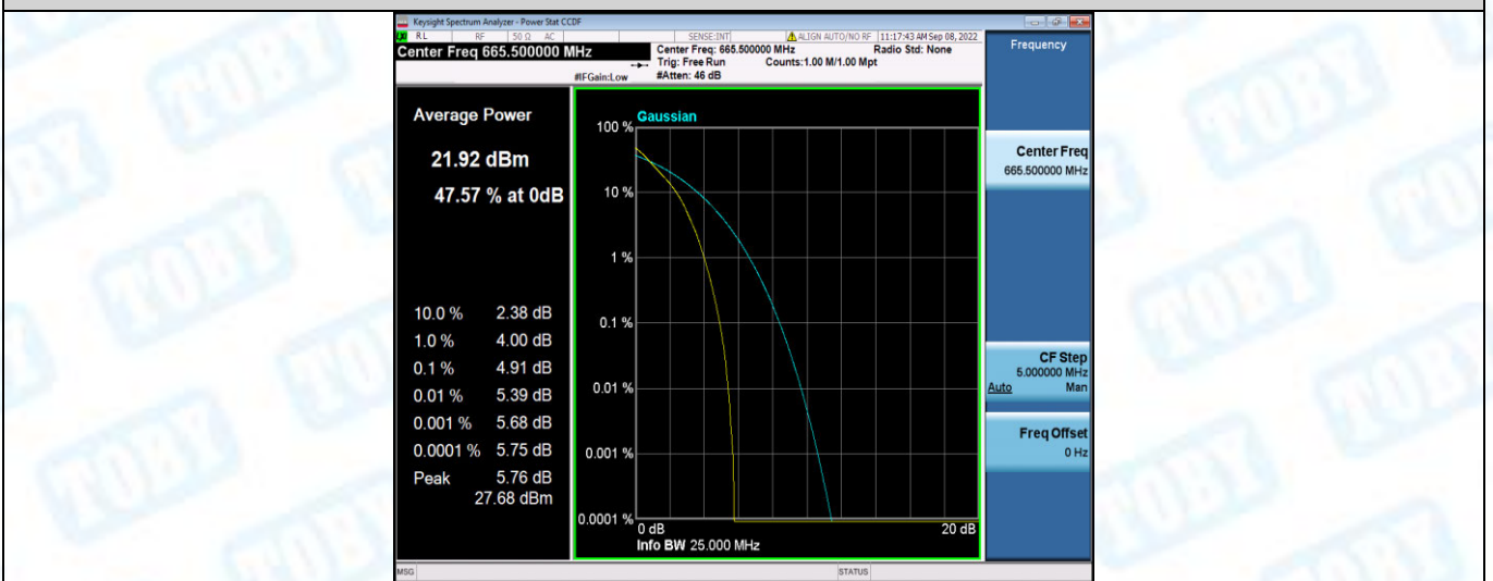
Band71-5MHz-QPSK-133297-1RB#0
