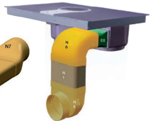
Luftudtag bagud
