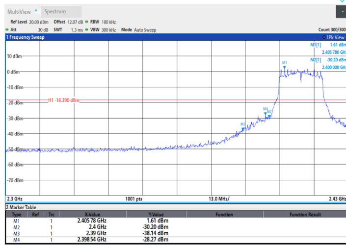
11G_Ant1_Low_2412
