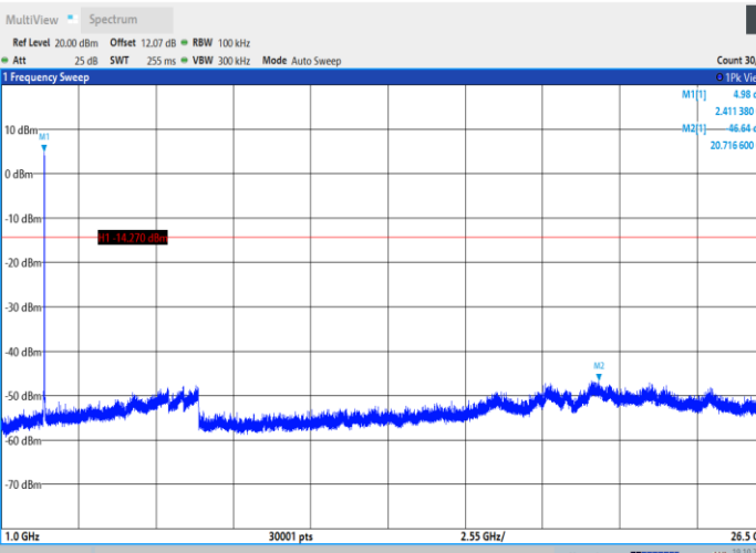
11B_Ant1_2412_1000~26500
