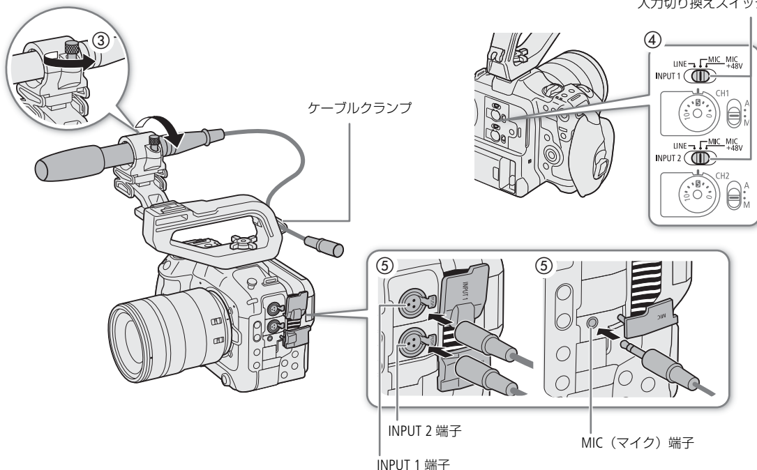
INPUT 1 / INPUT 2端子 入力切り換えスイッチ
