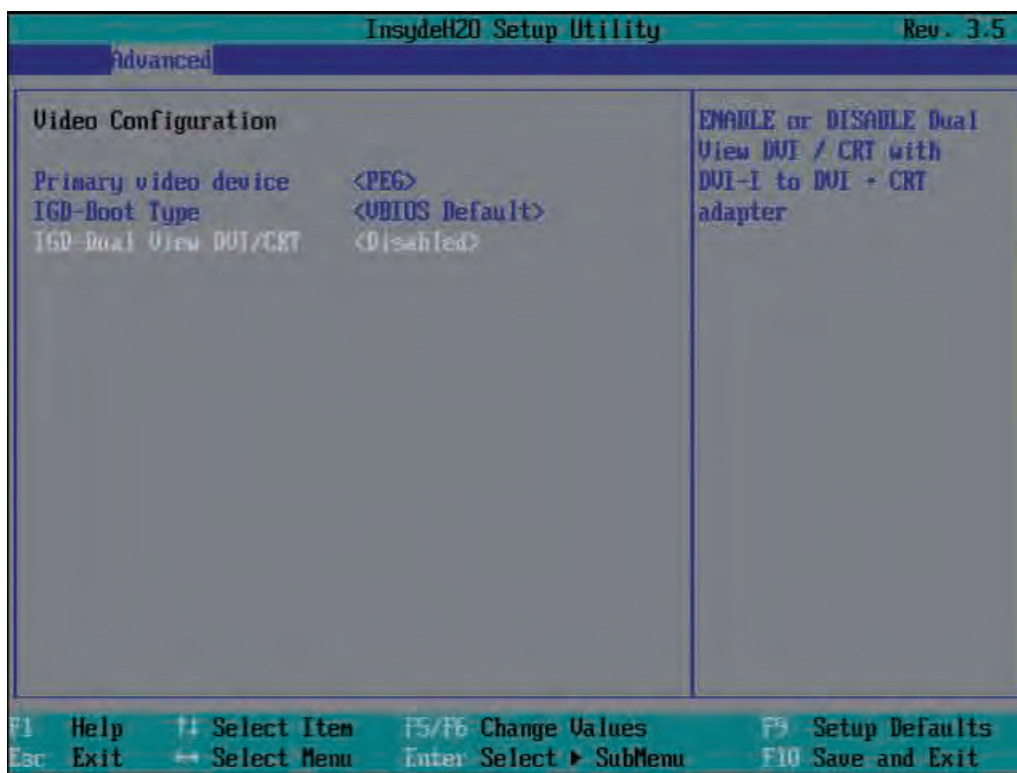
図 16-5 サブメニュー[Advanced]メニュー > [Video Configuration]
