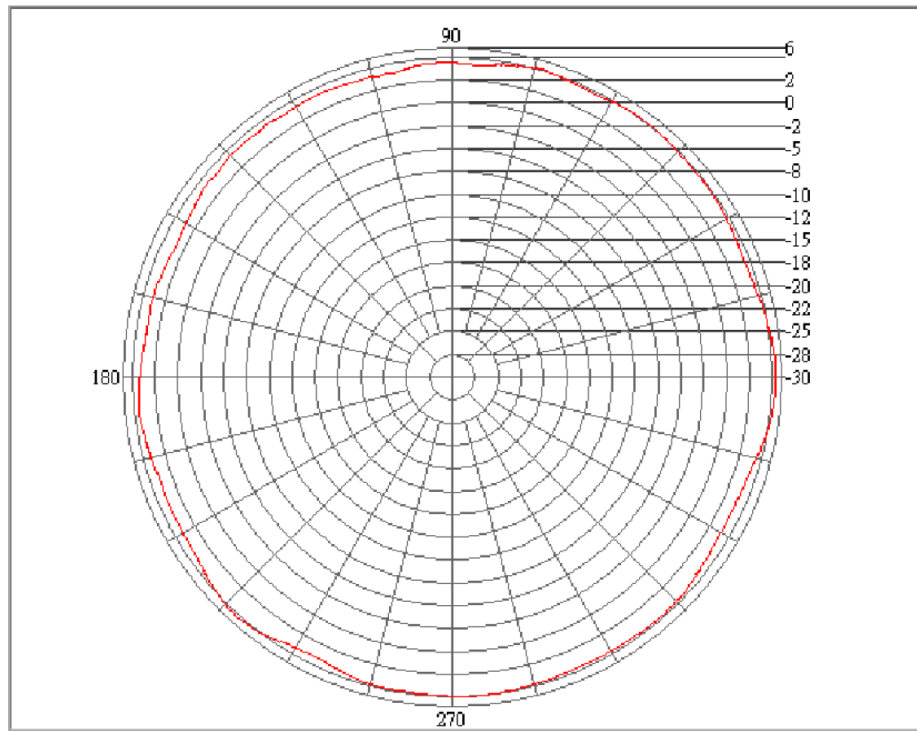
H-Plane 900mhz
