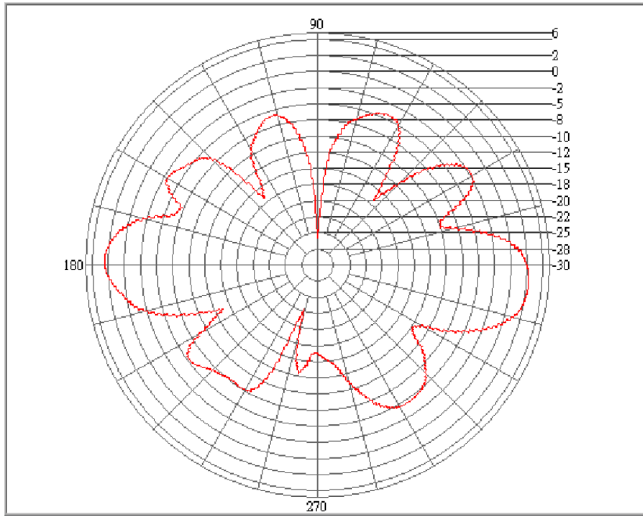
E-Plane 900mhz
