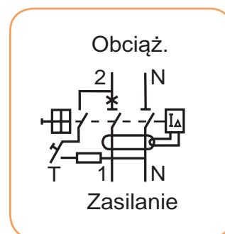
Układ połączeń wewnętrznych
