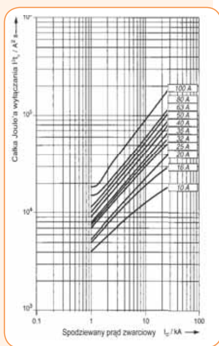
Charakterystyka I 2 t wyłączników selektywnych ETIMAT S
