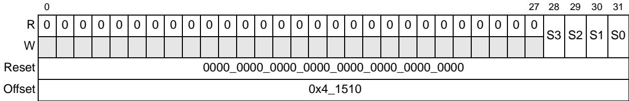
Figure 10-24. Message Status Register (MSR)
