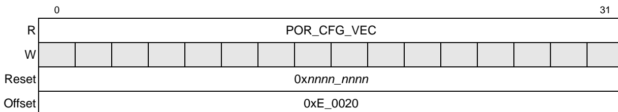
Figure 17-6. POR Configuration Register (GPPORCR)
