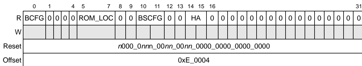
Figure 17-2. POR Boot Mode Status Register (PORBMSR)
