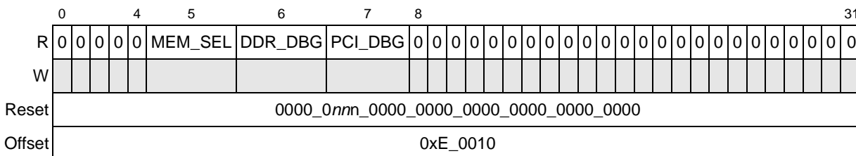
Figure 17-5. POR Debug Mode Status Register (PORDBGMSR)
