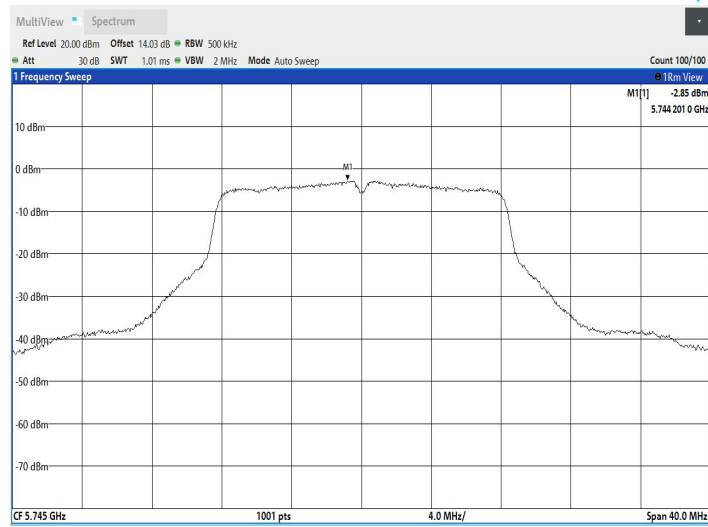
11A_Ant2_5745
