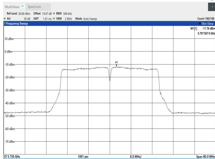
11N40SISO_Ant2_5755
