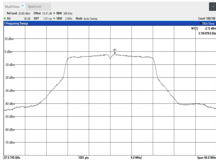
11N20MIMO_Ant1_5785
