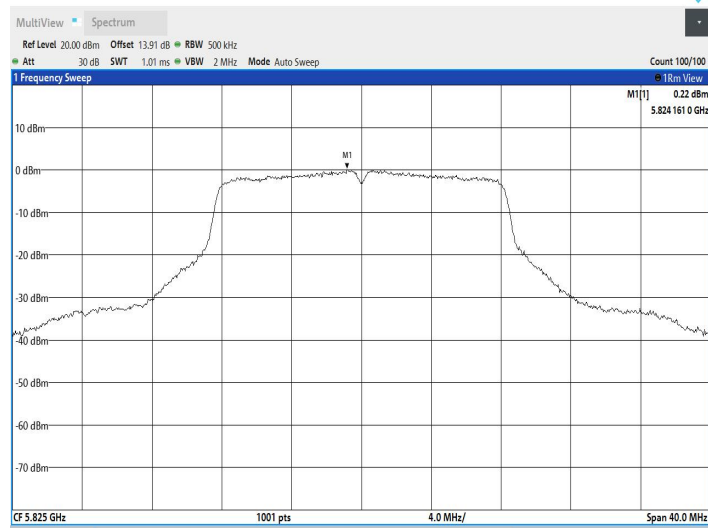
11A_Ant2_5825
