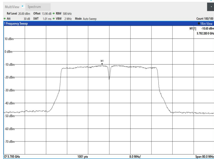
11AC40SISO_Ant2_5795
