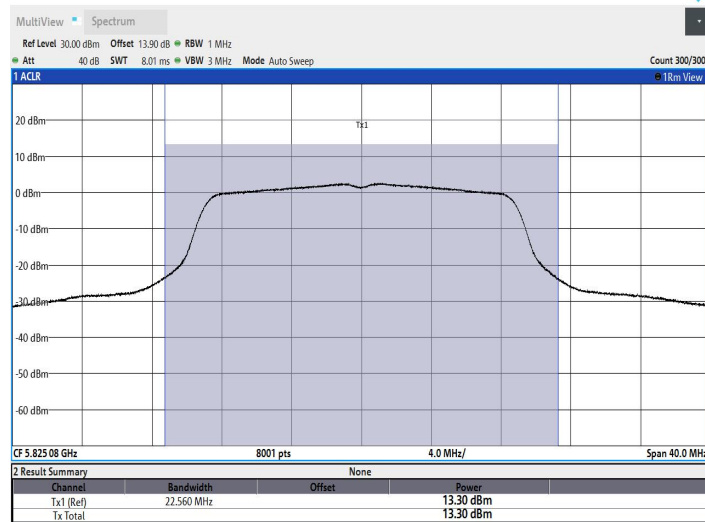
11N20MIMO_Ant2_5825
