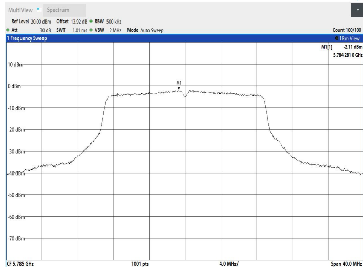
11N20SISO_Ant2_5785
