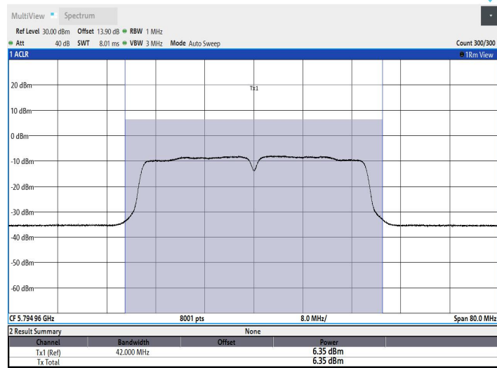
11N40MIMO_Ant2_5795
