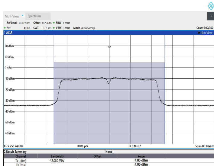
11AC40MIMO_Ant1_5795
