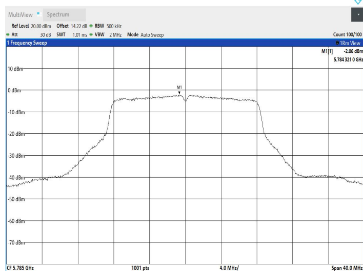
11A_Ant1_5825
