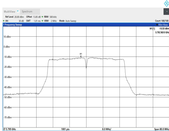
11N40SISO_Ant2_5795
