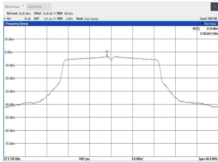
11N20SISO_Ant2_5745
