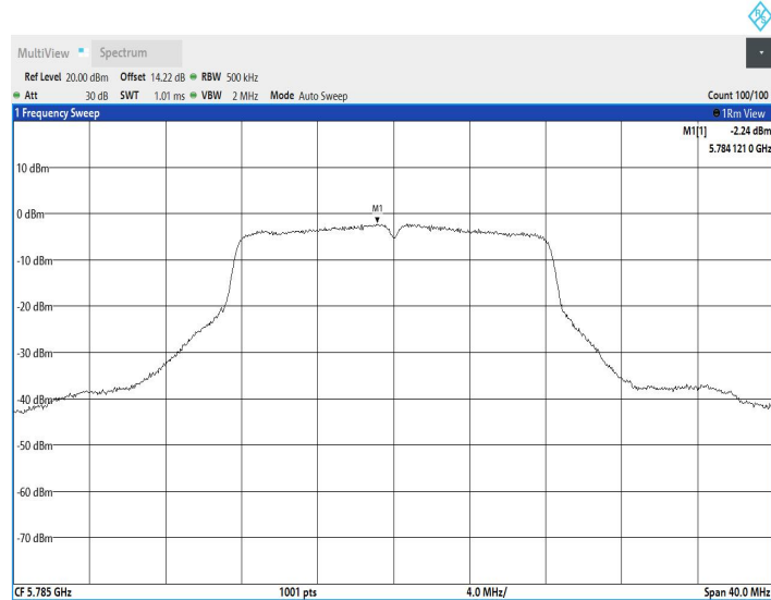
11A-CDD_Ant1_5825
