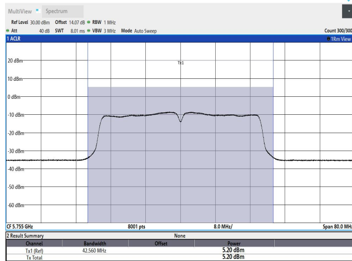
11N40MIMO_Ant2_5755
