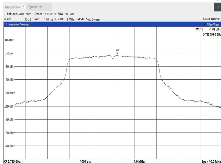
11A_Ant2_5785
