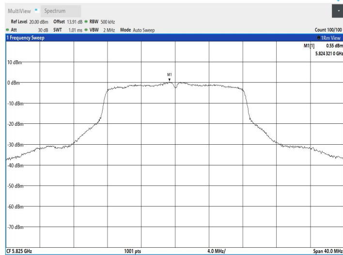
11A-CDD_Ant2_5825
