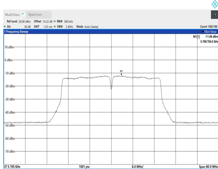
11AC80SISO_Ant1_5775
