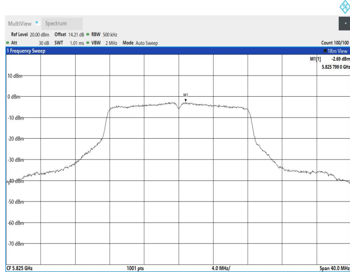
11N20MIMO_Ant1_5745
