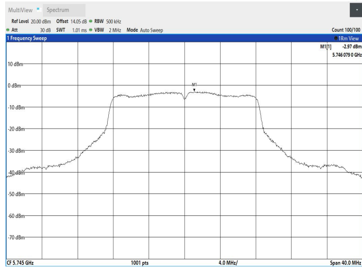
11A-CDD_Ant2_5745
