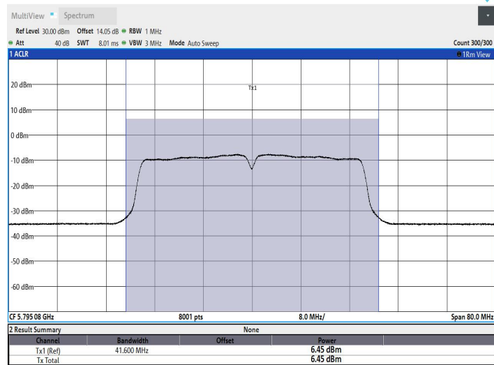
11AC40MIMO_Ant2_5795
