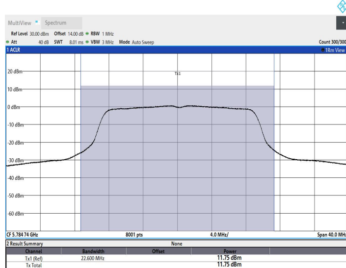
11AC20MIMO_Ant2_5785
