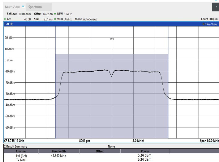
11AC40MIMO_Ant2_5755
