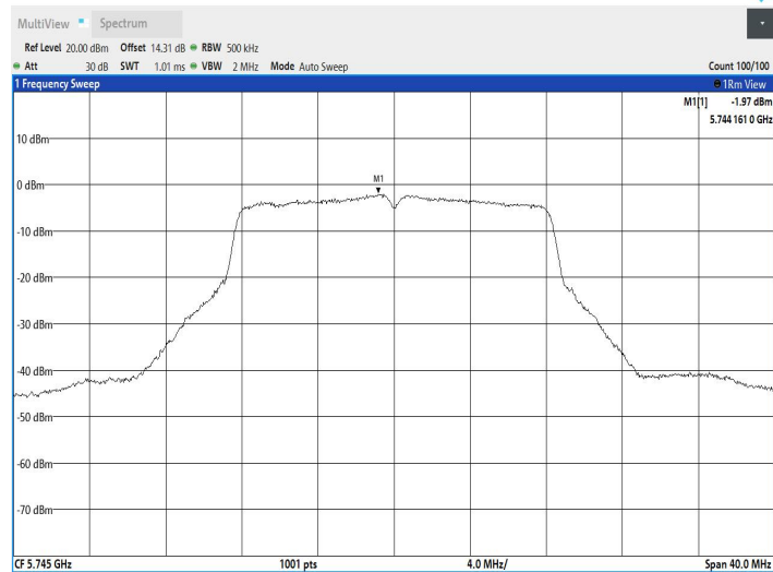
11A-CDD_Ant1_5785
