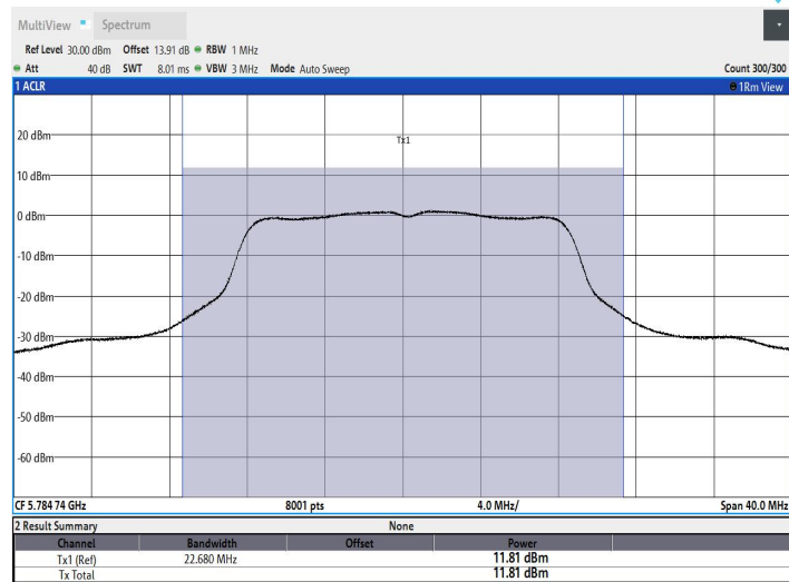
11N20MIMO_Ant2_5785
