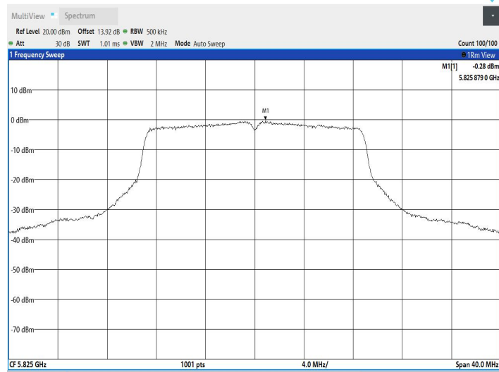
11N20SISO_Ant2_5825
