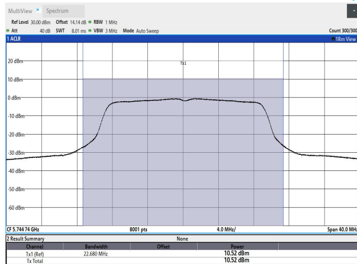
11AC20MIMO_Ant2_5745
