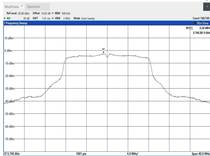
11N20MIMO_Ant2_5745
