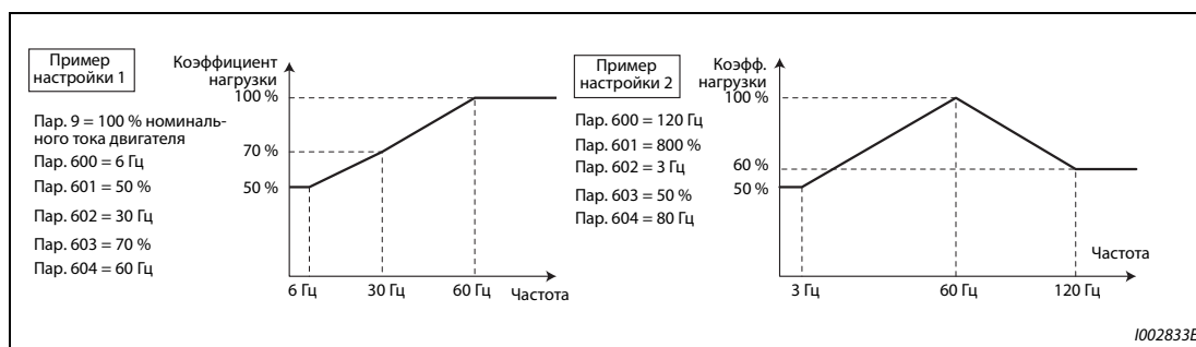
Рис. 5-55: Примеры настройки
