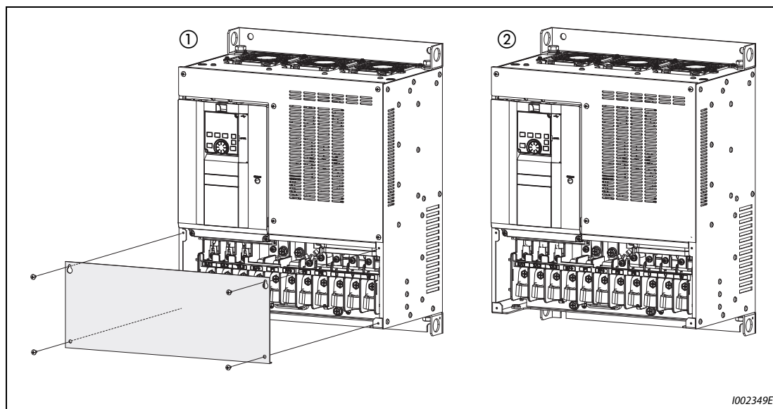
Рис. 2-10: Снятие нижней передней панели
