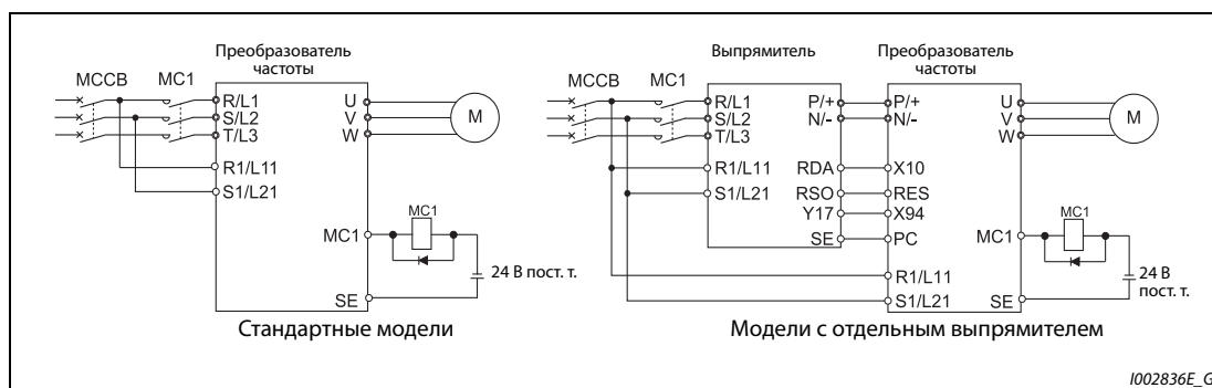
Рис. 5-151: Электроснабжение через клеммы R1 и S1
