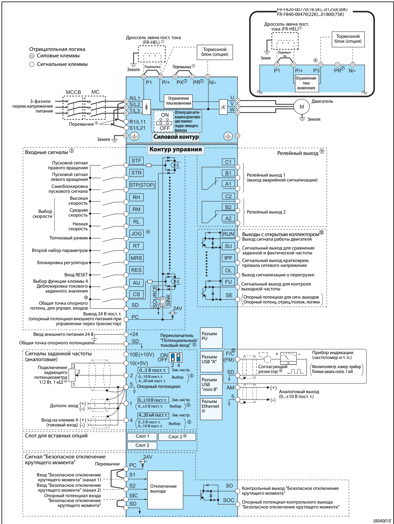
Рис. 2-22: Схема подключения преобразователя частоты (тип FM) (FR-F800-E)
