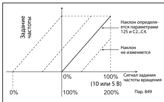
Рис. 5-123: Настройка смещения
