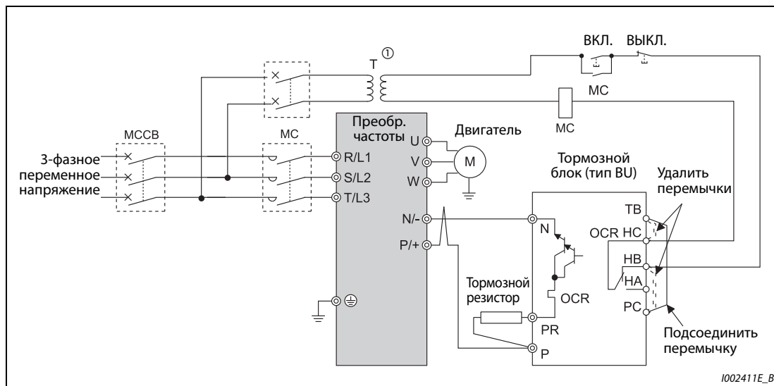
Рис. 2-52: Подключение тормозного блока типа ВU
