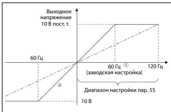
Рис. 5-83: Опорная величина для выхода AM
