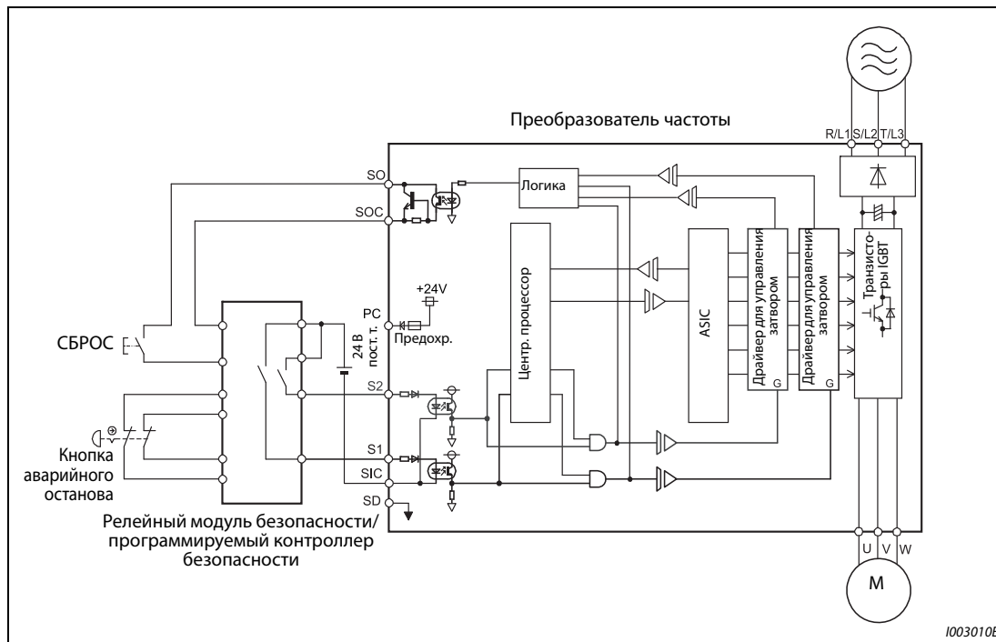
Рис. 2-44: Подключение релейного модуля безопасности
