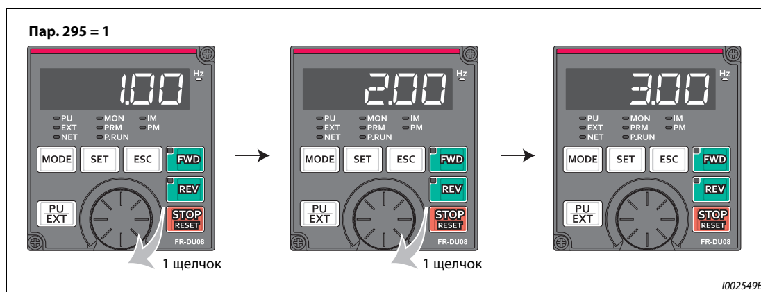
Рис. 5-9: Дискретность задания при настройке параметра 295 на "1,00"
