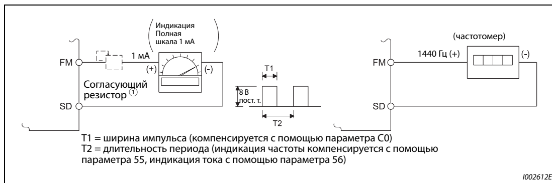
Рис. 5-85: Калибровка выхода FM
