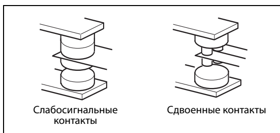
Рис. 2-37: Виды контактов
