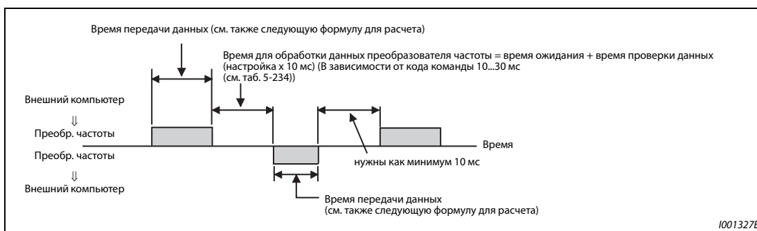
Рис. 5-238: Время передачи
