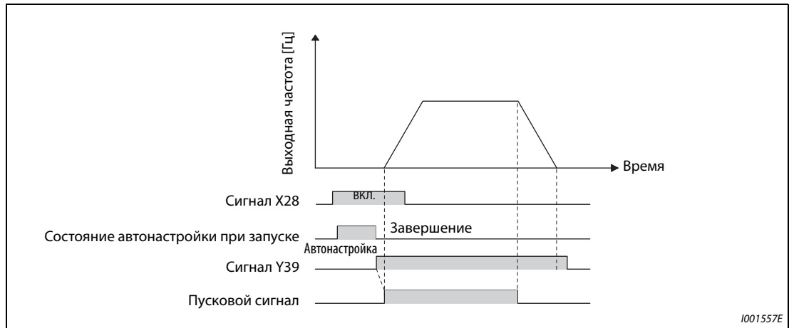
Рис. 5-143: Запуск онлайн-автонстройки параметров двигателя по внешнему сигналу
