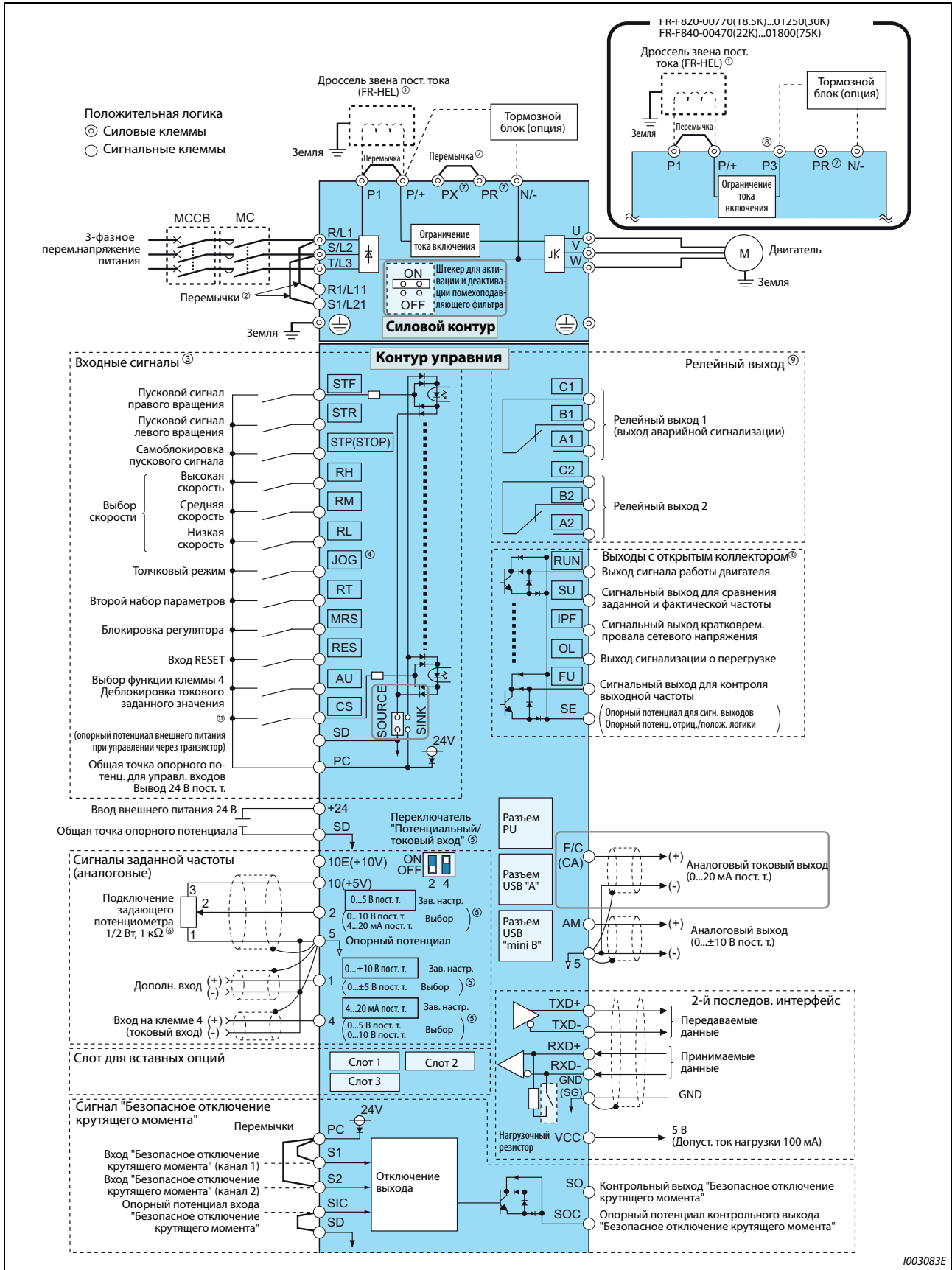
Рис. 2-19: Схема подключения преобразователя частоты (тип СА)
