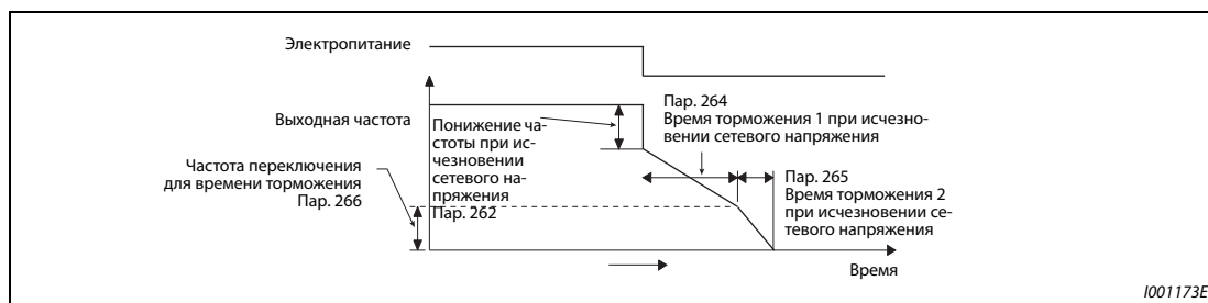
Рис. 5-214: Параметры метода останова при исчезновении сетевого напряжения
