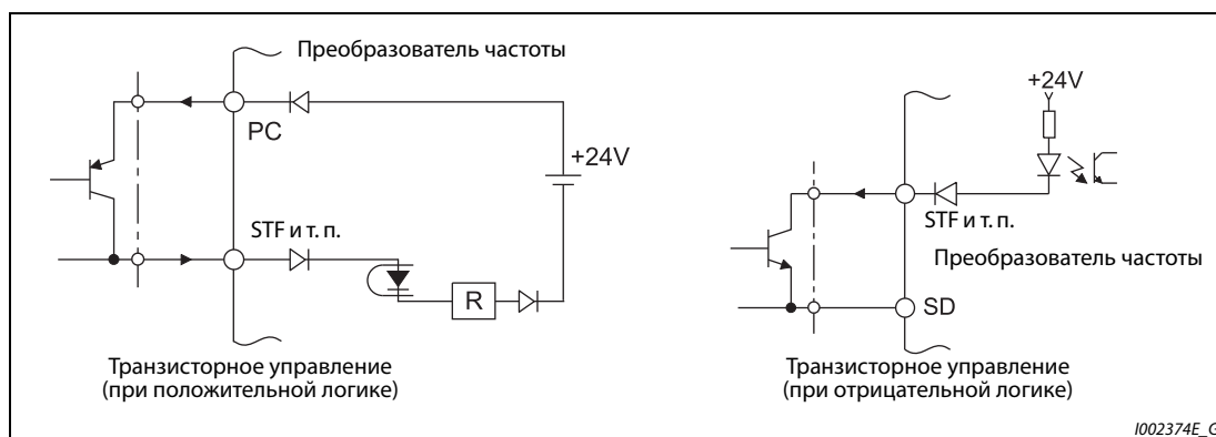
Рис. 2-36: Управление входами через транзисторы
