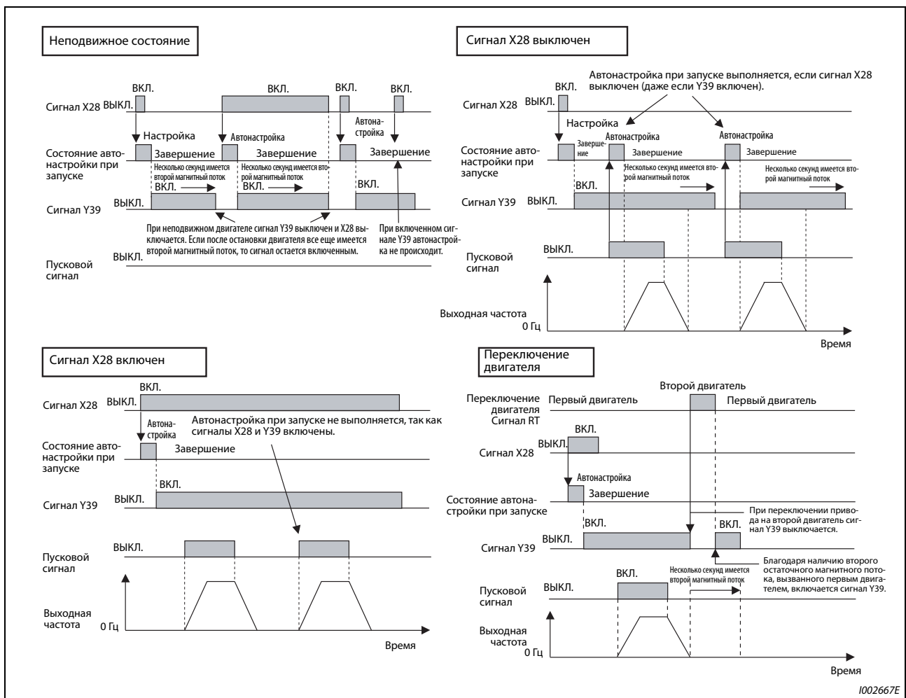
Рис. 5-144: Временные диаграммы онлайн-автонстройки параметров двигателя
