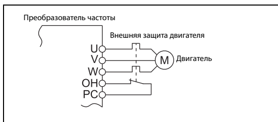
Рис. 5-50: Подключение внешней защиты двигателя
