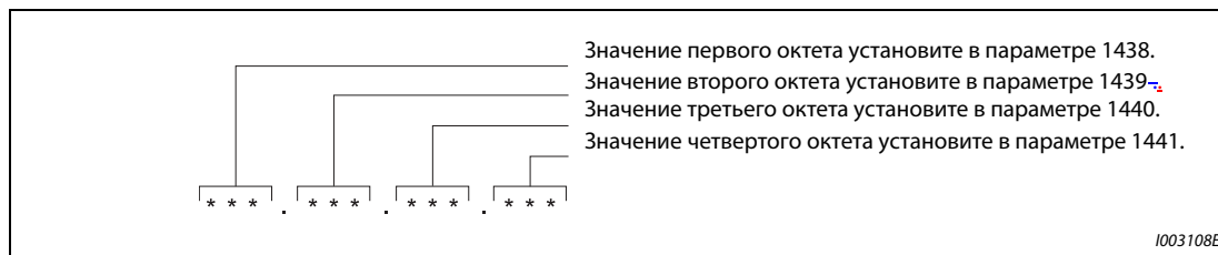
Рис. 5-249: Настройка маски подсети
