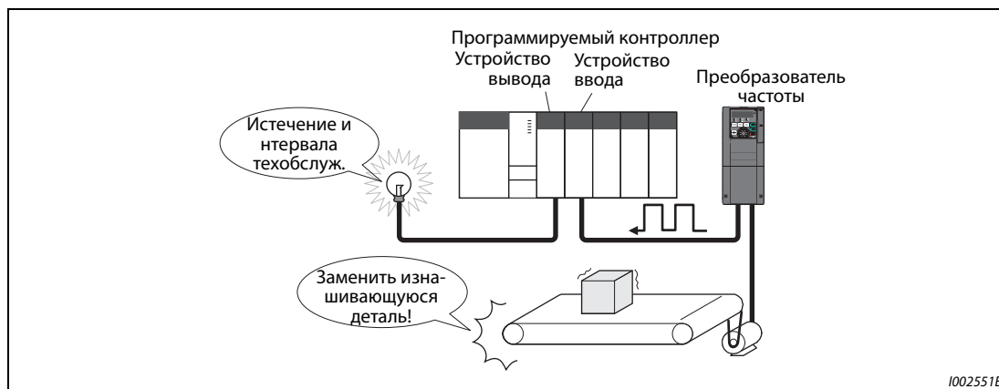
Рис. 5-12: Контроль интервала техобслуживания и среднего значения тока
