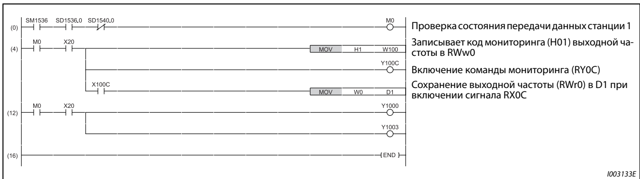
Рис. 5-293: Пример программы 4
