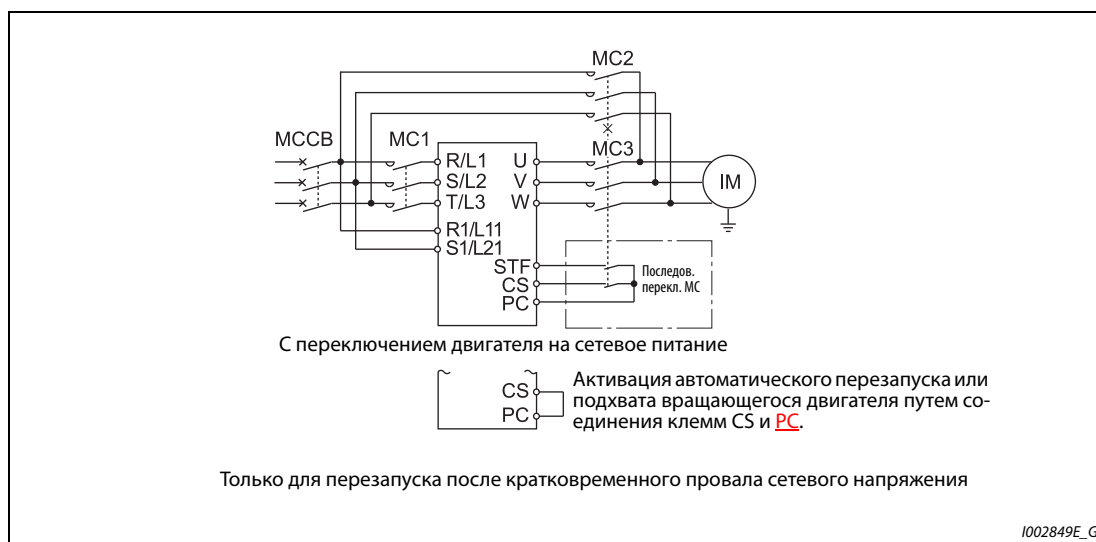
Рис. 5-205: Пример подключения
