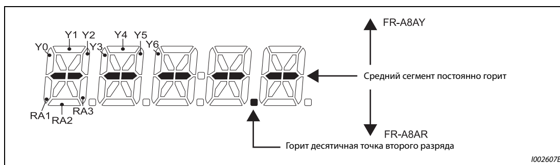
Рис. 5-80: Индикация при установленной опции FR-A8AY или FR-A8AR
