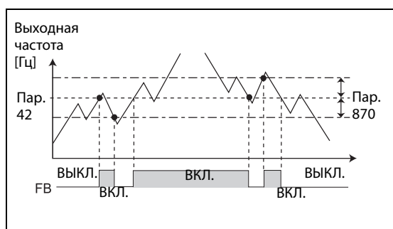
Рис. 5-99: Пример для вывода сигнала FB
