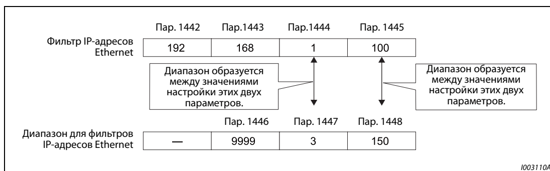
Рис. 5-251: Пример 1 настройки для фильтрации IP-адресов Ethernet
