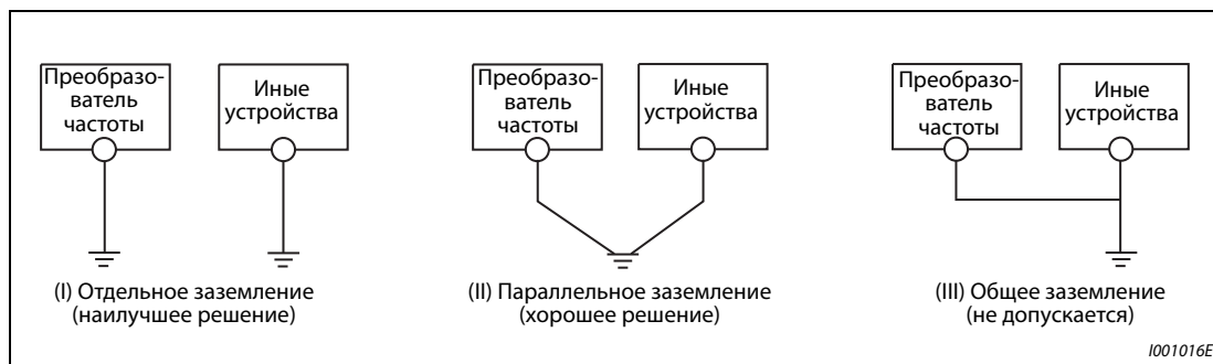
Рис. 2-25: Заземление системы привода
