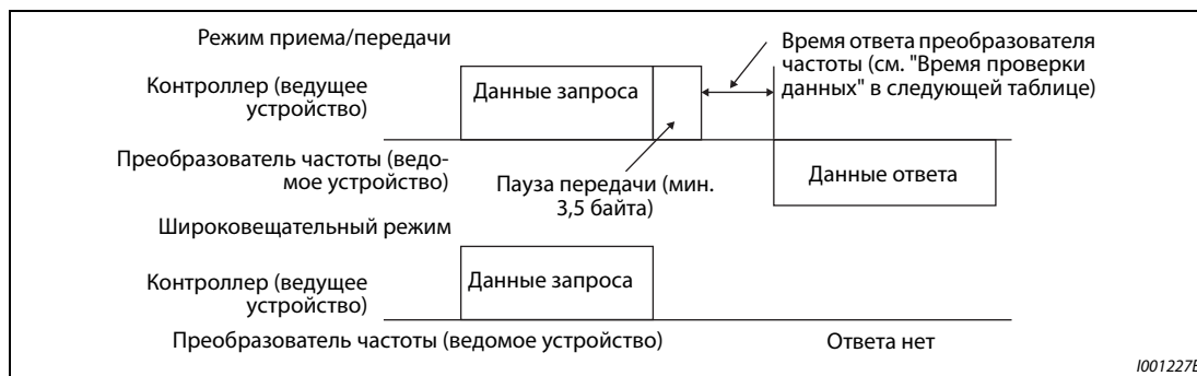
Рис. 5-242: Формат сообщений
