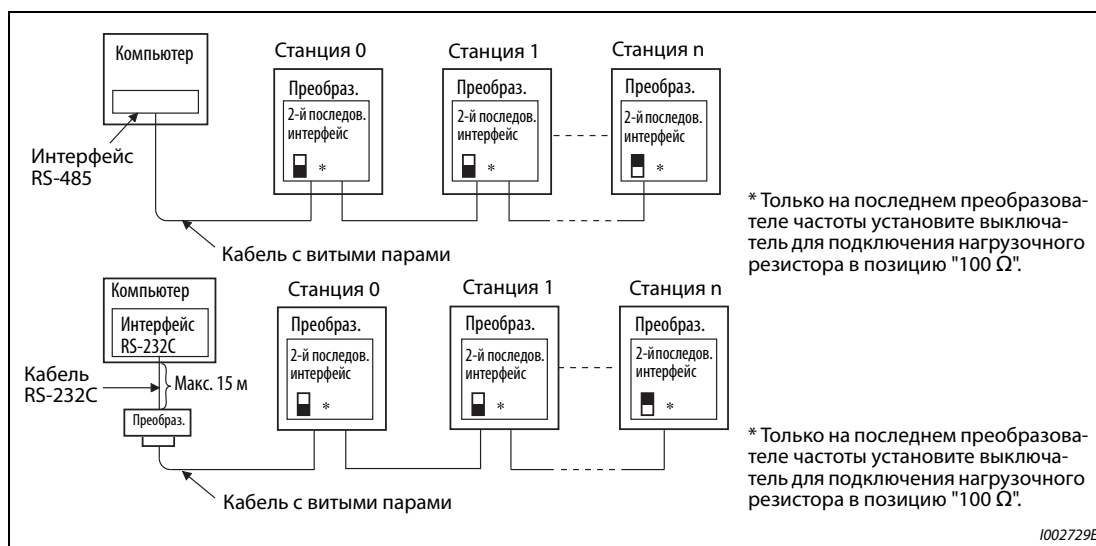
Рис. 5-227: Соединение с несколькими преобразователями частоты
