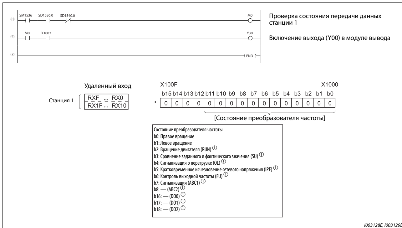
Рис. 5-290: Пример программы 1
