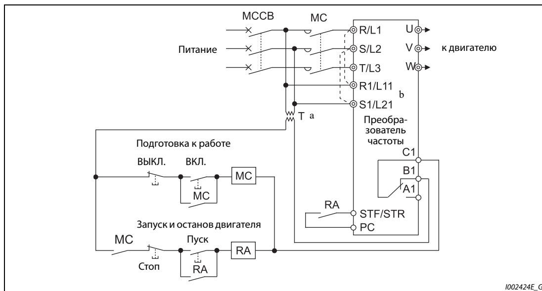
Рис. 3-12: Запуск/останов преобразователя частоты
