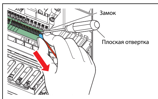
Рис. 2-35: Удаление провода
