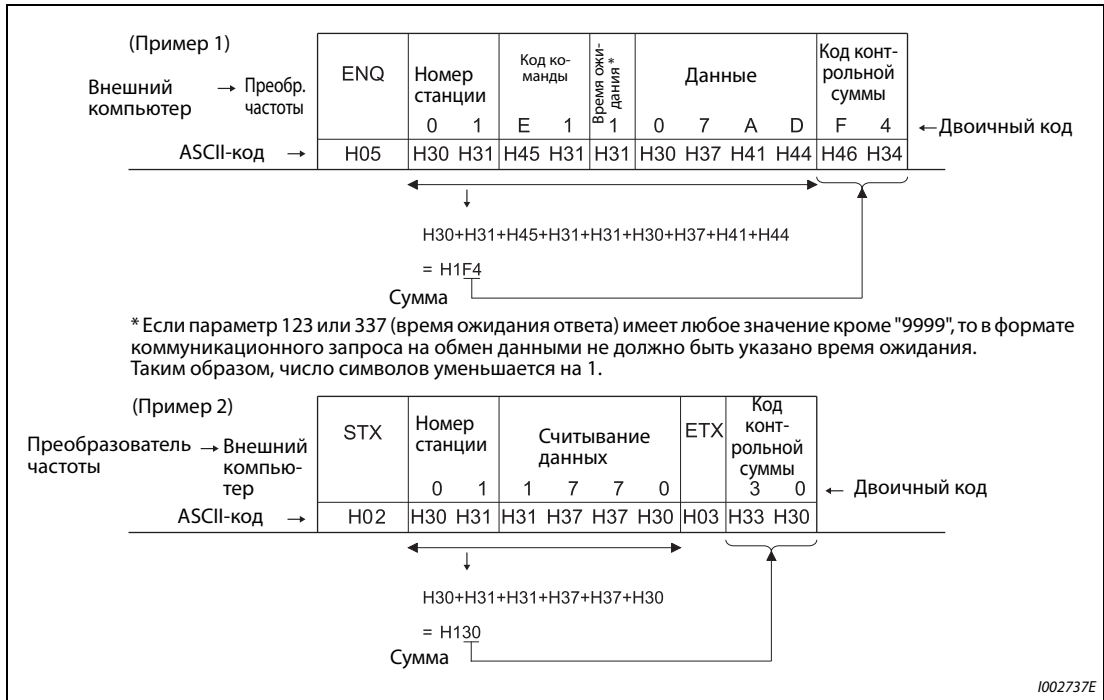
Рис. 5-237: Код контрольной суммы (примеры)
