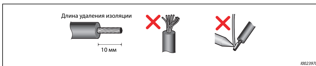
Рис. 2-31: Подготовка провода
