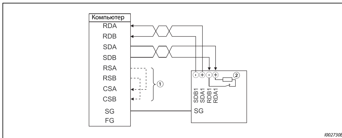
Рис. 5-228: Соединение с одним преобразователем частоты
