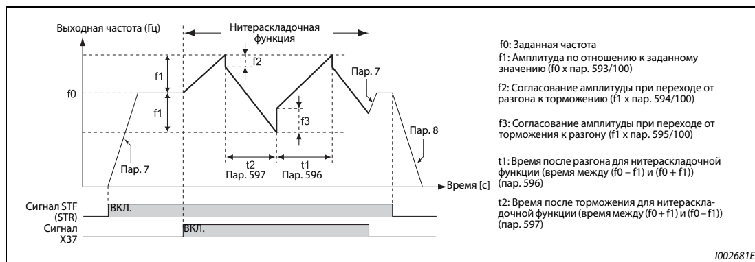
Рис. 5-154: Нитераскладочная функция
