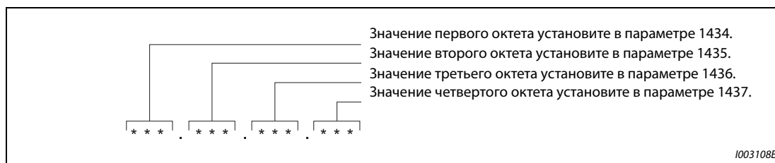
Рис. 5-248: Настройка IP-адреса
