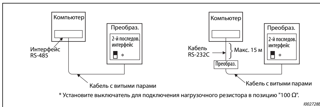
Рис. 5-226: Соединение с одним преобразователем частоты
