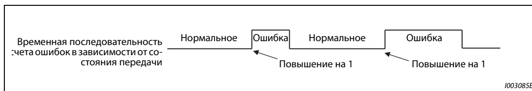
Рис. 5-234: Счет ошибок коммуникации
