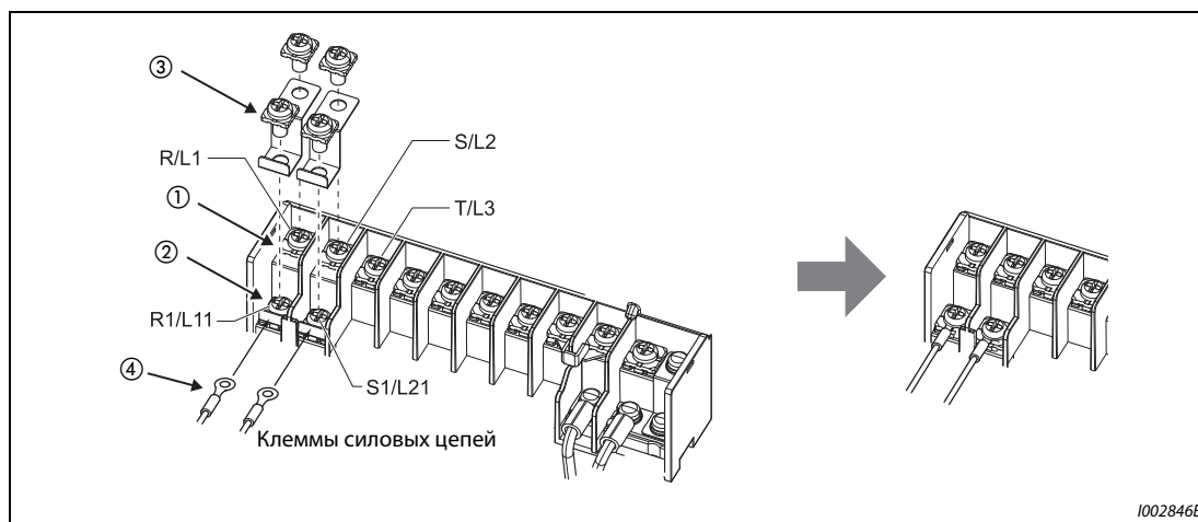
Рис. 2-40: Детальный вид клемм
