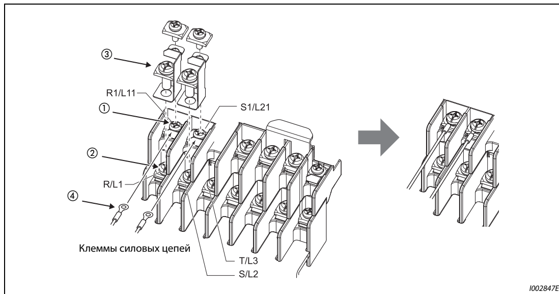
Рис. 2-41: Детальный вид клемм
