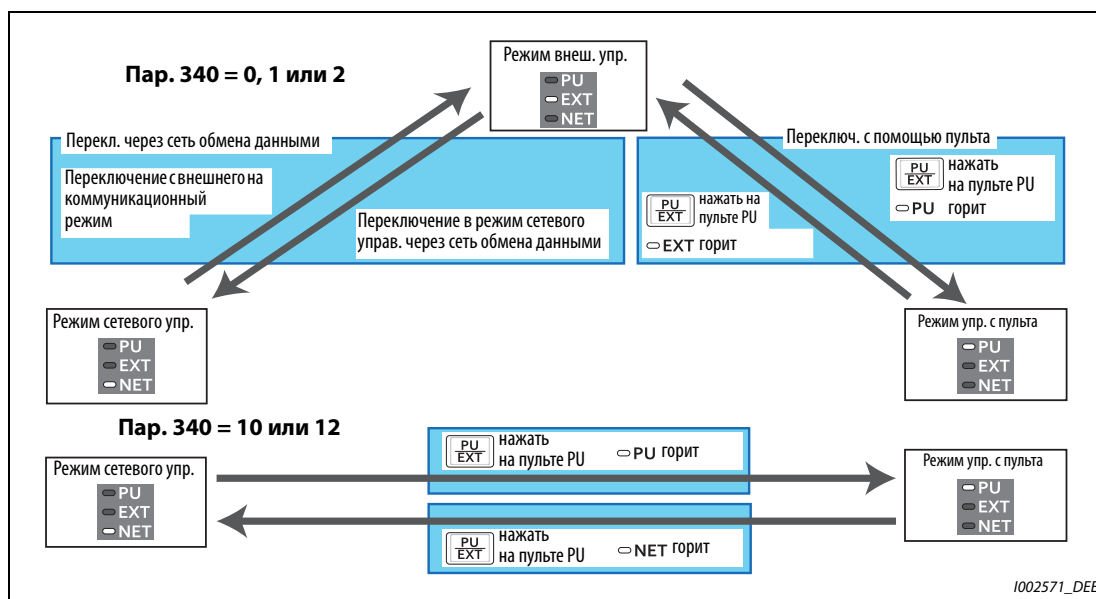
Рис. 5-32: Переключение режима
