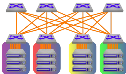
アリストアのボックス型システムのリーフ/スパイン構成。10GbE/25GbE 6,144 ポート、または 40GbE/100GbE 1,536 ポートまで拡張可能 (3:1 のオーバーサブスクリプション)
