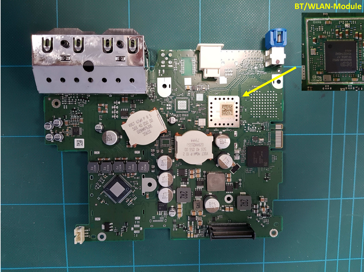
PCBA 4110 MAIN MMB 12GB D11 M303
