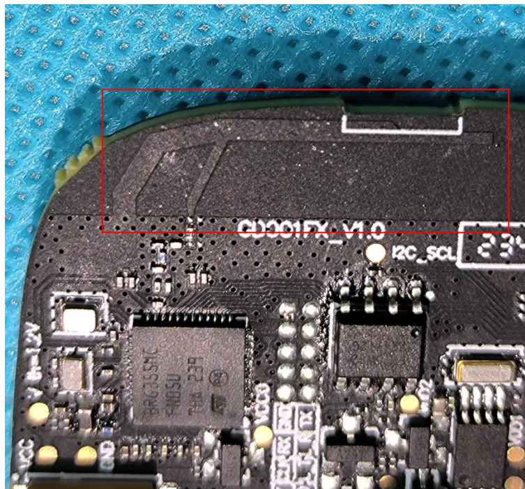
BLE ANT
