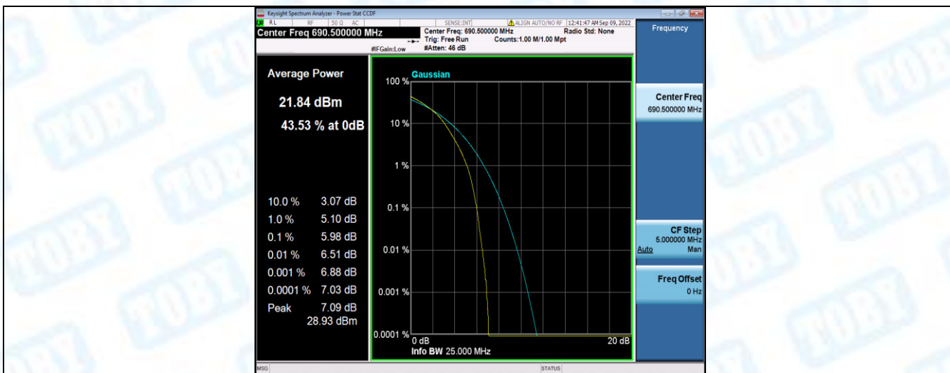
Band71-20MHz-QPSK-133222-1RB#0
