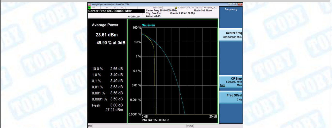
Band71-10MHz-QPSK-133422-50RB#0
