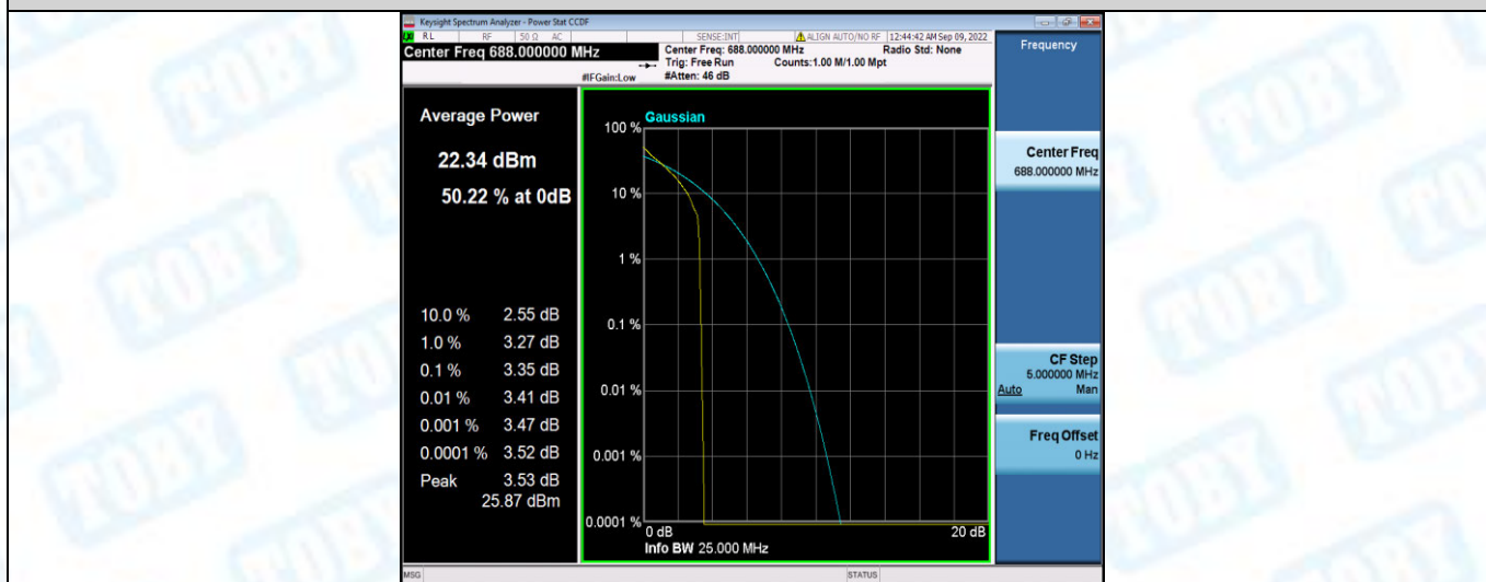
Band71-20MHz-QPSK-133372-100RB#0
