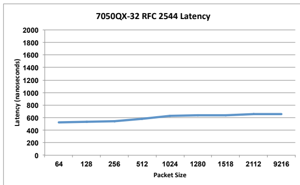
Arista 7050QX: 通过 QSFP+ 端口的延迟
