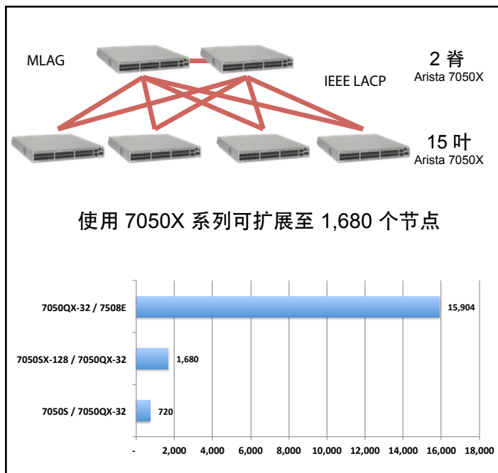
Arista L2 MLAG 叶子 - 骨干设计
