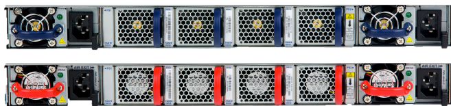
Arista 7050QX 1RU 后视图：
