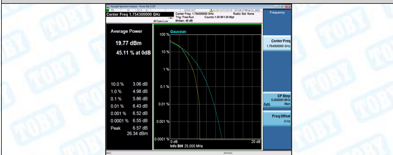
Band4-3MHz-QPSK-19965-1RB#0
