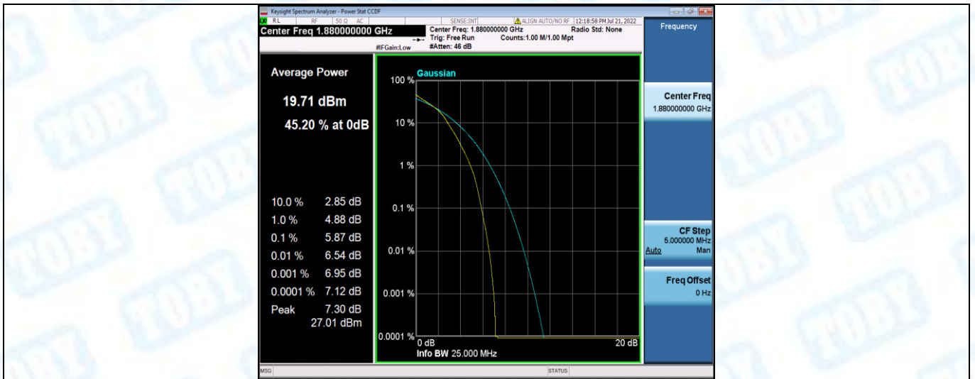
Band2-20MHz-16QAM-19100-1RB#0
