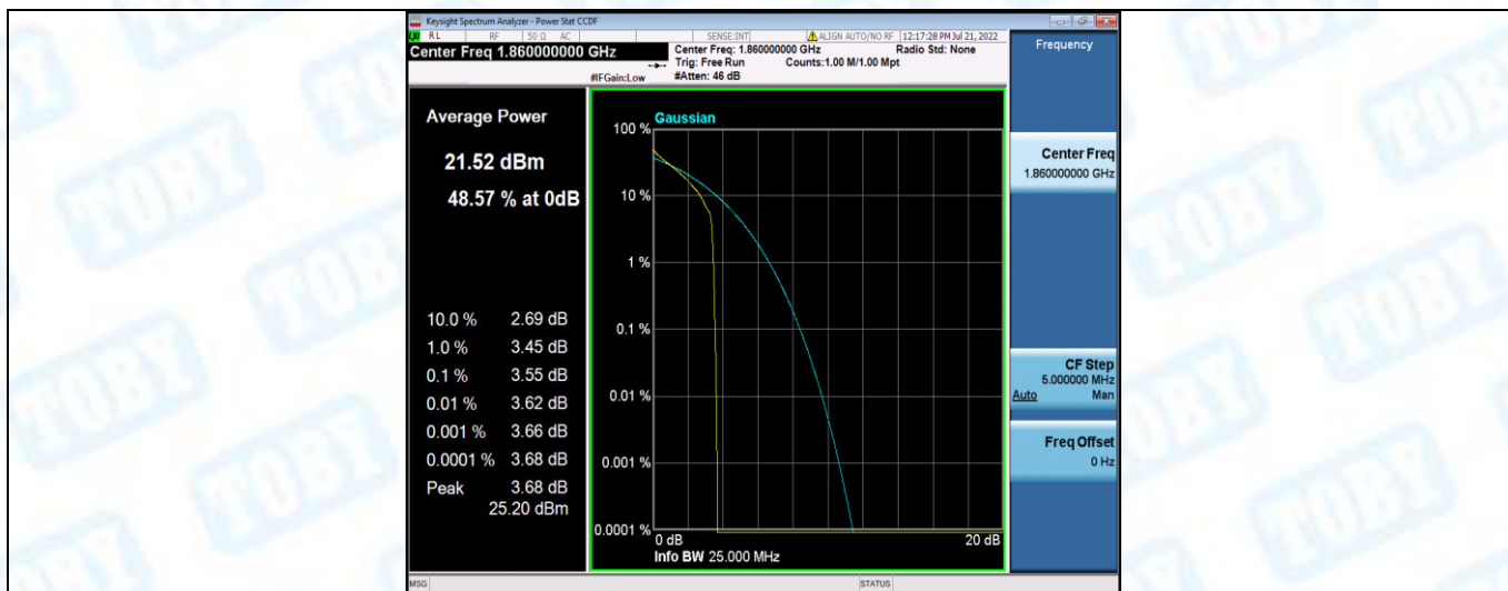
Band2-20MHz-QPSK-18700-100RB#0
