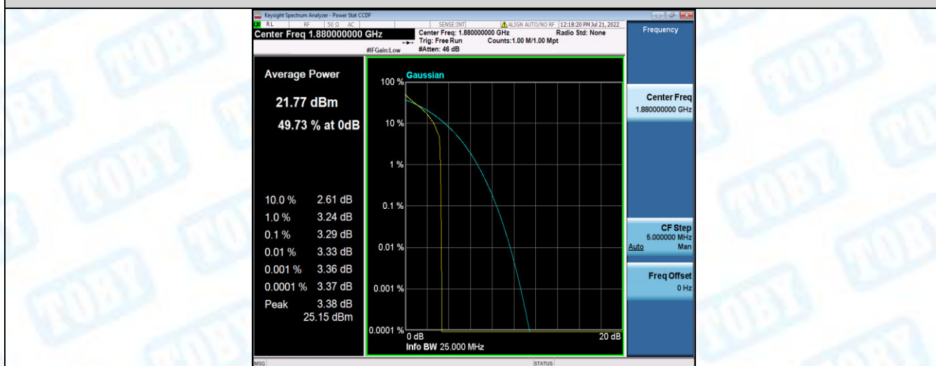
Band2-20MHz-QPSK-18900-100RB#0
