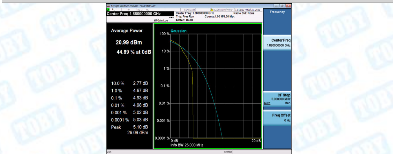
Band2-20MHz-16QAM-18900-100RB#0
