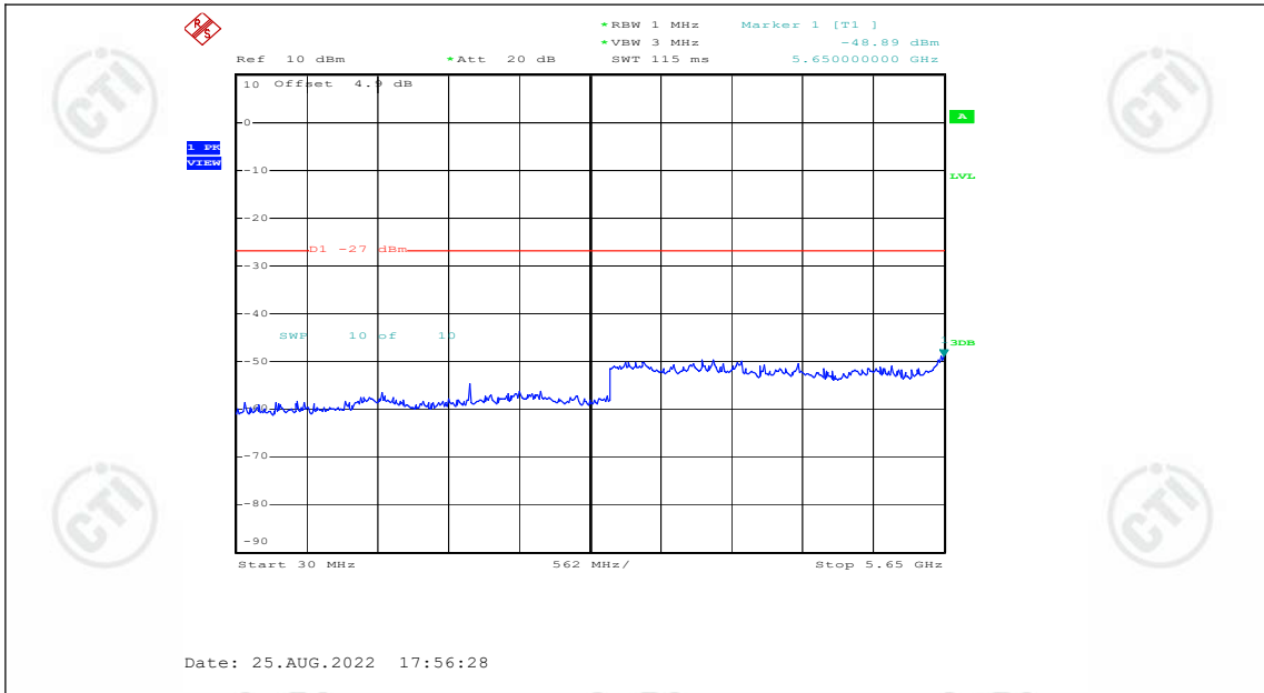
11AC80SISO_Ant1_5775_30~5650
