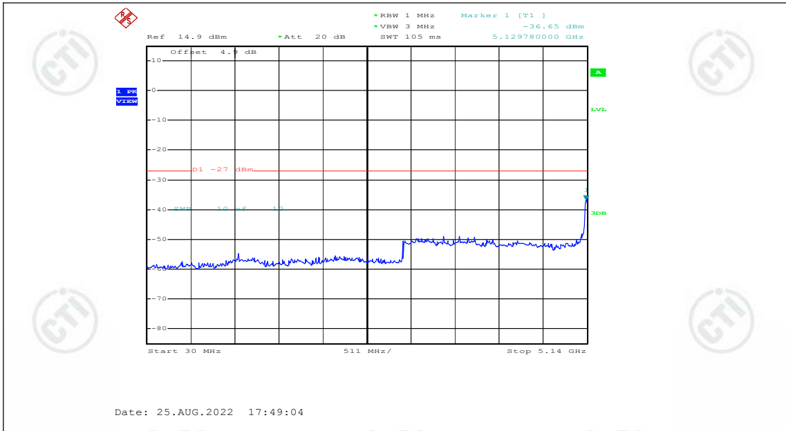
11AC80SISO_Ant1_5210_30~5140
