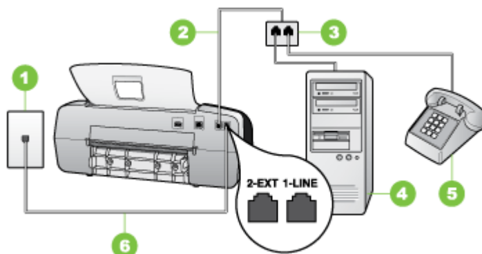
Рис. 7-8 Вид аппарата сзади
