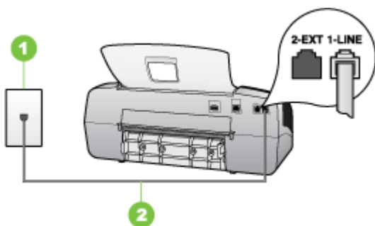
Рис. 7-1 Вид аппарата сзади
