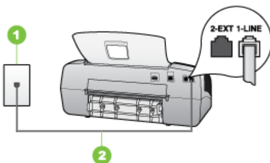
Рис. 7-3 Вид аппарата сзади
