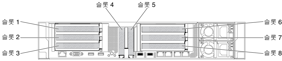
그림 124. PCI 라이저 카드 어댑터 확장 슬롯 위치
