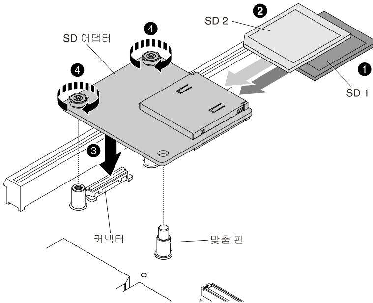
그림 207. SD 어댑터 설치
