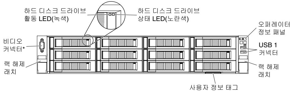
그림 15. 12 하드 디스크 드라이브 구성 앞면 보기
