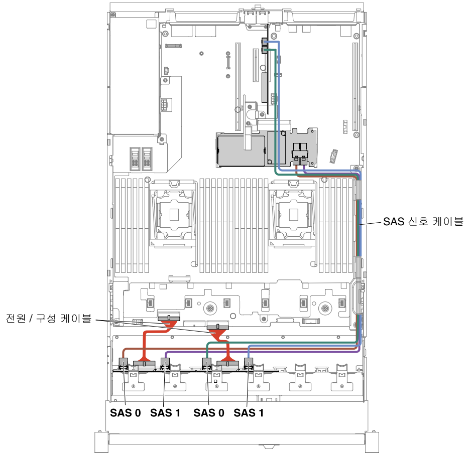
그림 269. 케이블 배선
