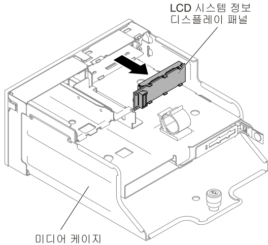
그림 212. LCD 시스템 정보 디스플레이 패널 제거
