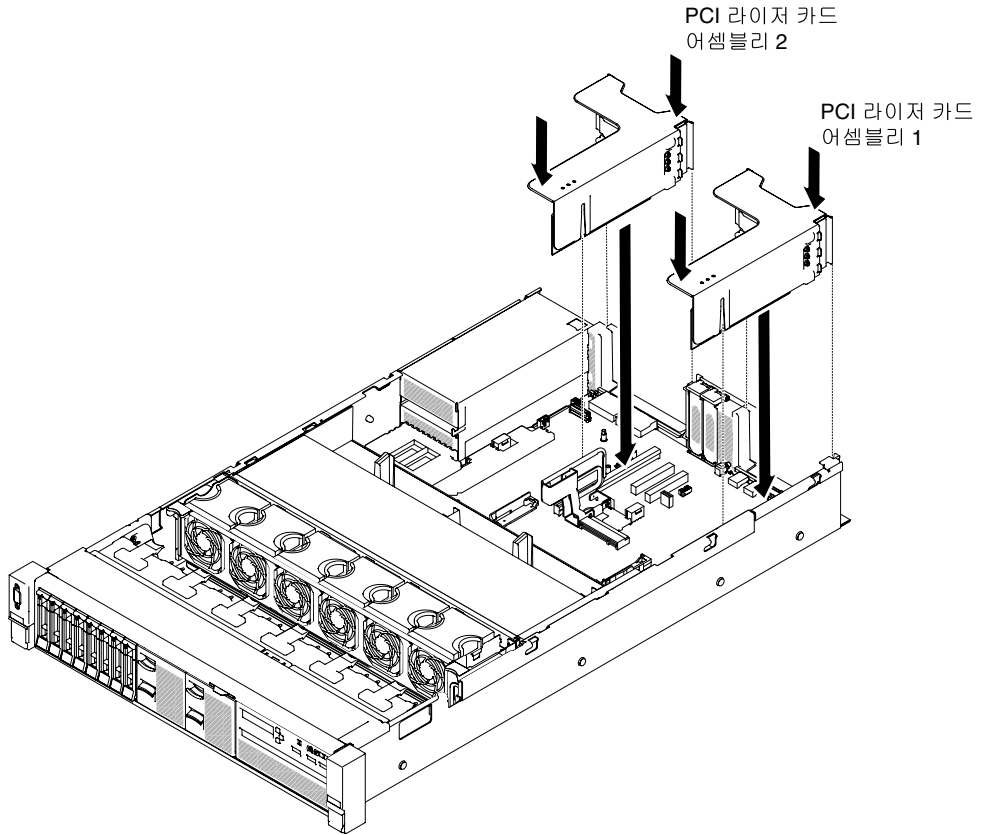
그림 129. 라이저 카드 어셈블리 설치 - 절반 길이 및 로우 프로파일 어댑터
