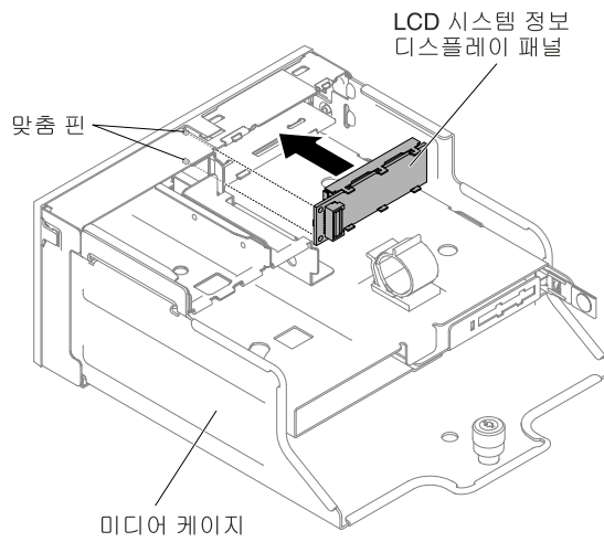
그림 221. LCD 시스템 정보 디스플레이 패널 설치
