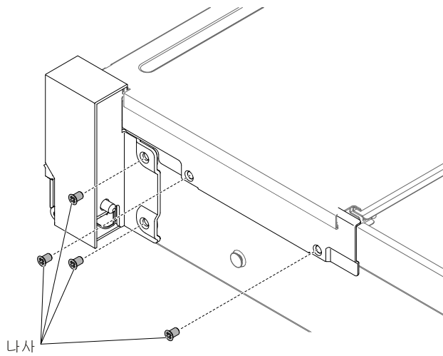
그림 180. 나사 설치
