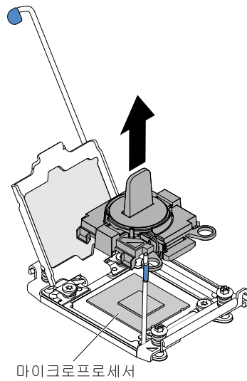
그림 247. 설치 도구 제거
