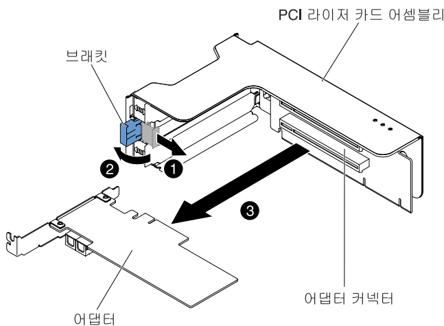
그림 121. 어댑터 제거
