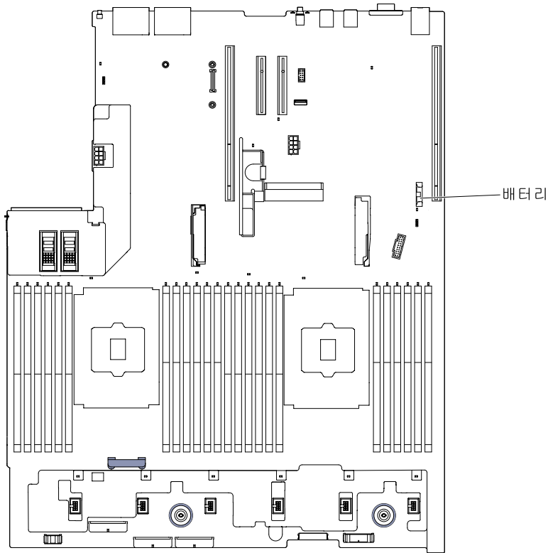
그림 204. 코인 셀 배터리 위치
