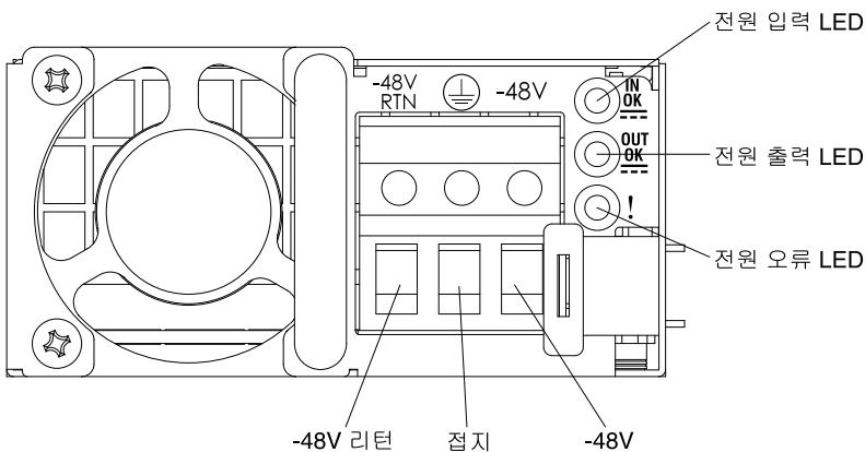
그림 46. DC 전원 공급 장치 LED
