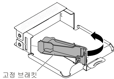
그림 215. 고정 브래킷 설치
