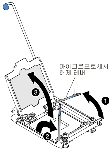
그림 243. 마이크로프로세서 소켓 레버 및 고정장치 분리
