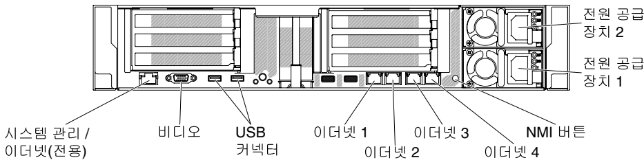
그림 21. 뒷면
