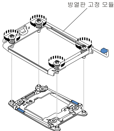
그림 256. 방열판 고정 모듈 제거
