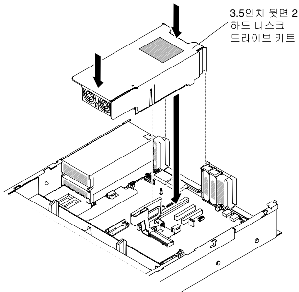
그림 143. 3.5인치 뒷면 2 하드 디스크 드라이브 키트 설치
