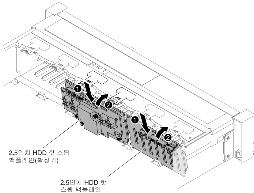
그림 275. 확장기 설치
