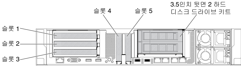
그림 125. PCI 라이저 카드 어댑터 확장 슬롯 위치
