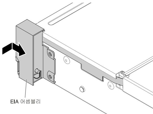
그림 178. EIA 어셈블리 설치
