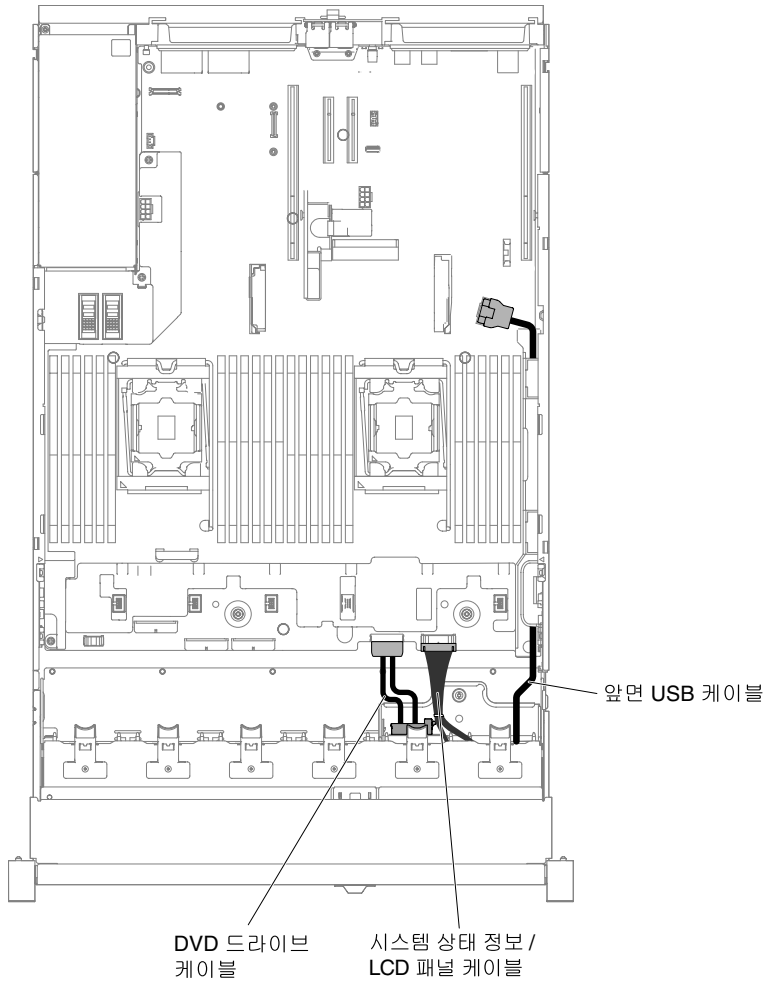
그림 105. 케이블 배선
