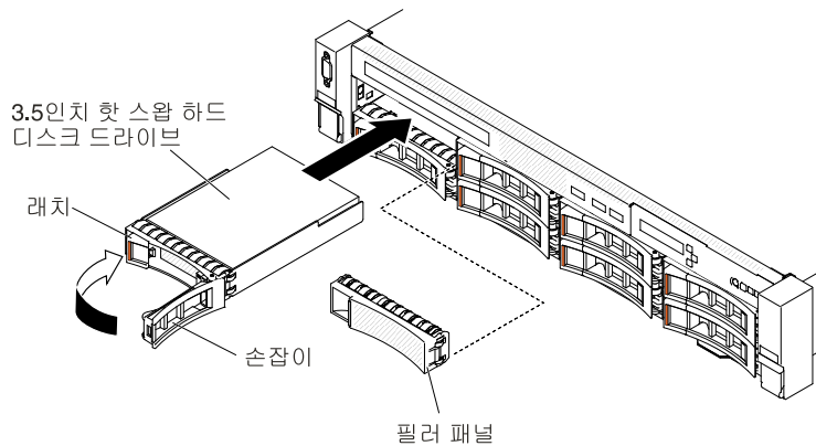
그림 83. 3.5인치 핫 스왑 하드 디스크 드라이브 설치
