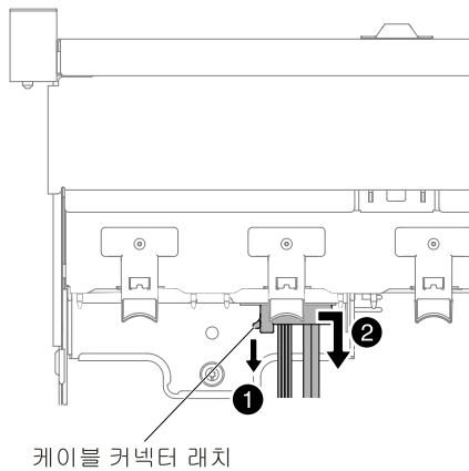
그림 89. 광 드라이브 케이블 래치
