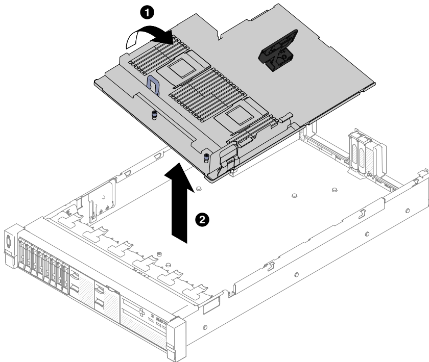
그림 259. 시스템 보드 제거
