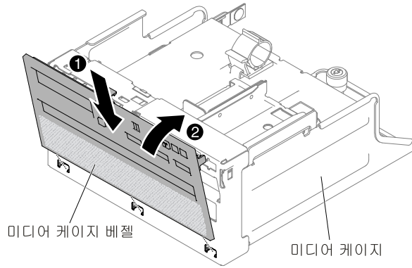
그림 224. 고정 브래킷 설치
