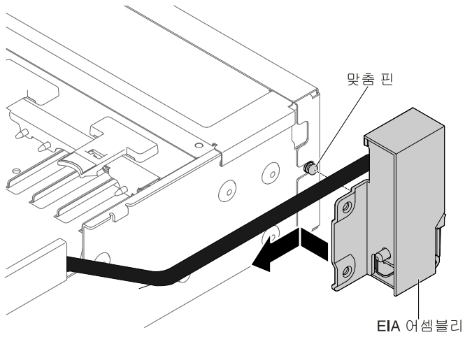
그림 172. EIA 어셈블리 정렬
