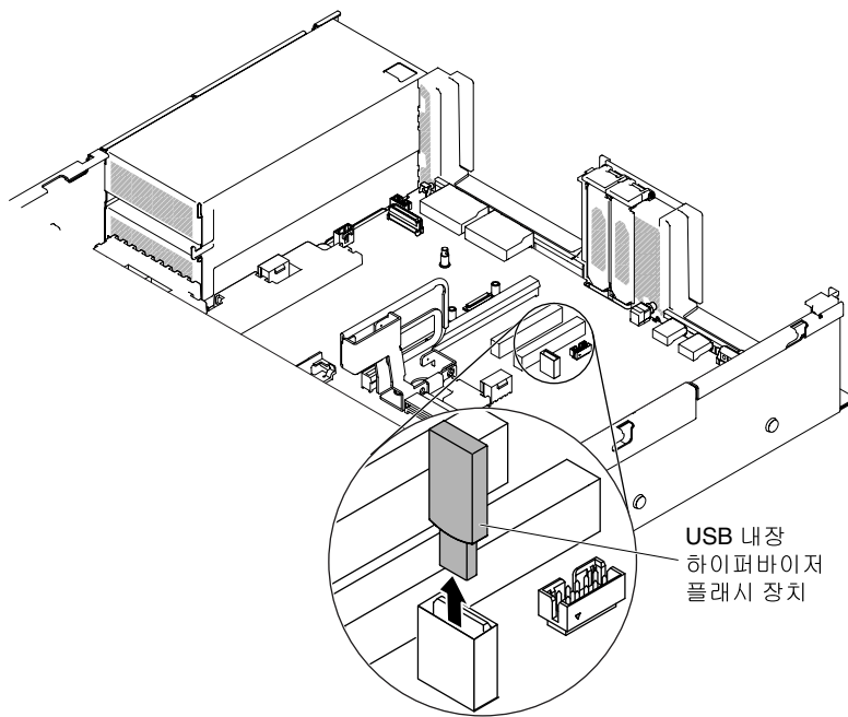
그림 200. USB 하이퍼바이저 플래시 장치, 제거
