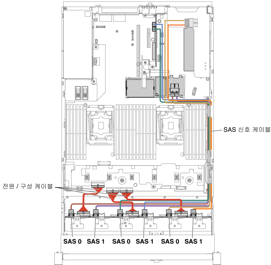
그림 61. 24x2.5인치 핫 스왑 하드 디스크 드라이브 케이블 연결
