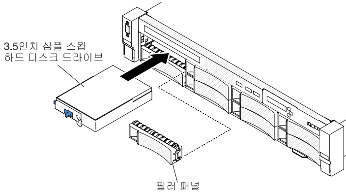
그림 87. 3.5인치 심플 스왑 하드 디스크 드라이브 설치
