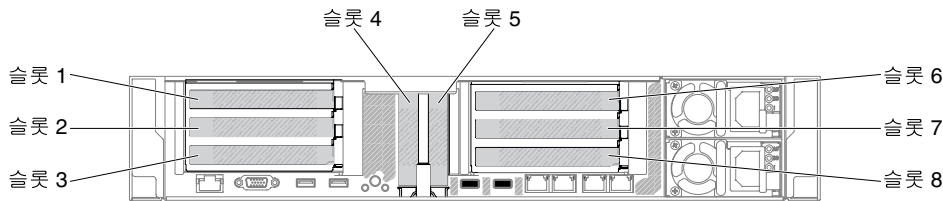
그림 23. PCI 라이저 카드 어댑터 확장 슬롯 위치
