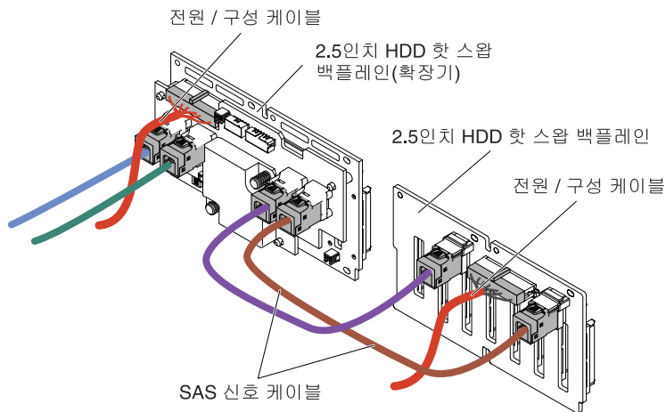
그림 276. 케이블 연결
