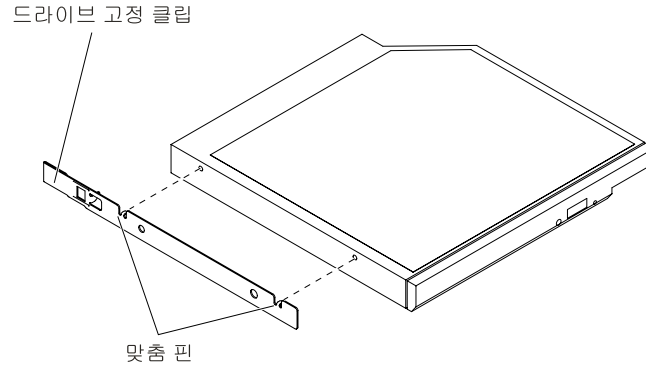
그림 94. 광 드라이브 고정 클립 설치
