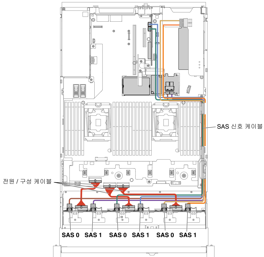
그림 270. 케이블 연결
