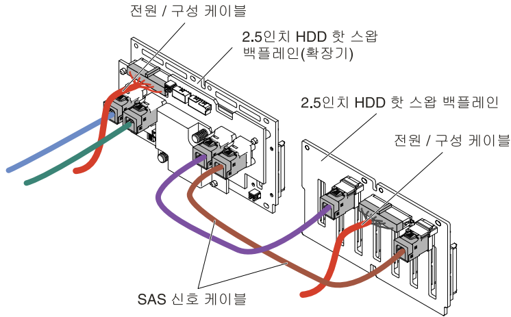
그림 58. 16x2.5인치 핫 스왑 하드 디스크 드라이브 케이블 연결
