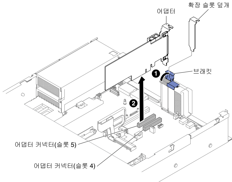
그림 131. 어댑터 설치
