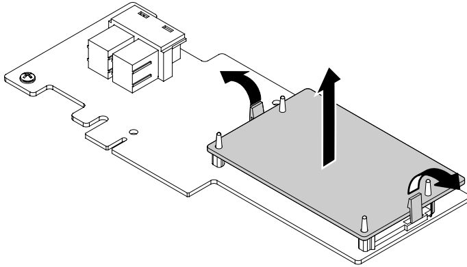
그림 230. ServeRAID 어댑터 메모리 모듈 제거
