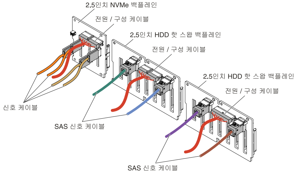
그림 284. 케이블 연결
