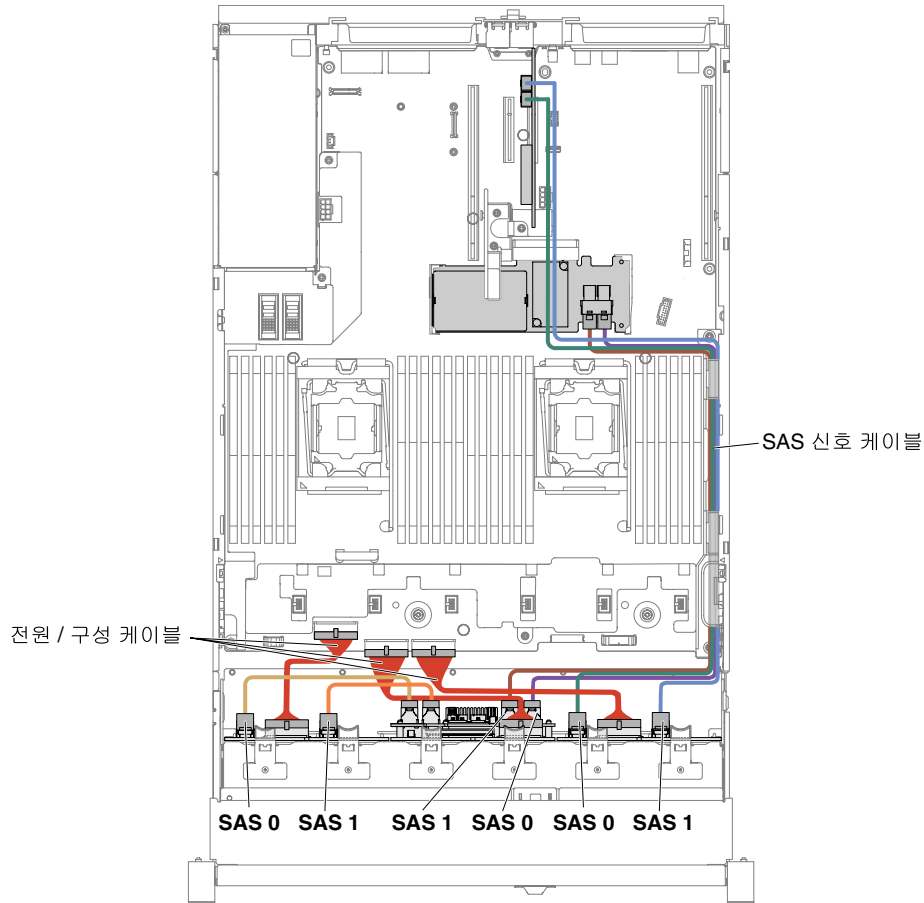
그림 273. 케이블 배선
