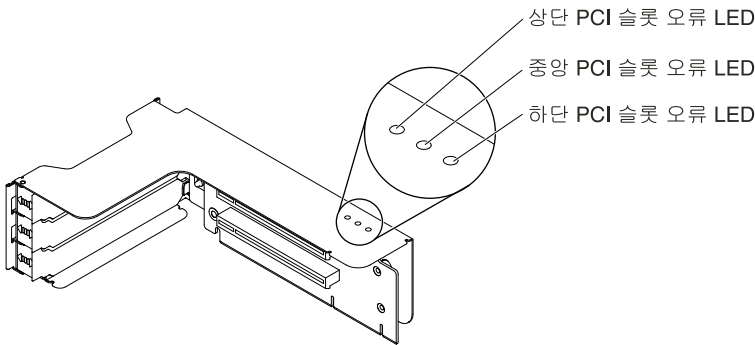
그림 47. PCI 라이저 카드 LED
