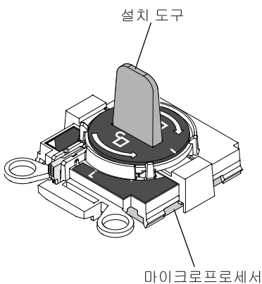
그림 232. 마이크로프로세서 설치 도구
