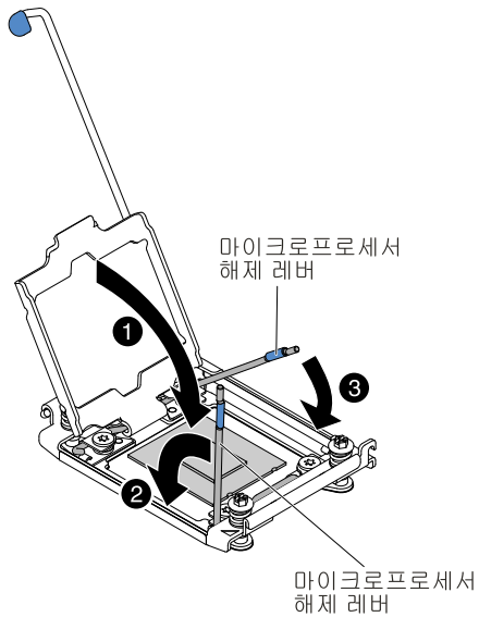
그림 249. 마이크로프로세서 소켓 레버 및 고정장치 고정
