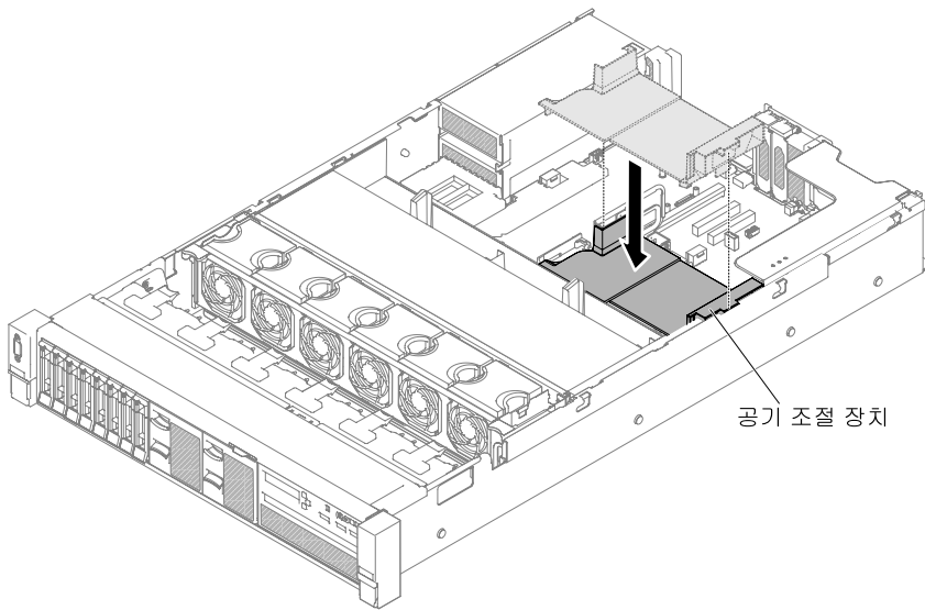
그림 288. 공기 조절 장치 설치
