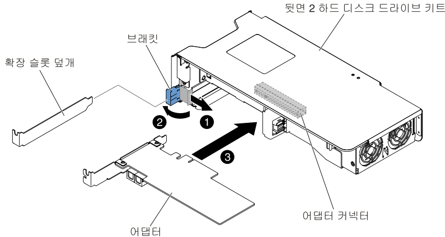
그림 132. 어댑터 설치
