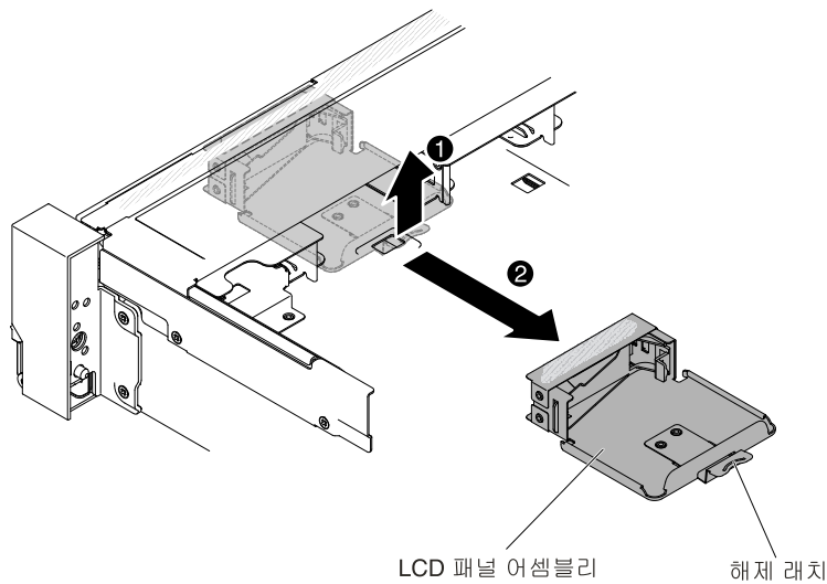
그림 208. LCD 패널 어셈블리 제거
