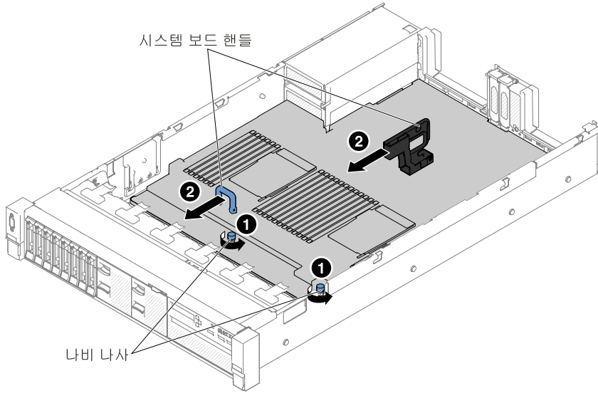
그림 258. 시스템 보드 제거
