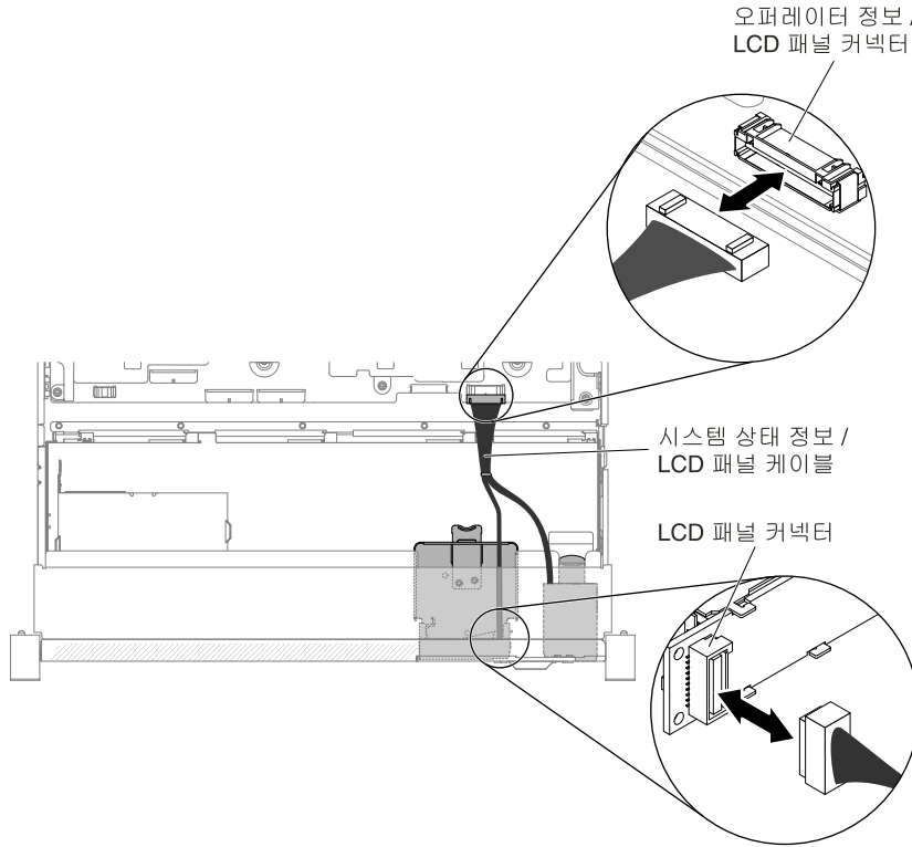
그림 217. LCD 패널 어셈블리 케이블 배선
