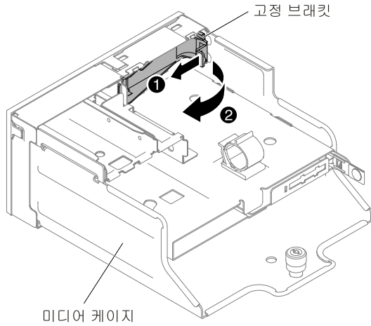
그림 220. 고정 브래킷 제거
