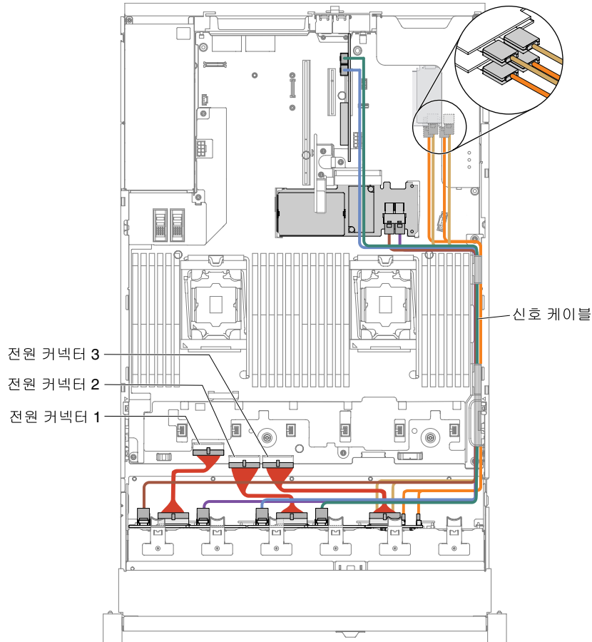
그림 287. 케이블 배선
