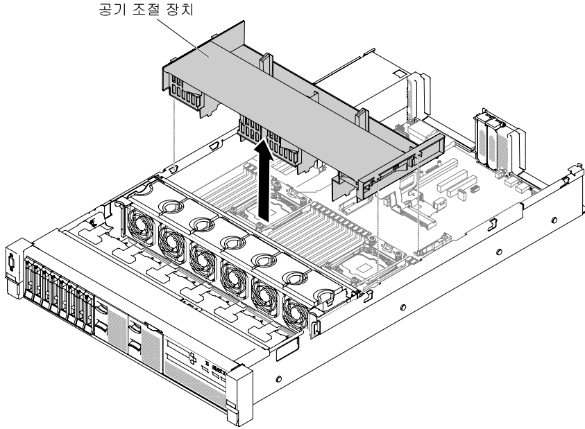
그림 73. 공기 조절 장치 제거
