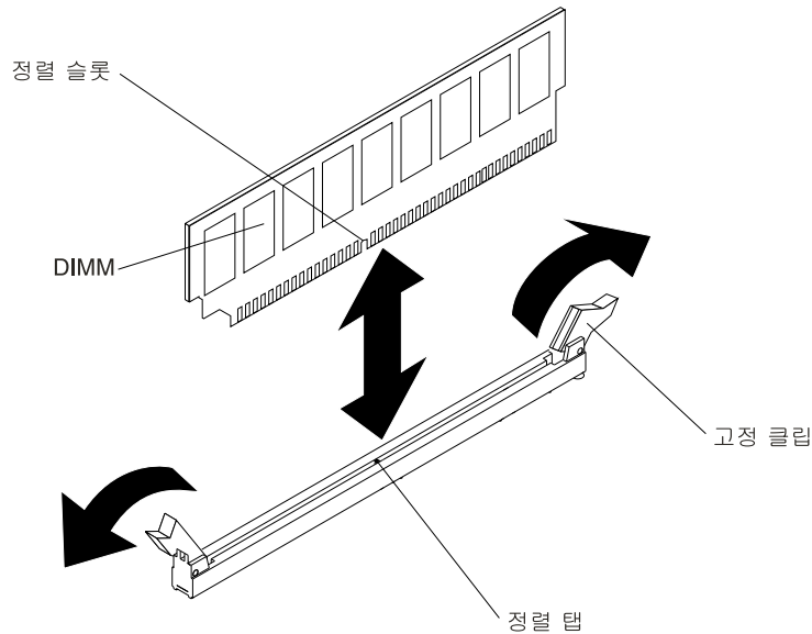
그림 96. DIMM 제거
