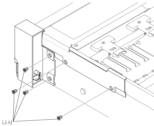
그림 169. 나사 설치
