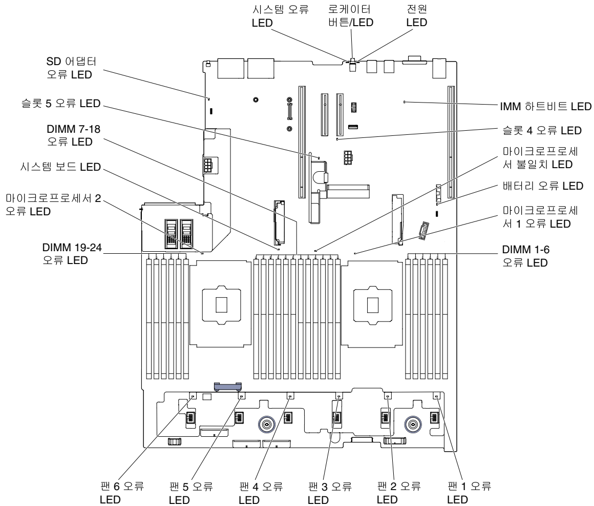
그림 31. 시스템 보드 LED
