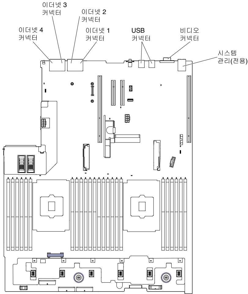
그림 28. 시스템 보드 외부 커넥터
