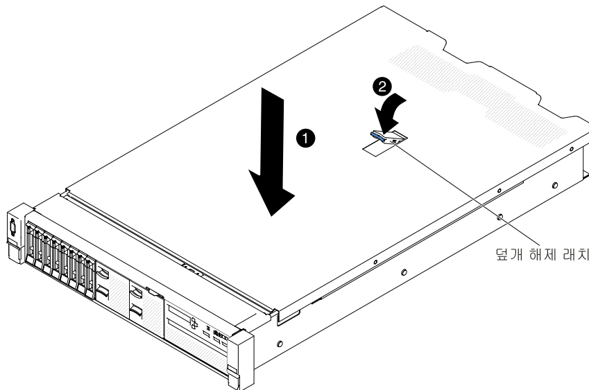
그림 71. 윗면 덮개 설치
