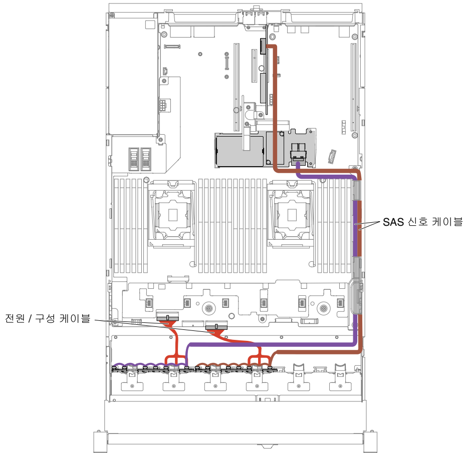
그림 55. 하드웨어 RAID 케이블이 연결된 16x2.5인치 심플 스왑 하드 디스크 드라이브
