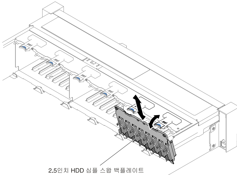
그림 262. 2.5인치 심플 스왑/핫 스왑 하드 디스크 드라이브 백플레이트 어셈블리/백플레이트 설치
