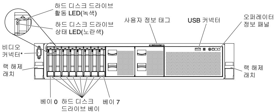
그림 10. 8 하드 디스크 드라이브 구성 / 16 하드 디스크 드라이브 구성 1
