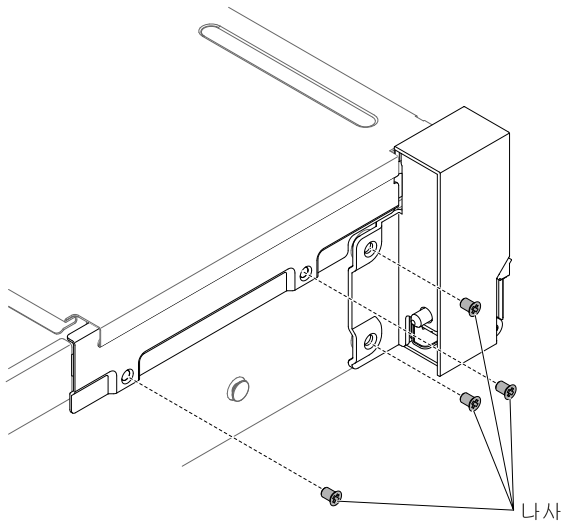
그림 162. 나사 제거
