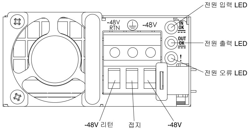
그림 191. DC 전원 공급 장치 뒷면
