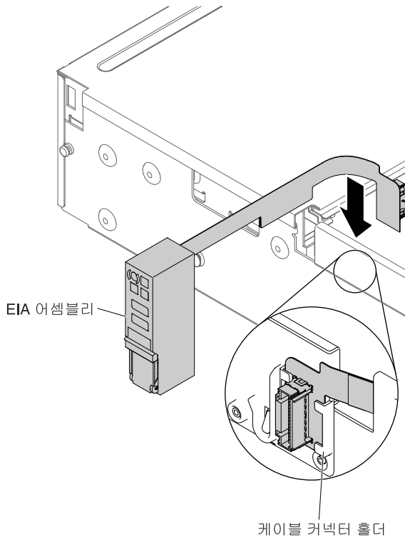
그림 176. 케이블 커넥터 설치
