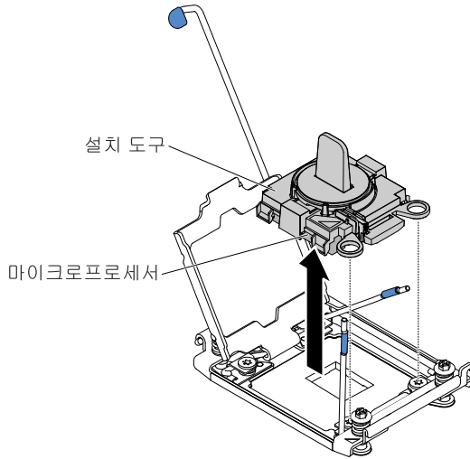
그림 240. 설치 도구 제거
