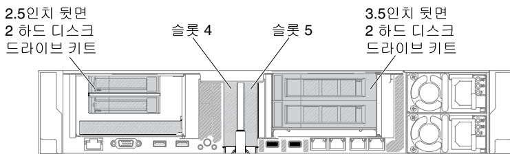
그림 25. PCI 라이저 카드 어댑터 확장 슬롯 위치
