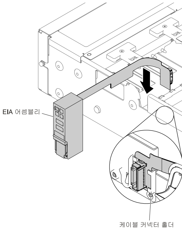
그림 165. 케이블 커넥터 설치
