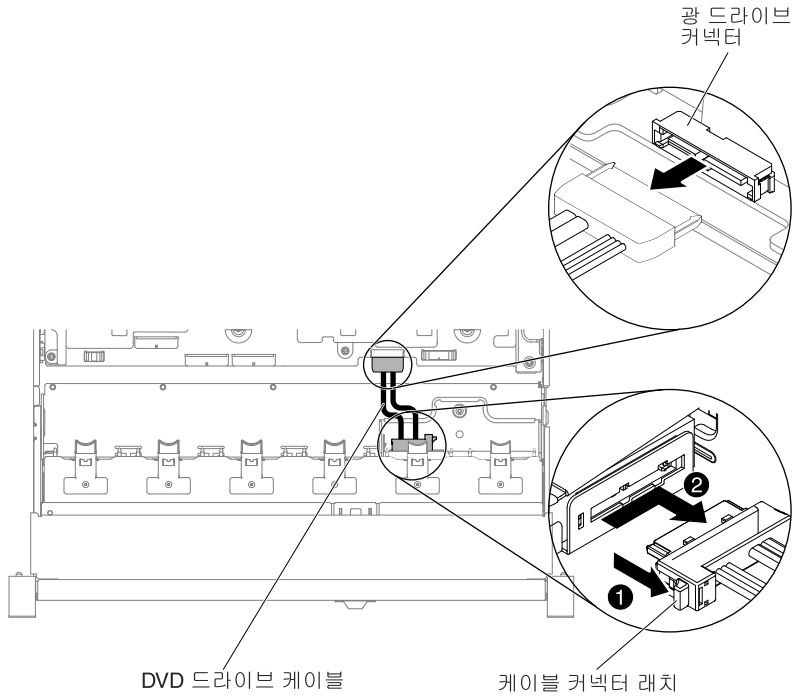
그림 88. 광 드라이브 케이블 연결
