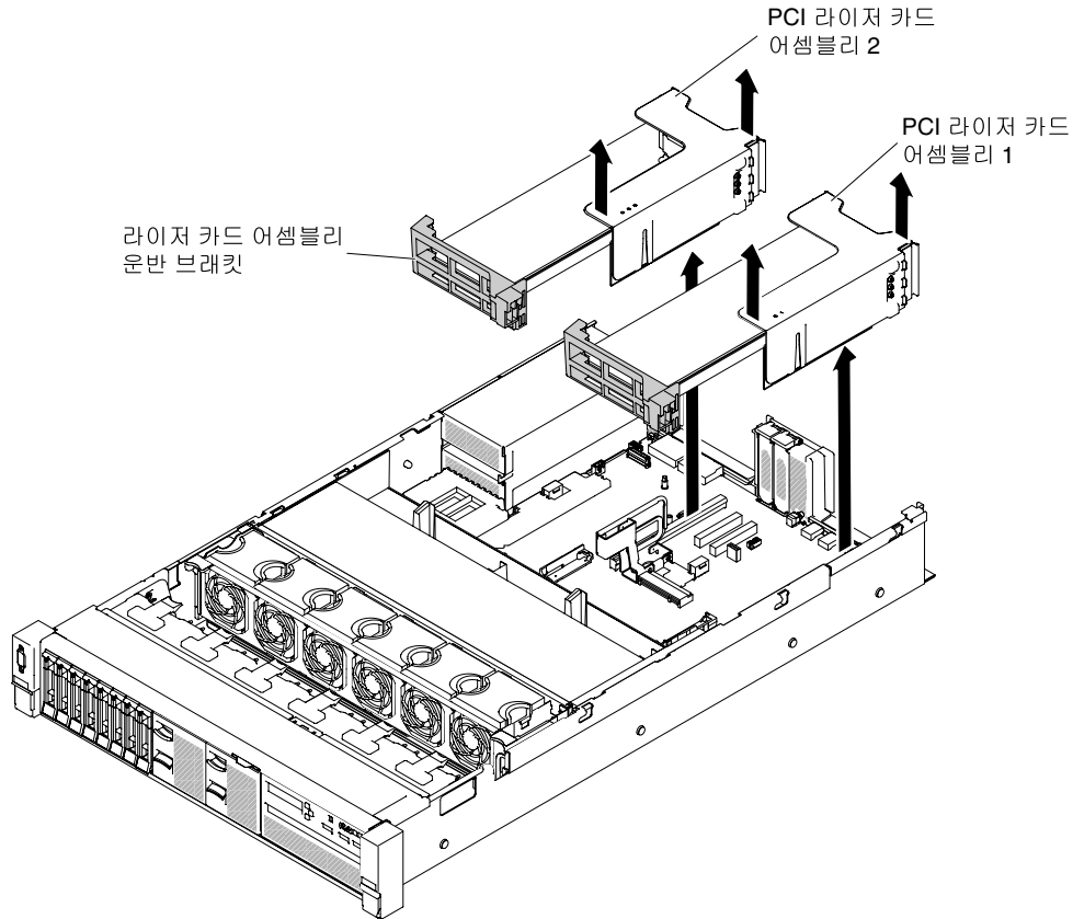
그림 112. 라이저 카드 어셈블리 제거 - 전체 높이, 전체 길이 어댑터
