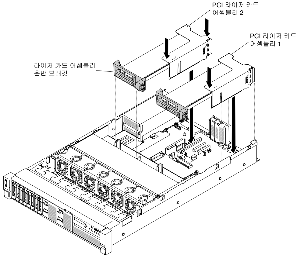
그림 130. 라이저 카드 어셈블리 설치 - 전체 높이, 전체 길이 어댑터
