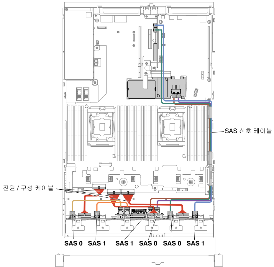
그림 279. 케이블 배선
