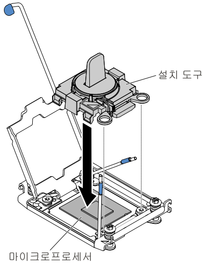
그림 238. 설치 도구 정렬
