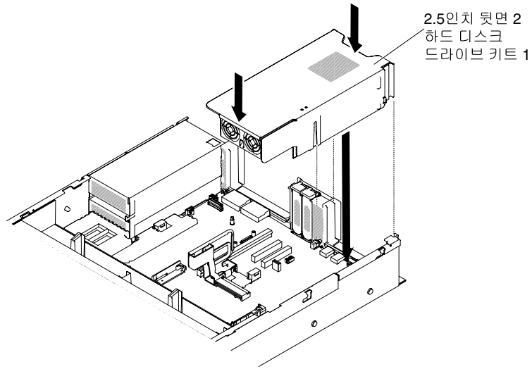
그림 142. 2.5인치 뒷면 2 하드 디스크 드라이브 키트 설치
