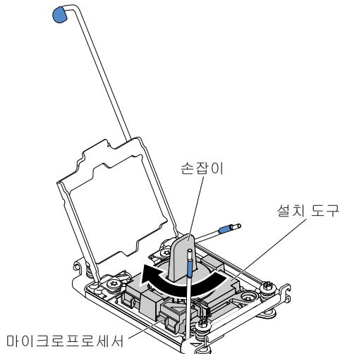
그림 239. 설치 도구 손잡이 조정
