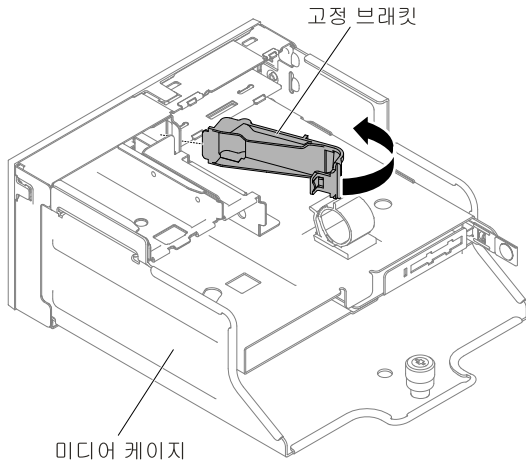
그림 222. 고정 브래킷 설치
