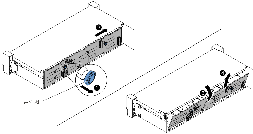
그림 197. 3.5인치 핫 스왑 하드 디스크 드라이브 백플레인 제거
