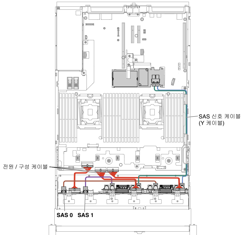
그림 280. 케이블 연결
