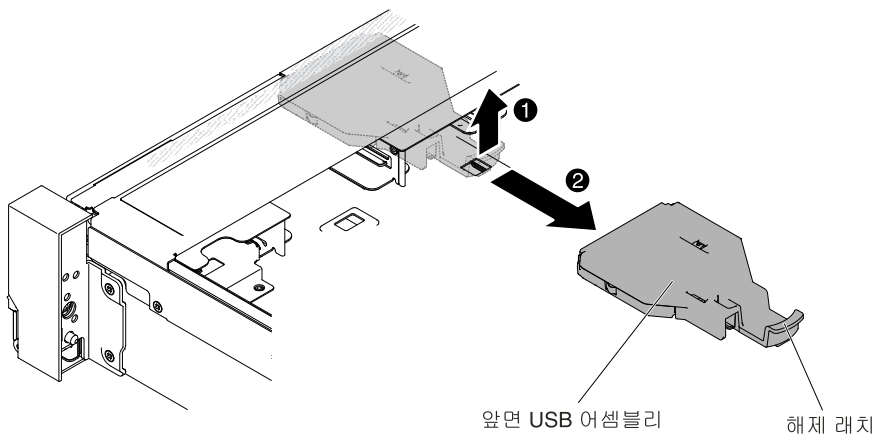
그림 77. 앞면 USB 어셈블리 제거
