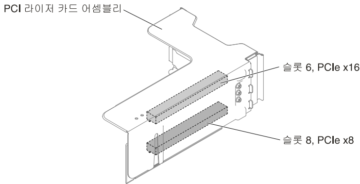
그림 37. 유형 6 PCI 라이저 카드
