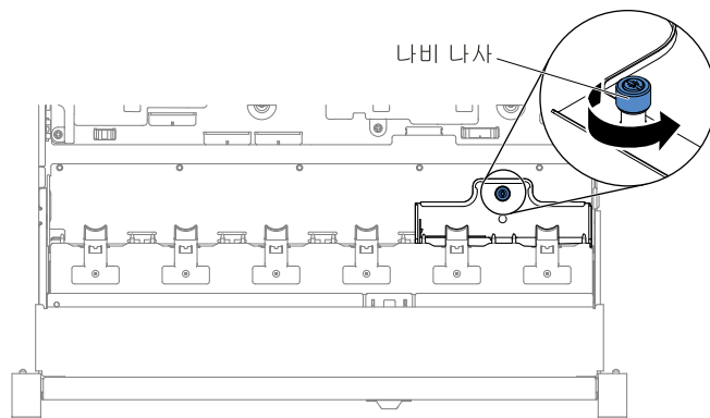
그림 106. 나비 나사
