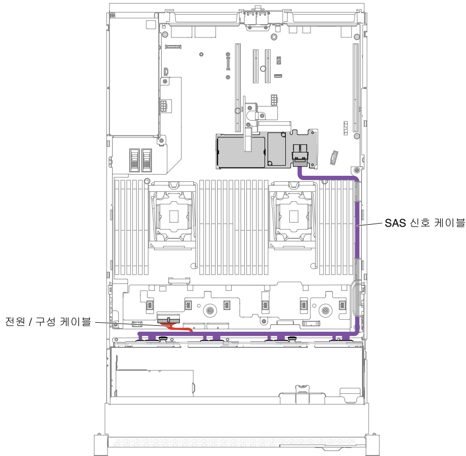
그림 265. 하드웨어 RAID 케이블이 연결된 8x3.5인치 심플 스왑 하드 디스크 드라이브
