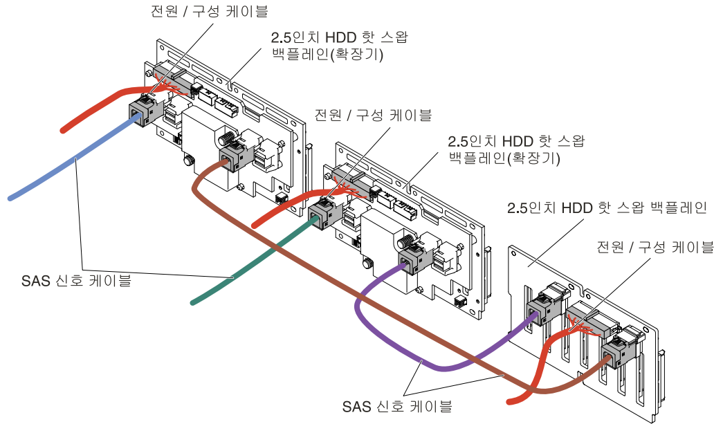
그림 280. 케이블 연결
