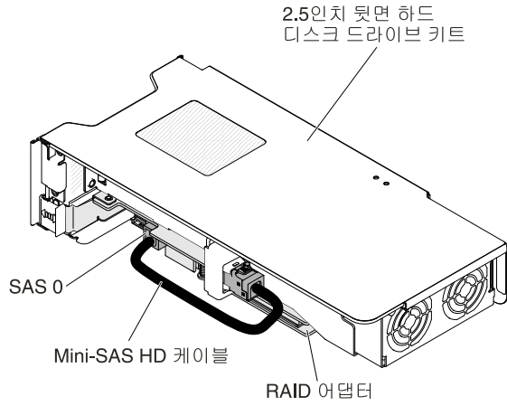
그림 144. 2.5인치 뒷면 2 하드 디스크 드라이브 키트 케이블 배선
