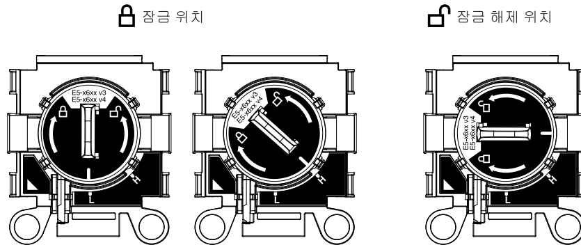
그림 237. 잠금 및 잠금 해제 위치
