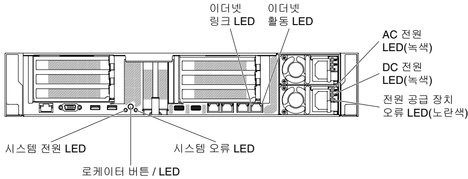
그림 22. LED 뒷면
