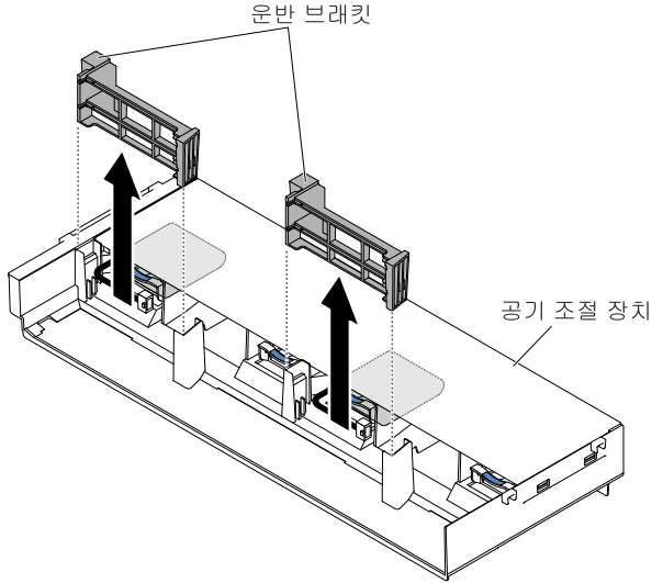
그림 134. 운반 브래킷 제거
