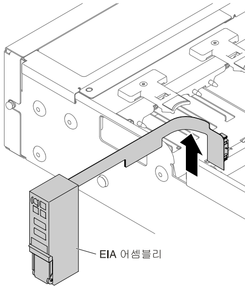
그림 151. EIA 어셈블리 제거
