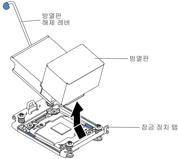
그림 234. 방열판 제거
