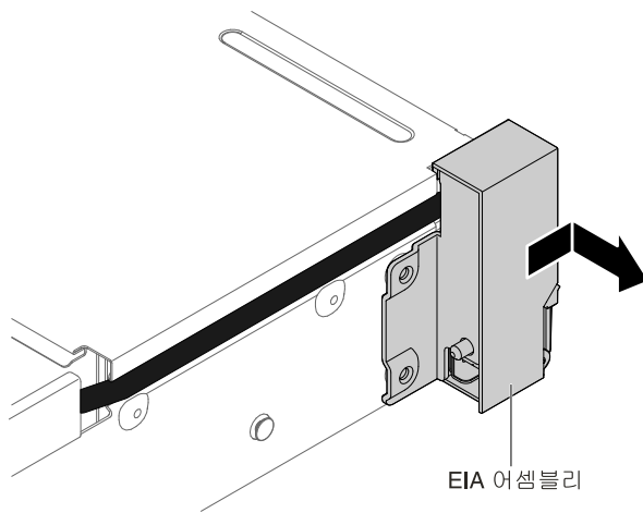
그림 164. EIA 어셈블리 제거
