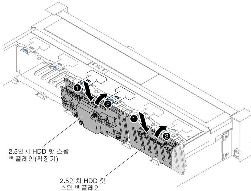
그림 195. 2.5인치 심플 스왑 백플레이트 어셈블리/핫 스왑 하드 디스크 드라이브 백플레인 설치
