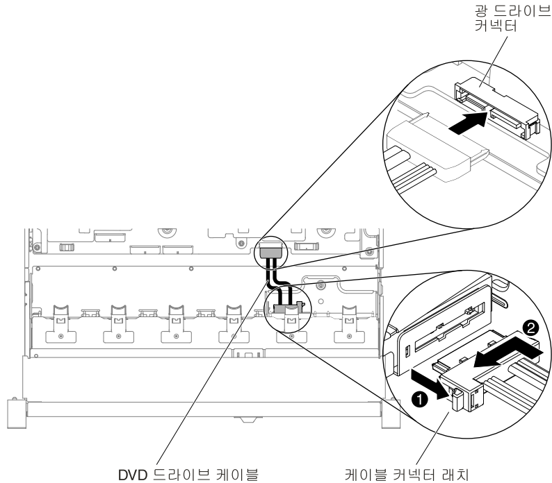
그림 91. 광 드라이브 케이블 배선
