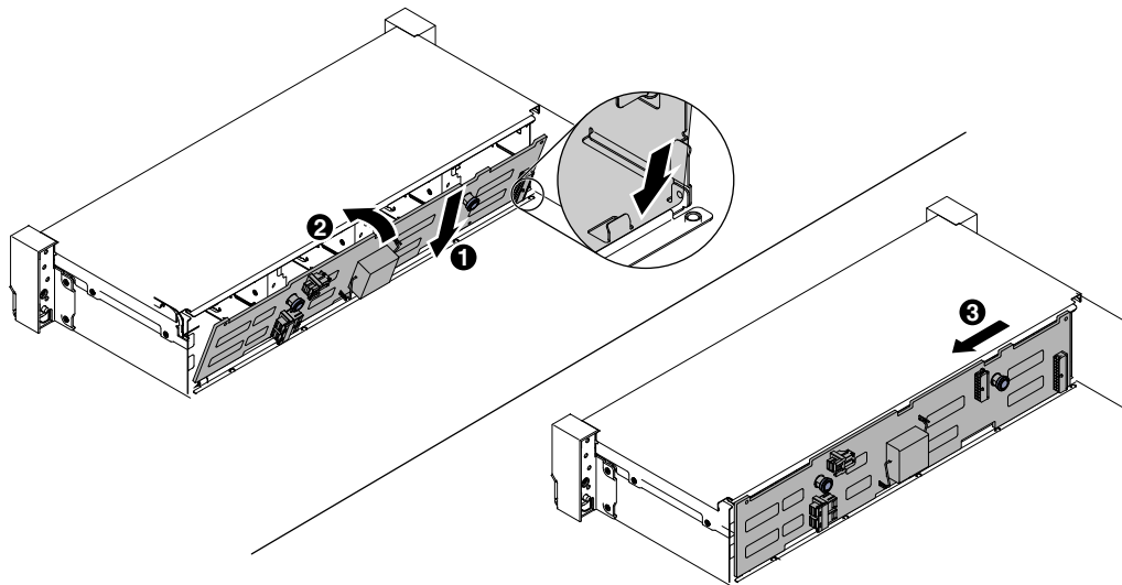
그림 199. 3.5인치 핫 스왑 하드 디스크 드라이브 백플레이트 설치
