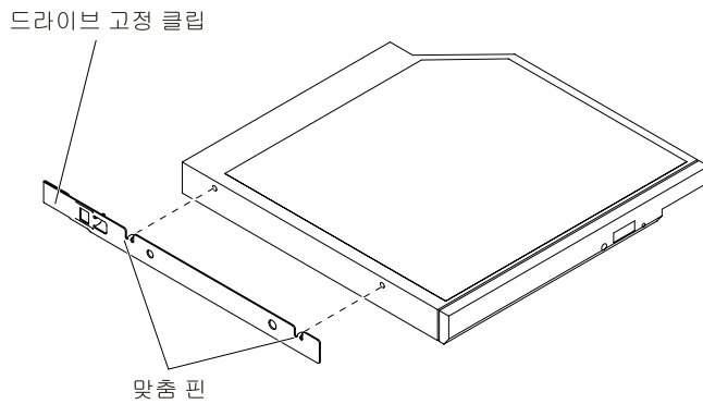
그림 93. 광 드라이브 고정 클립 제거
