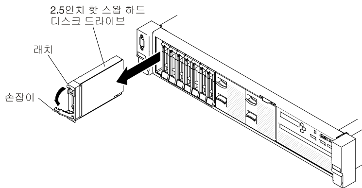
그림 80. 2.5인치 핫 스왑 하드 디스크 드라이브 제거
