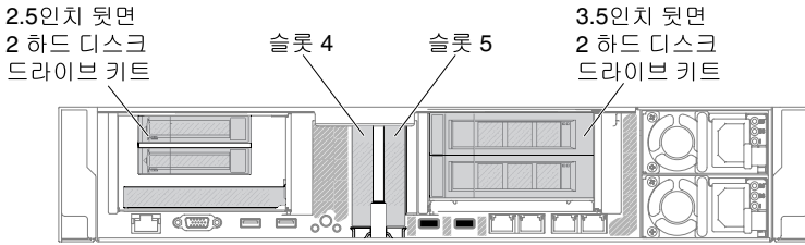
그림 119. PCI 라이저 카드 어댑터 확장 슬롯 위치
