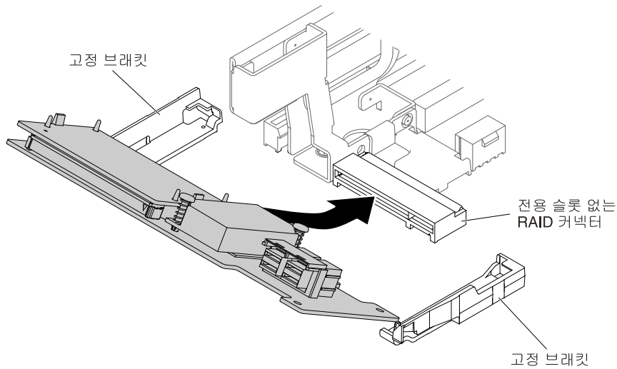
그림 116. 전용 슬롯 없는 RAID 컨트롤러 설치
