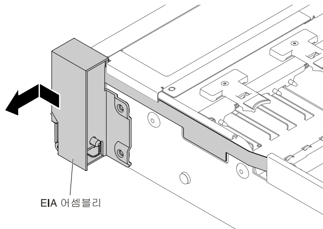
그림 150. EIA 어셈블리 제거
