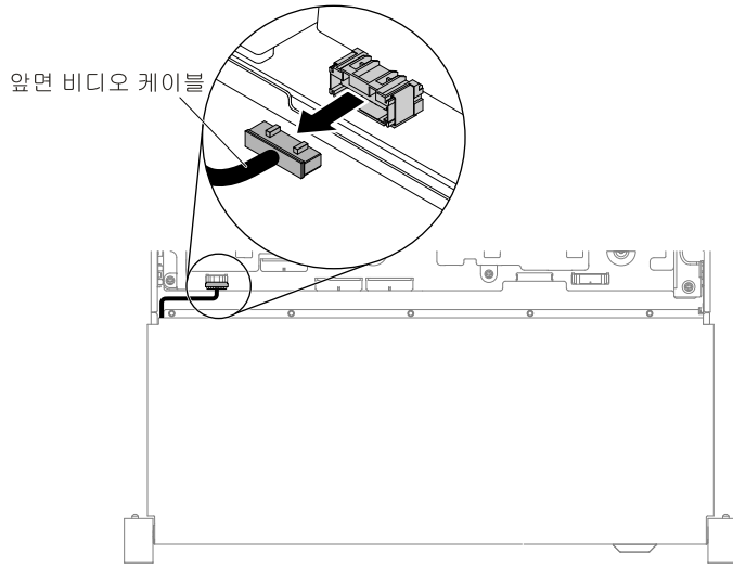
그림 161. 앞면 비디오 케이블 제거
