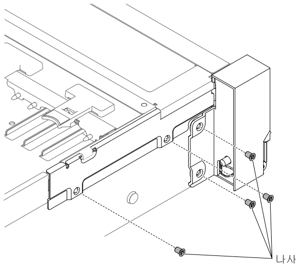
그림 153. 나사 제거
