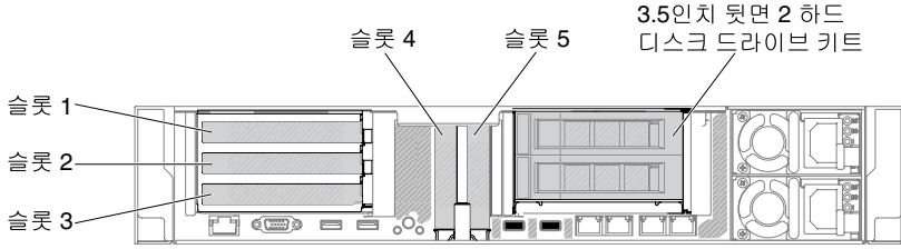
그림 118. PCI 라이저 카드 어댑터 확장 슬롯 위치
