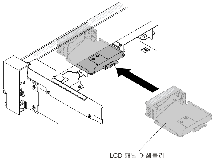
그림 216. LCD 패널 어셈블리 설치
