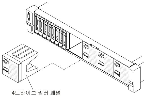
그림 266. 필터 패널
