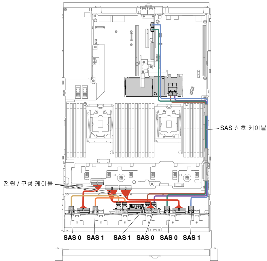
그림 63. 24x2.5인치 핫 스왑 하드 디스크 드라이브 케이블 연결
