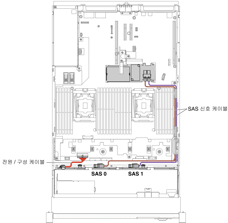
그림 67. 8x3.5인치 핫 스왑 하드 디스크 드라이브 케이블 연결
