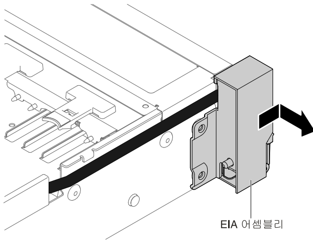
그림 155. EIA 어셈블리 제거
