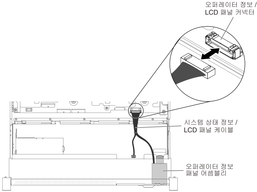
그림 227. 오퍼레이터 정보 패널 케이블 배선
