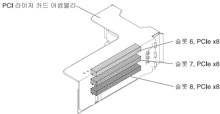
그림 36. 유형 5 PCI 라이저 카드
