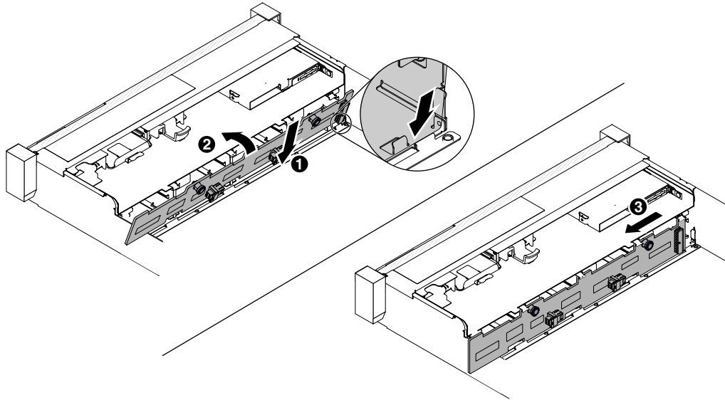
그림 198. 3.5인치 심플 스왑 백플레이트 어셈블리/핫 스왑 하드 디스크 드라이브 백플레이트 8개
