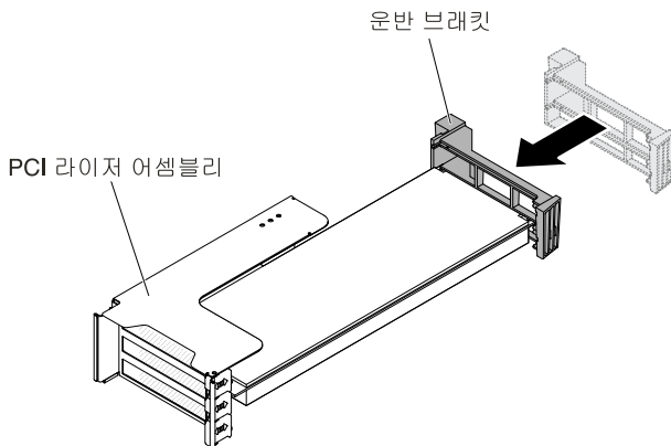
그림 128. 전체 높이, 전체 길이 어댑터
