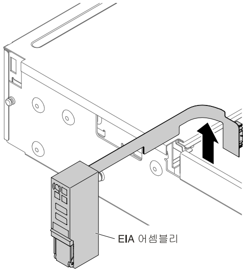
그림 160. 케이블 제거
