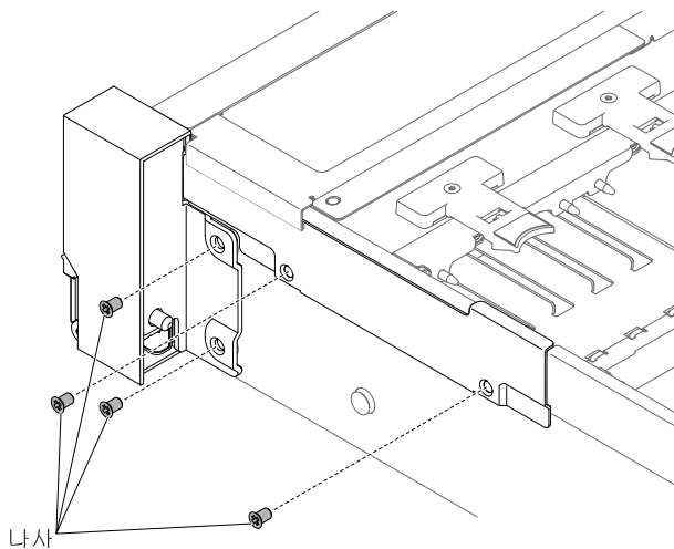
그림 148. 나사 제거
