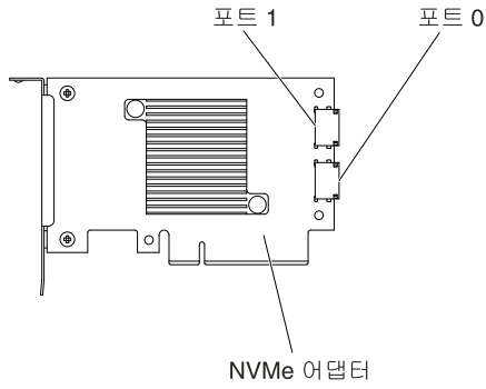
그림 285. NVMe 어댑터 커넥터
