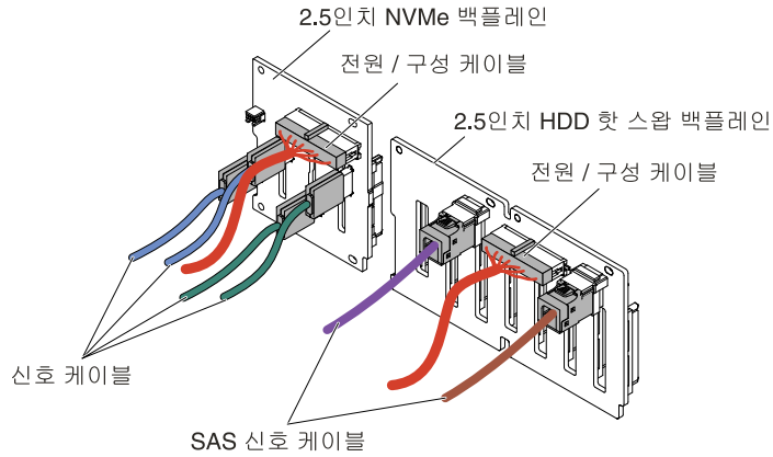
그림 283. 케이블 연결
