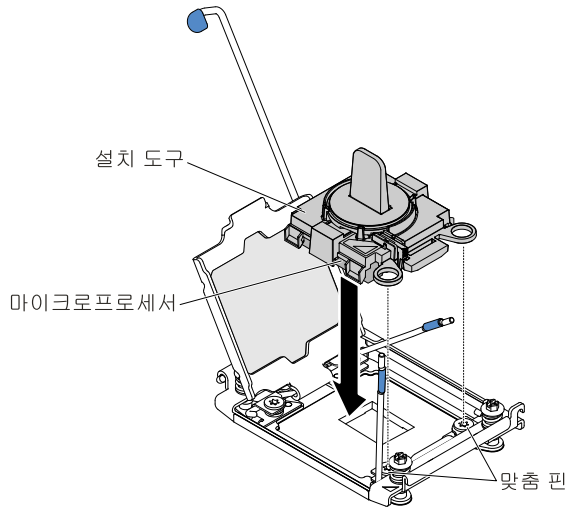
그림 244. 설치 도구 정렬
