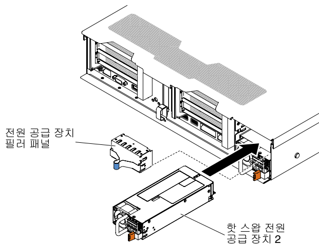
그림 192. 전원 공급 장치 설치
