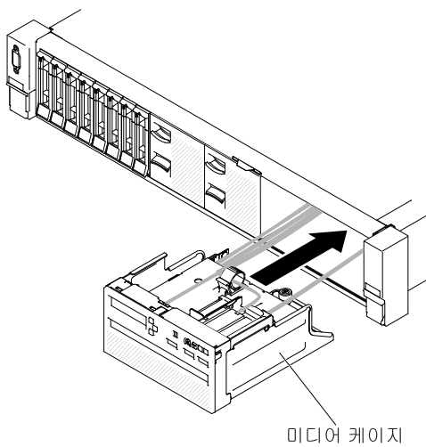
그림 108. 미디어 케이지 설치
