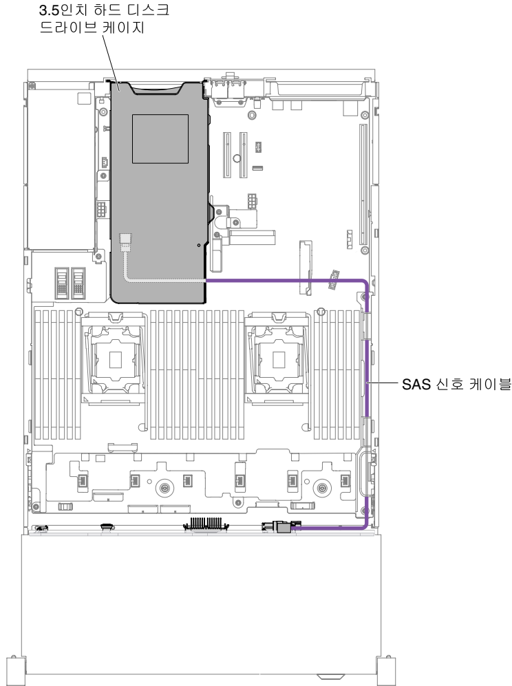
그림 146. 3.5인치 뒷면 2 하드 디스크 드라이브 키트 케이블 배선
