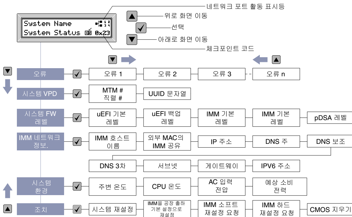
그림 19. LCD 시스템 정보 디스플레이 패널 메뉴 옵션 흐름
