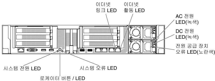
그림 45. AC 전원 공급 장치 LED
