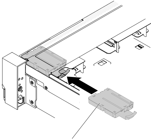
오퍼레이터 정보 패널 어셈블리
