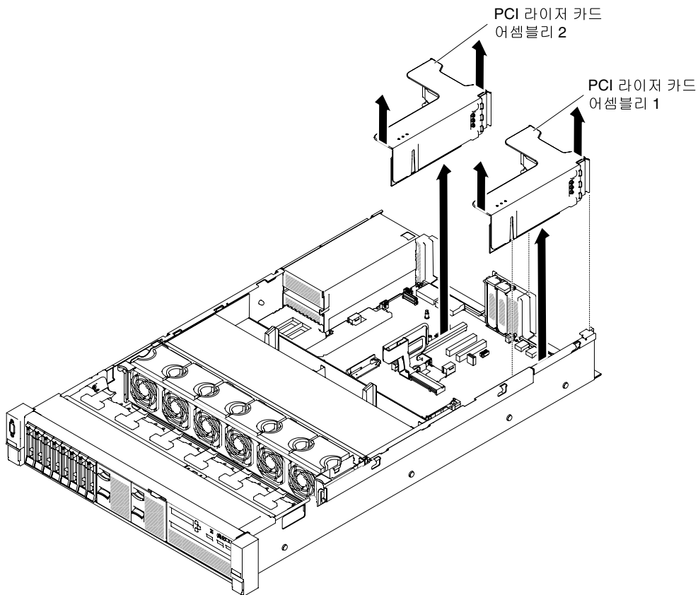
그림 111. 라이저 카드 어셈블리 제거 - 절반 길이 및 로우 프로파일 어댑터
