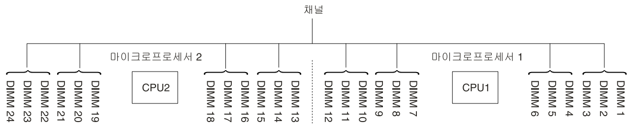
그림 98. 각 메모리 채널의 커넥터
