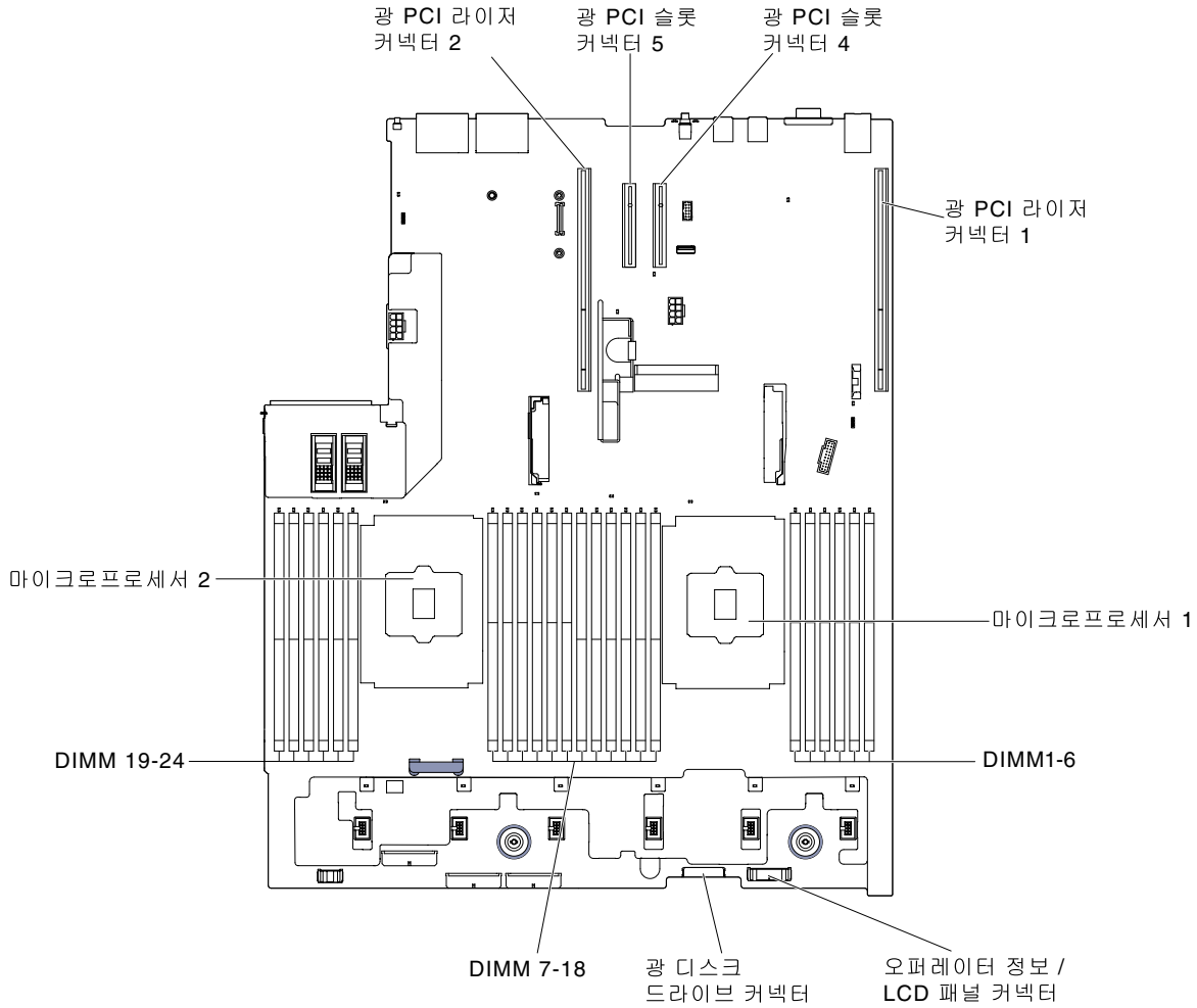
그림 29. 시스템 보드 옵션 장치 커넥터
