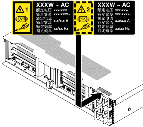
그림 189. 중복 전원 정보 레이블 부착
