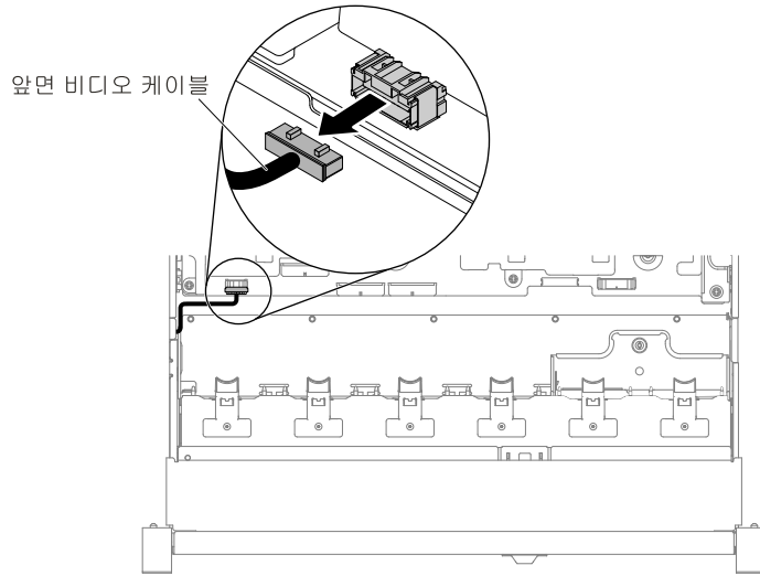
그림 152. 앞면 비디오 케이블 제거
