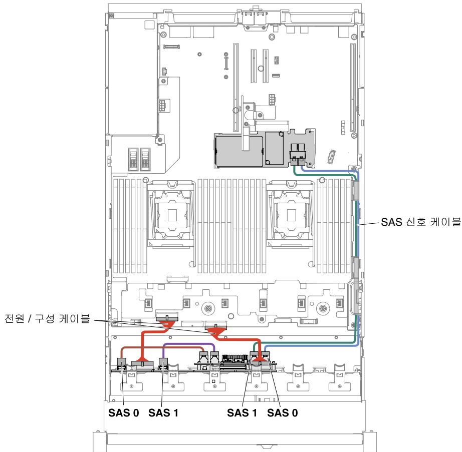
그림 59. 16x2.5인치 핫 스왑 하드 디스크 드라이브 케이블 연결
