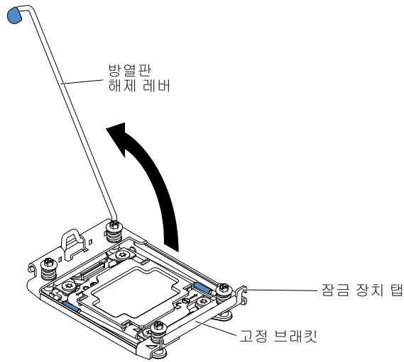
그림 242. 방열판 레버 회전
