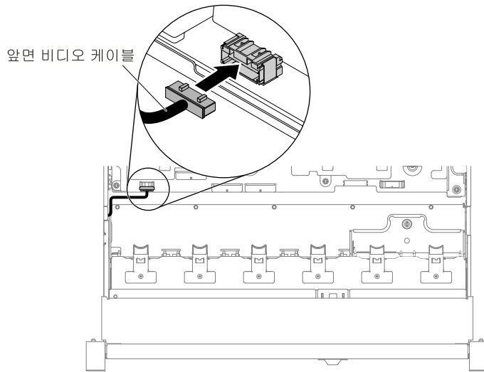
그림 175. 케이블 연결
