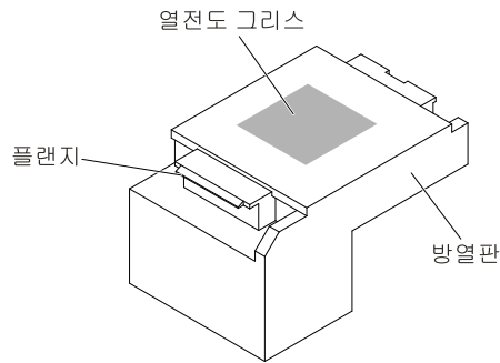
그림 250. 열전도 그리스
