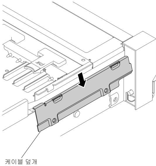
그림 154. 케이블 덮개 제거
