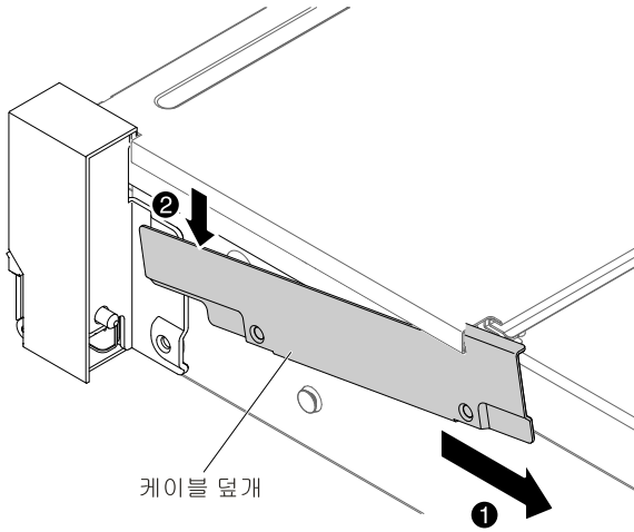
그림 158. 케이블 덮개 제거
