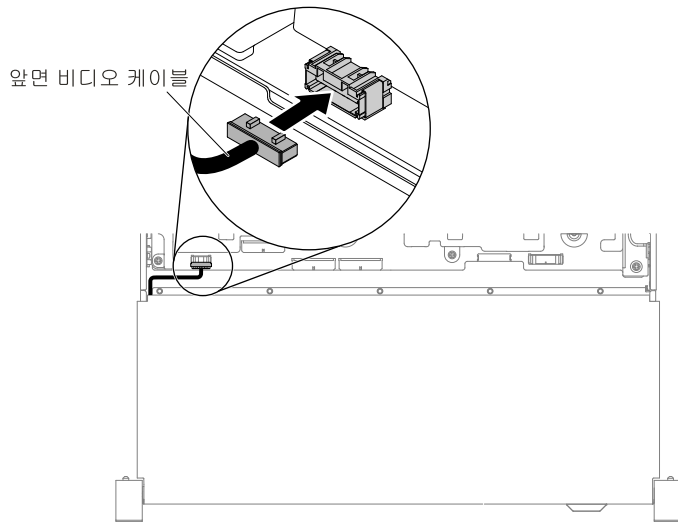
그림 186. 케이블 연결
