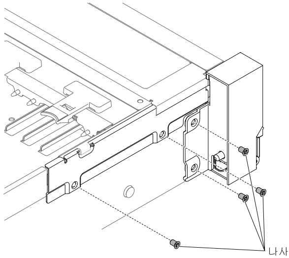
그림 174. 나사 설치
