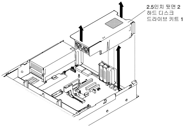
그림 136. 2.5인치 뒷면 2 하드 디스크 드라이브 키트 제거
