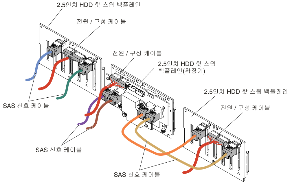
그림 278. 케이블 연결
