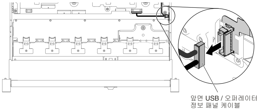
그림 147. 앞면 USB/오퍼레이터 정보 패널 케이블 제거
