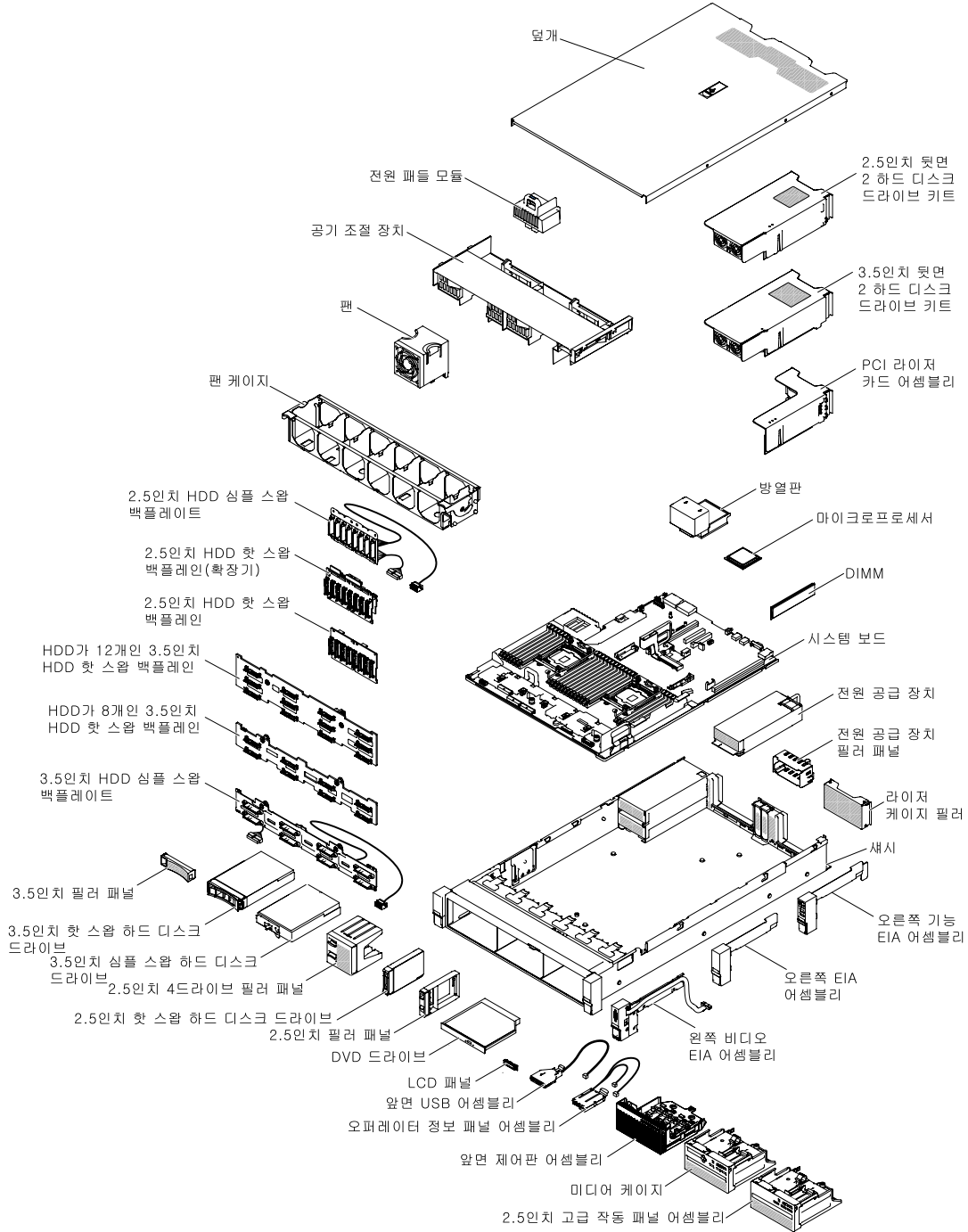
그림 26. 서버 구성 요소
