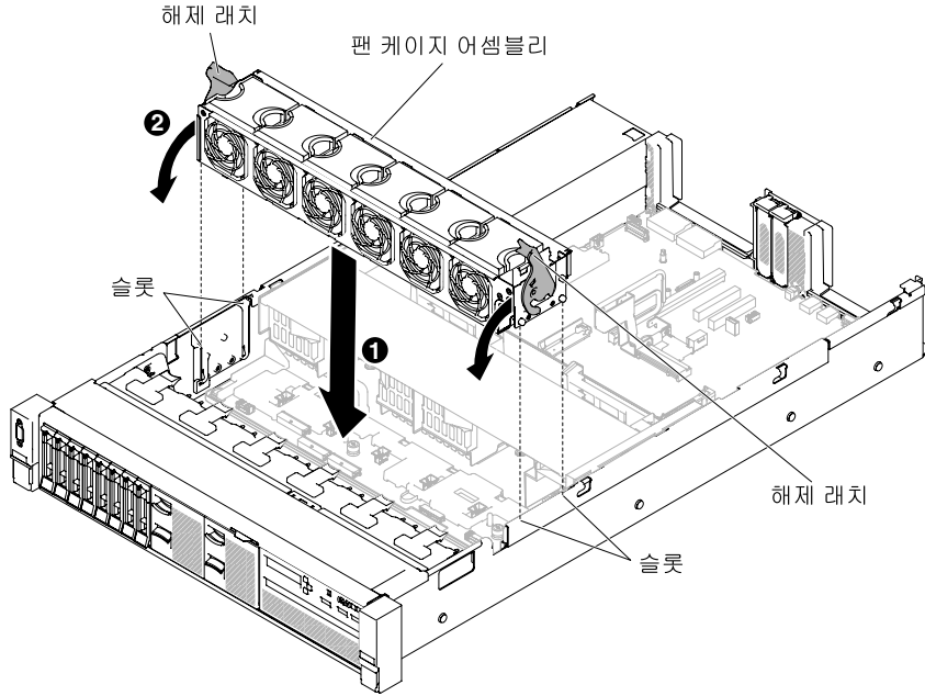
그림 102. 팬 케이스 어셈블리 설치
