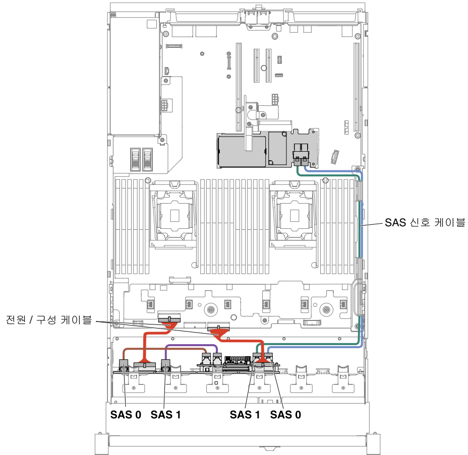
그림 277. 케이블 배선
