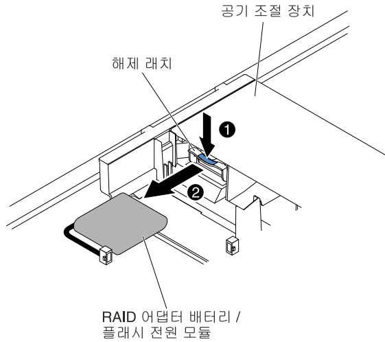
그림 133. RAID 어댑터 배터리/플래시 전원 모듈 제거
