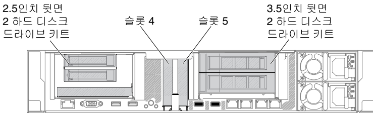
그림 126. PCI 라이저 카드 어댑터 확장 슬롯 위치
