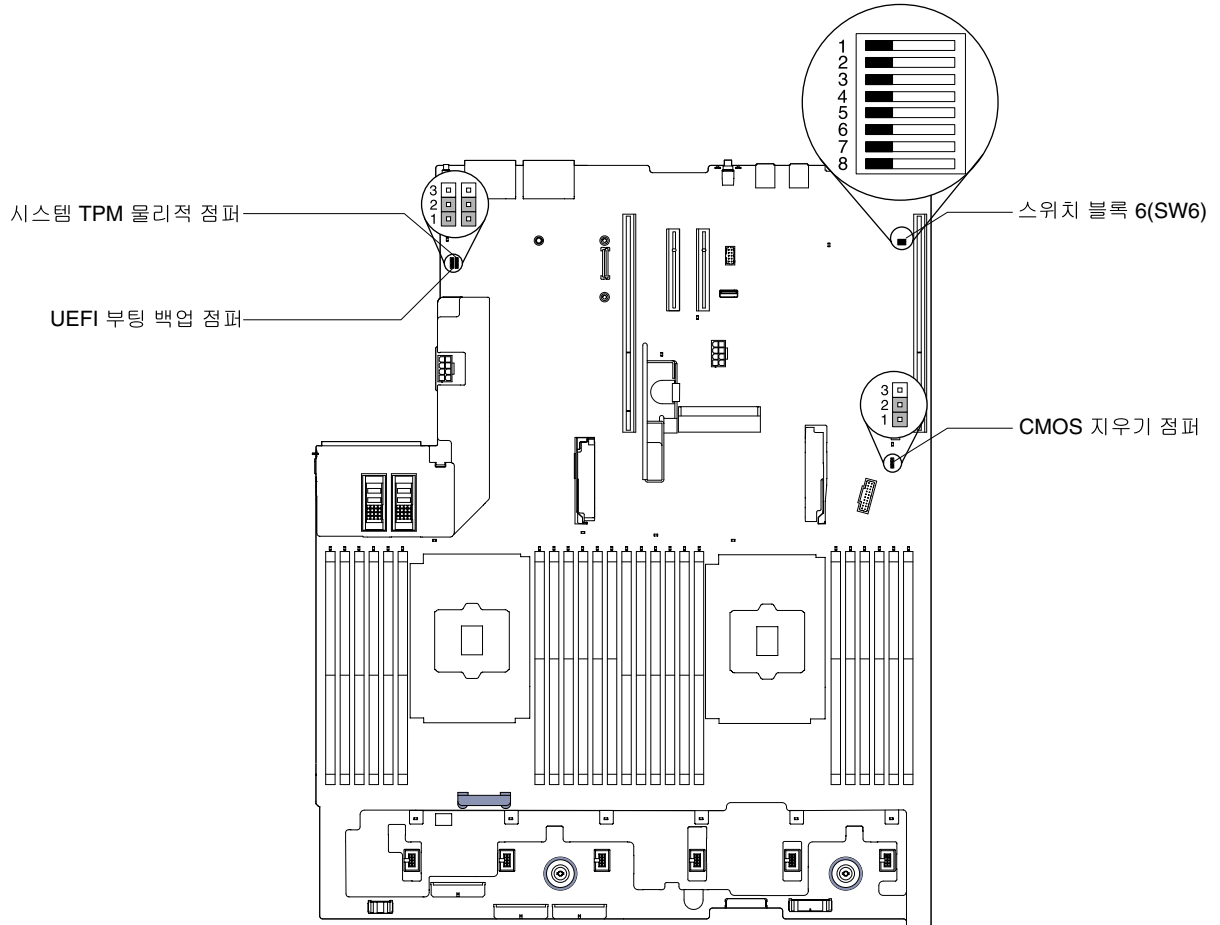
그림 49. UEFI 부팅 백업 점퍼(J15) 위치
