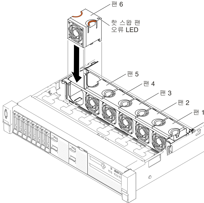
그림 104. 팬 설치
