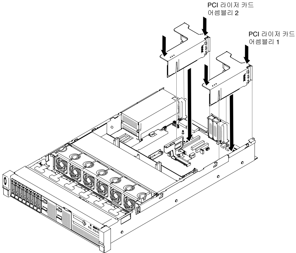
그림 113. 라이저 카드 어셈블리 설치 - 절반 길이 및 로우 프로파일 어댑터
