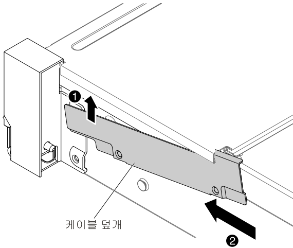
그림 179. 케이블 덮개 설치
