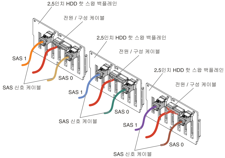
그림 270. 케이블 연결
