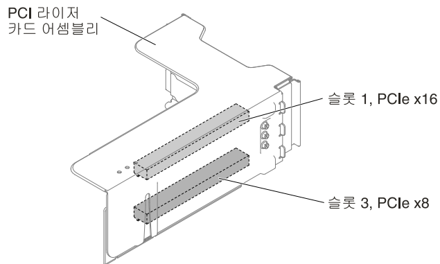
그림 34. 유형 3 PCI 라이저 카드
