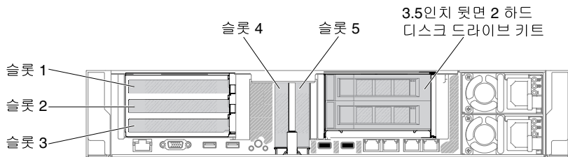
그림 24. PCI 라이저 카드 어댑터 확장 슬롯 위치
