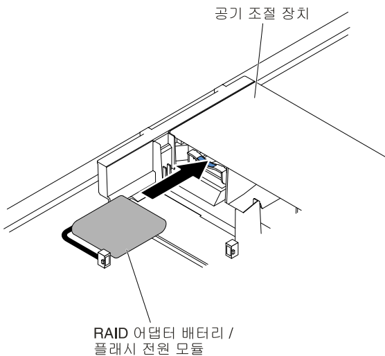
그림 135. RAID 어댑터 배터리/플래시 전원 모듈 설치
