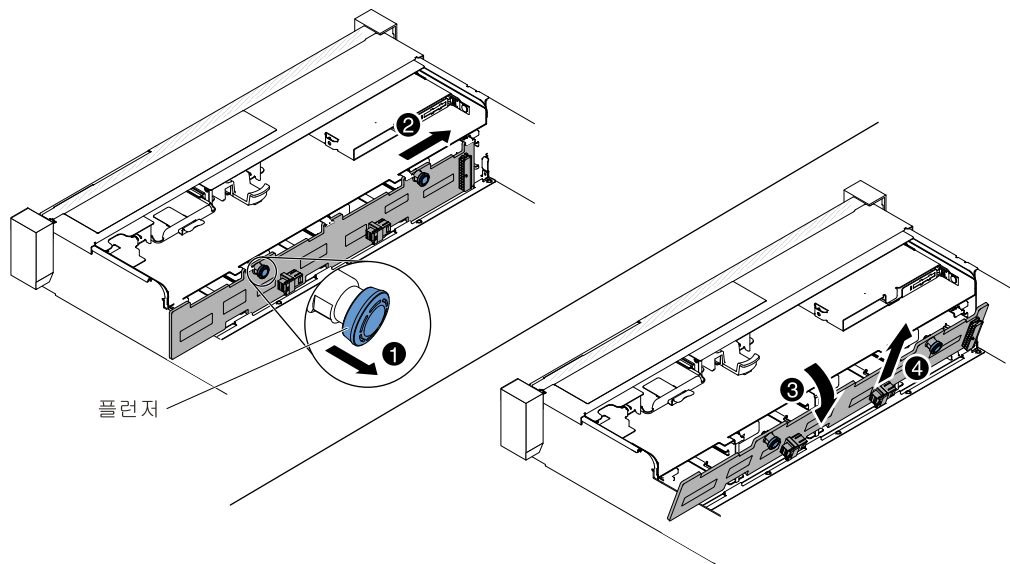
그림 196. 3.5인치 심플 스왑 백플레이트 어셈블리/핫 스왑 하드 디스크 드라이브 백플레이트 제거
