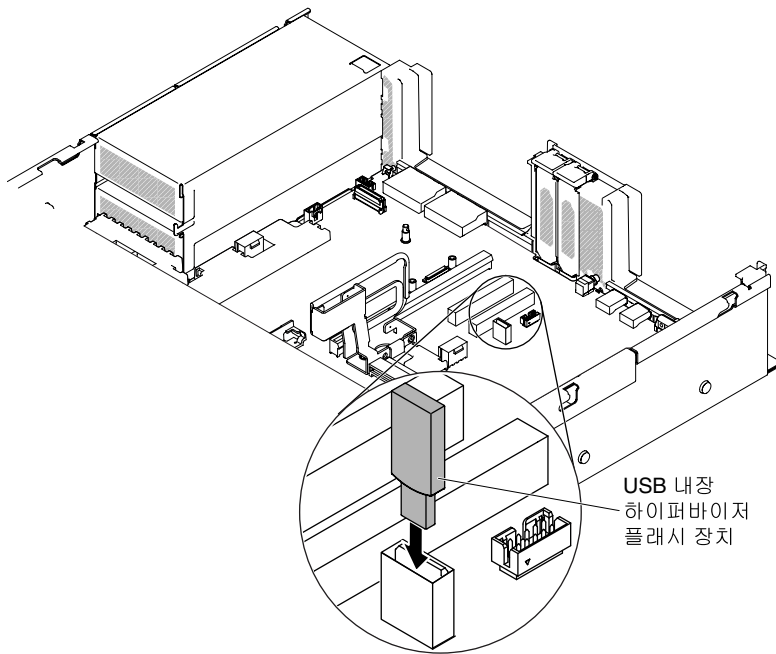
그림 201. USB 하이퍼바이저 플래시 장치 설치
