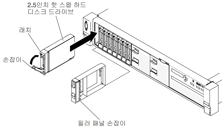
그림 82. 2.5인치 핫 스왑 하드 디스크 드라이브 설치
