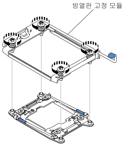
그림 257. 방열판 고정 모듈 설치
