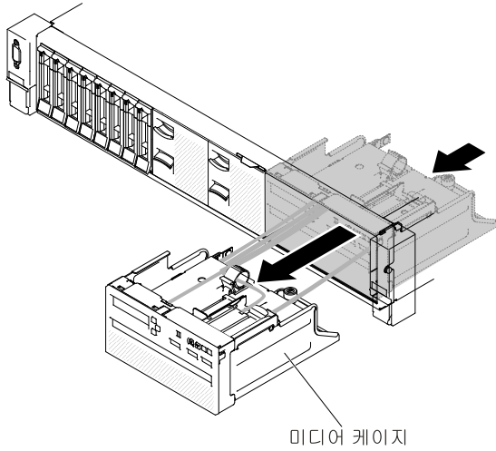
그림 107. 미디어 케이지 제거
