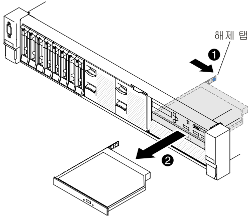
그림 92. 광 드라이브 제거
