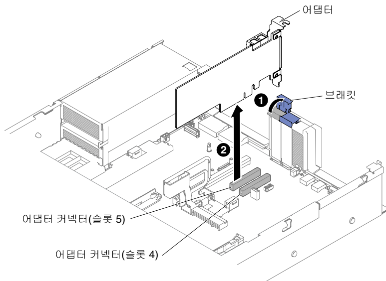
그림 122. 어댑터 제거
