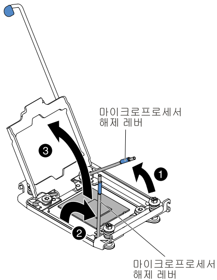
그림 235. 마이크로프로세서 소켓 레버 및 고정장치 분리
