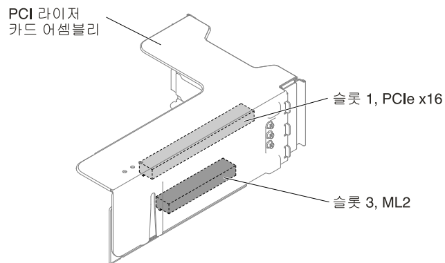
그림 35. 유형 4 PCI 라이저 카드
