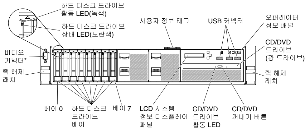
그림 12. 8 하드 디스크 드라이브 구성 / 16 하드 디스크 드라이브 구성 3: LCD 시스템 정보 디스플레이 패널, USB 커넥터 및 광 드라이브 포함
