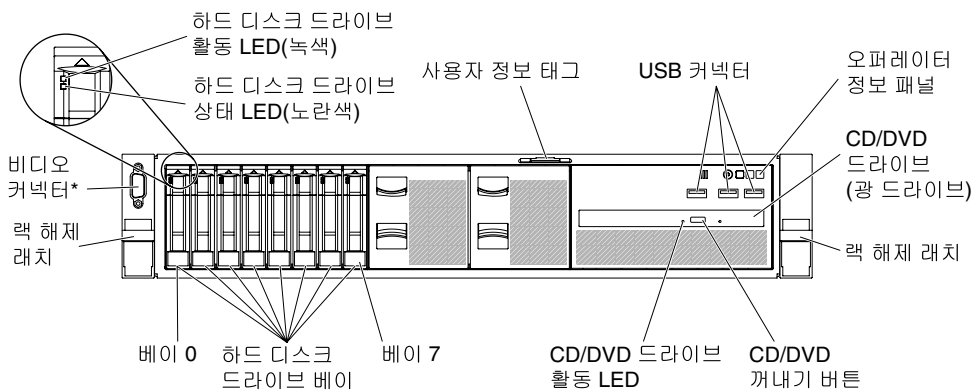
그림 11. 8 하드 디스크 드라이브 구성 / 16 하드 디스크 드라이브 구성 2: USB 커넥터 및 광 드라이브 포함
