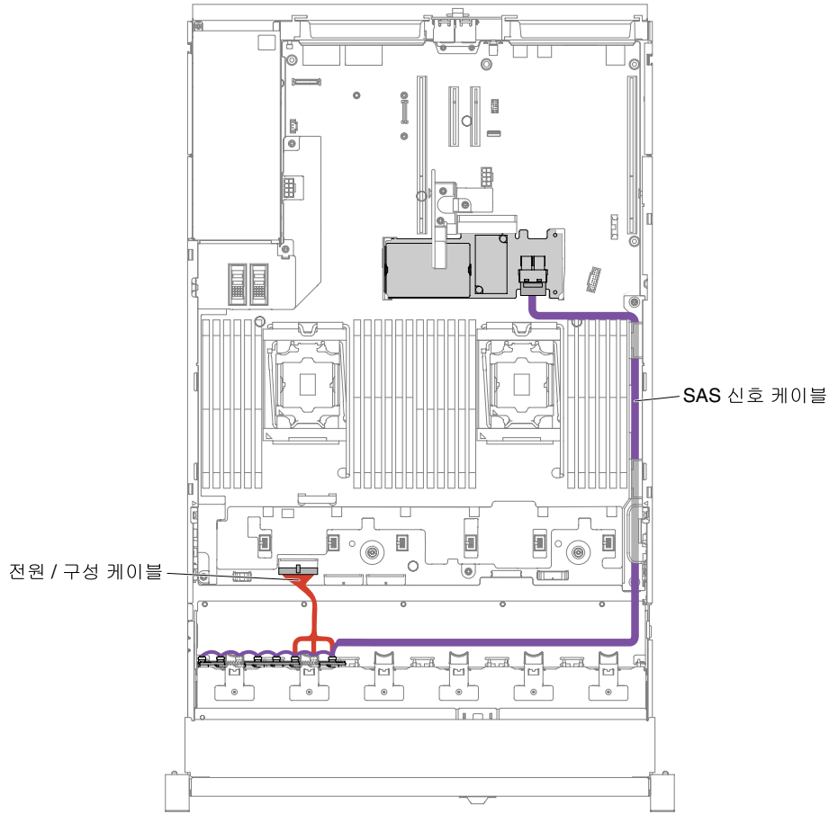
그림 52. 하드웨어 RAID 케이블이 연결된 8x2.5인치 심플 스왑 하드 디스크 드라이브
