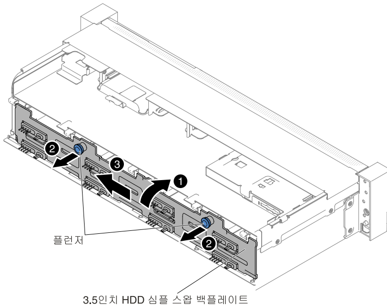
그림 264. 3.5인치 심플 스왑 백플레이트 어셈블리/핫 스왑 하드 디스크 드라이브 백플레인
