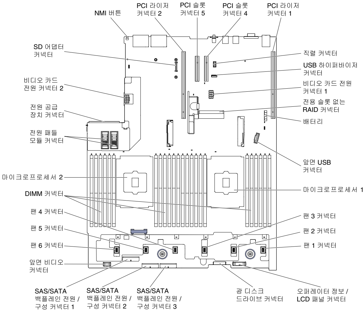
그림 27. 시스템 보드 내부 커넥터
