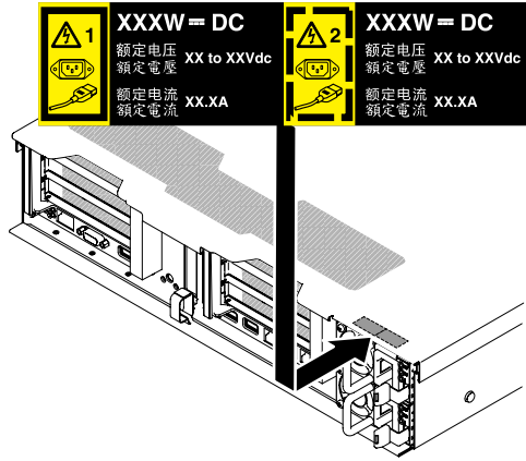
그림 193. 중복 전원 정보 레이블
