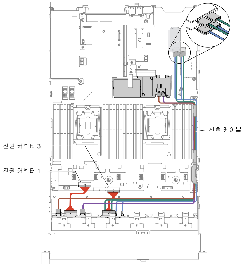
그림 286. 케이블 배선
