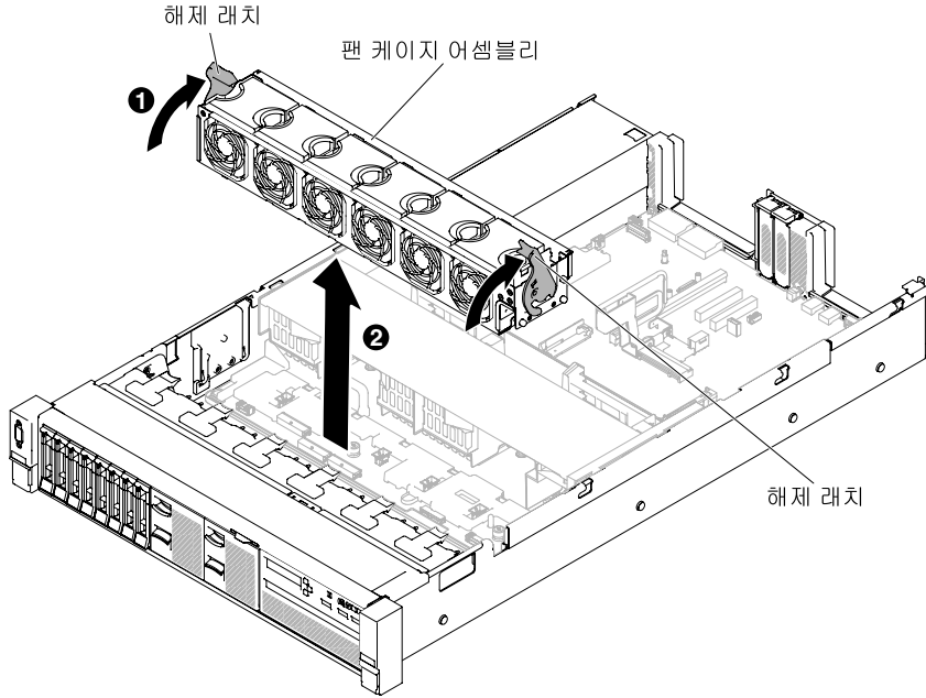
그림 101. 팬 케이지 어셈블리 제거
