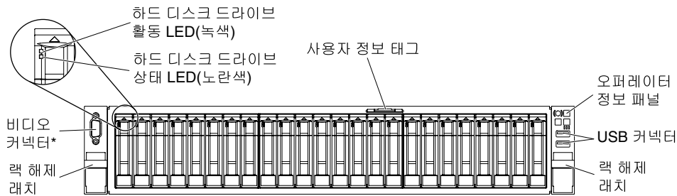
그림 13. 24 하드 디스크 드라이브 구성 앞면 보기
