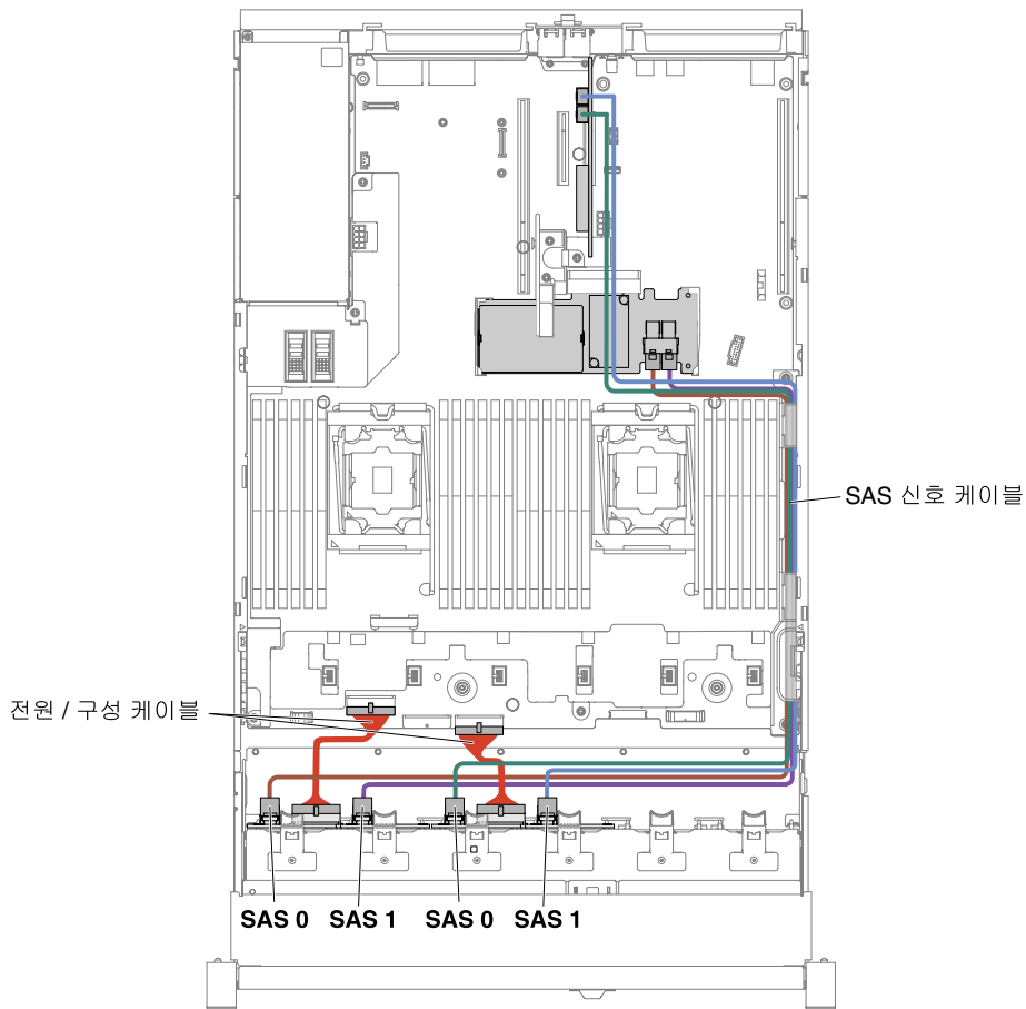
그림 57. 16x2.5인치 핫 스왑 하드 디스크 드라이브 케이블 연결
