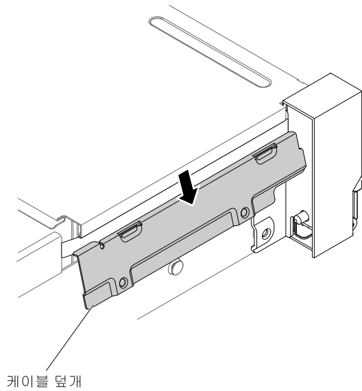
그림 163. 케이블 덮개 제거
