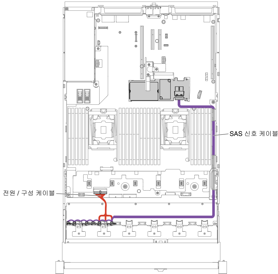
그림 263. 하드웨어 RAID 케이블이 연결된 8x2.5인치 심플 스왑 하드 디스크 드라이브
