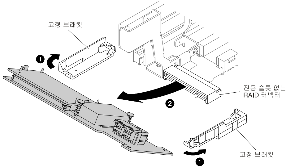
그림 115. 전용 슬롯 없는 RAID 컨트롤러 제거
