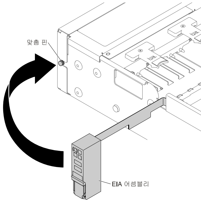
그림 166. EIA 어셈블리 정렬
