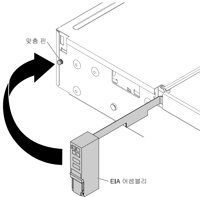
그림 177. EIA 어셈블리 정렬
