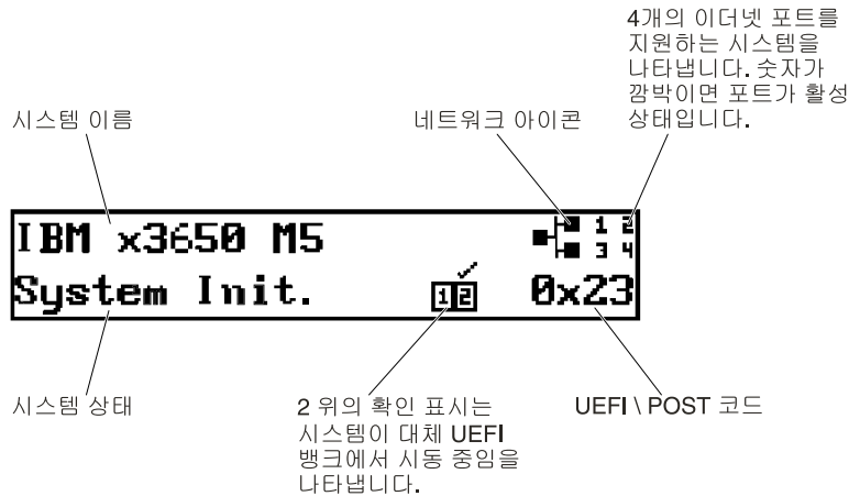
그림 20. 기본 메뉴
