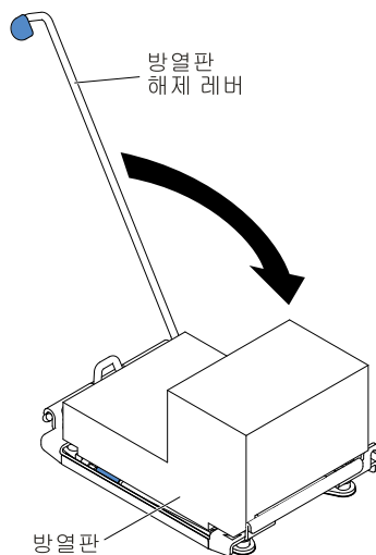
그림 253. 방열판 고정 모듈 해제 레버
