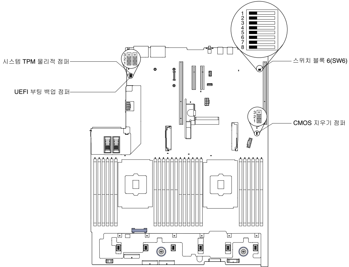
그림 30. 시스템 보드 스위치, 점퍼 및 버튼
