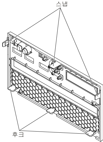
그림 218. 스냅(미디어 케이지 뒷면)
