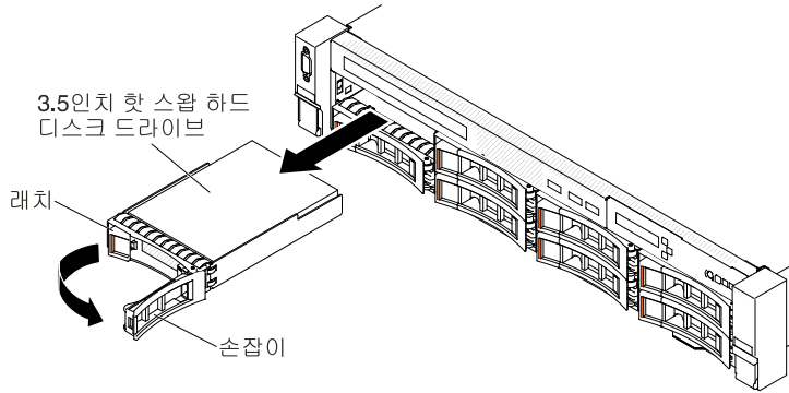
그림 81. 3.5인치 핫 스왑 하드 디스크 드라이브 제거
