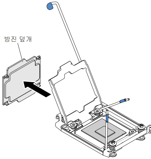
그림 248. 소켓 덮개 제거
