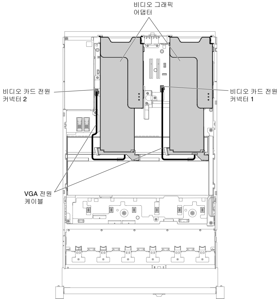
그림 51. VGA 전원 케이블 연결
