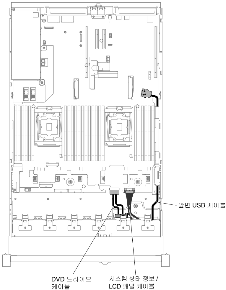
그림 110. 케이블 배선
