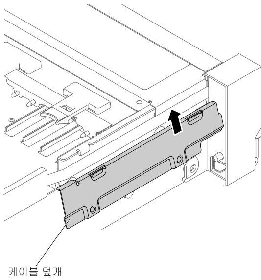
그림 173. 케이블 덮개 설치
