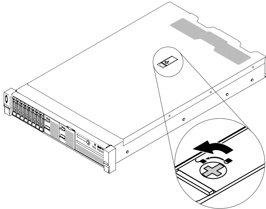
그림 69. 덮개 잠금 장치 나사 풀기
