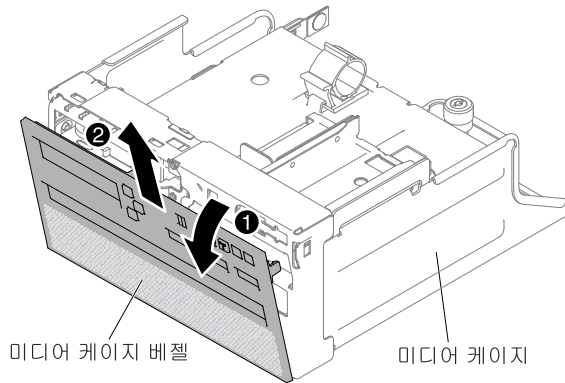
그림 219. 미디어 케이지 베젤 제거
