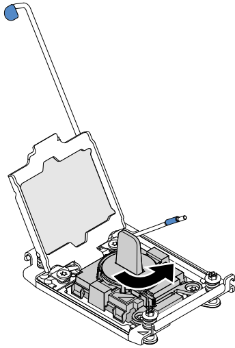
그림 245. 설치 도구 손잡이 조정
