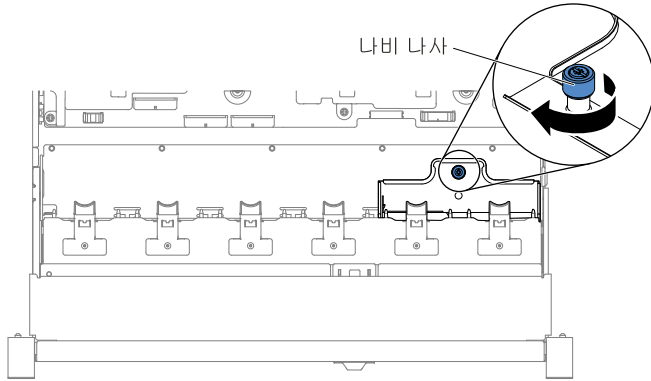
그림 109. 나비 나사
