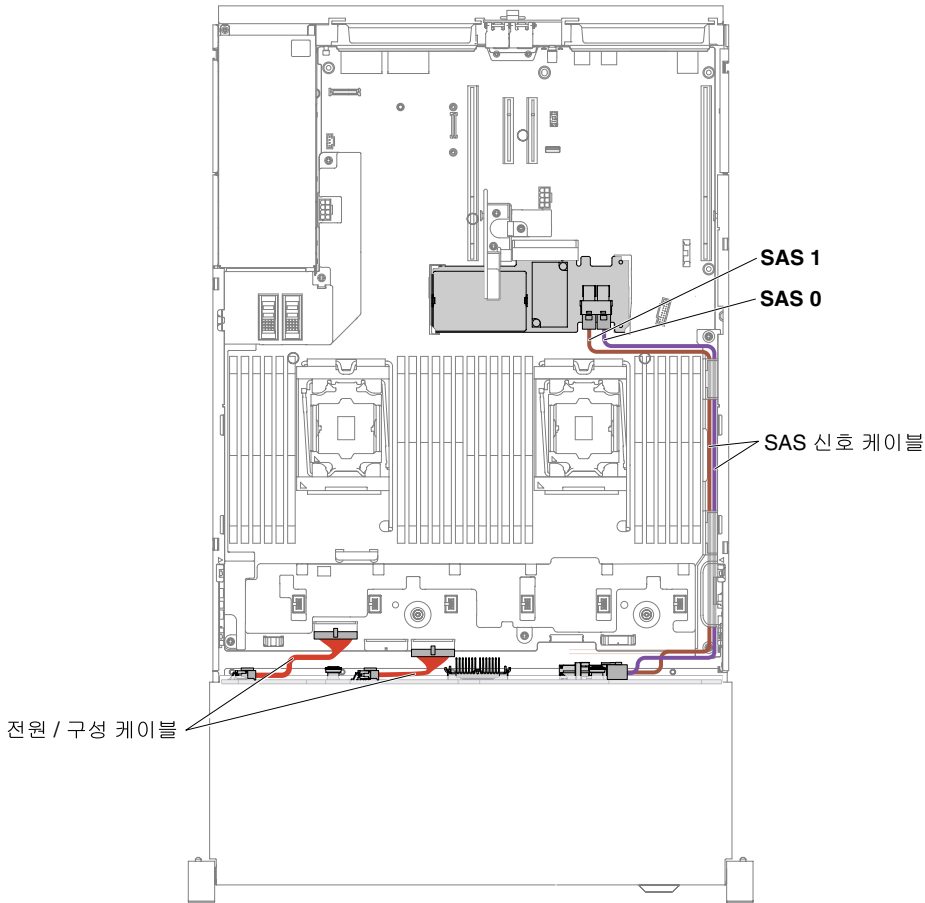
그림 68. 12x3.5인치 핫 스왑 하드 디스크 드라이브 케이블 연결
