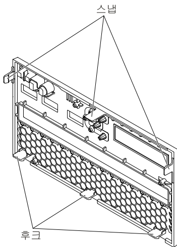
그림 223. 후크(미디어 케이지 뒷면)
