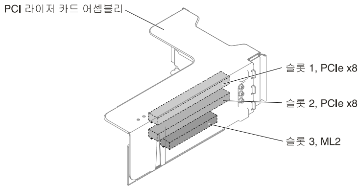
그림 33. 유형 2 PCI 라이저 카드
