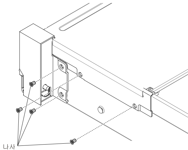
그림 157. 나사 제거
