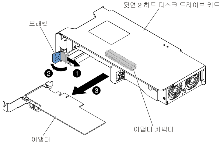
그림 123. 어댑터 제거
