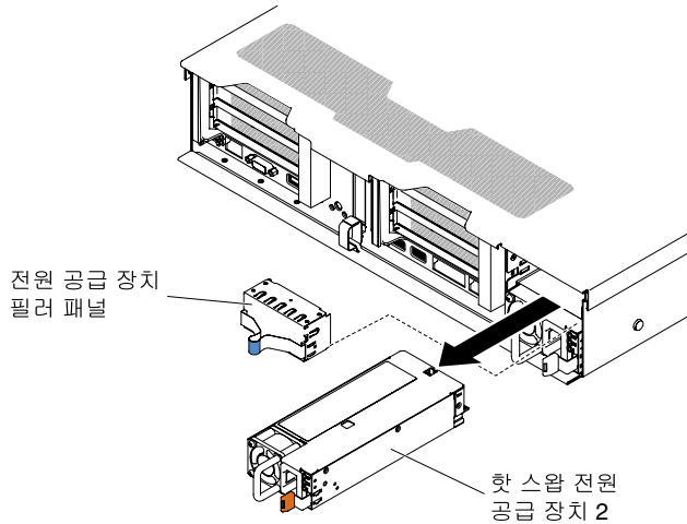
그림 187. 전원 공급 장치 제거
