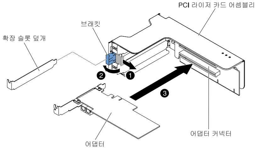
그림 127. 어댑터 설치
