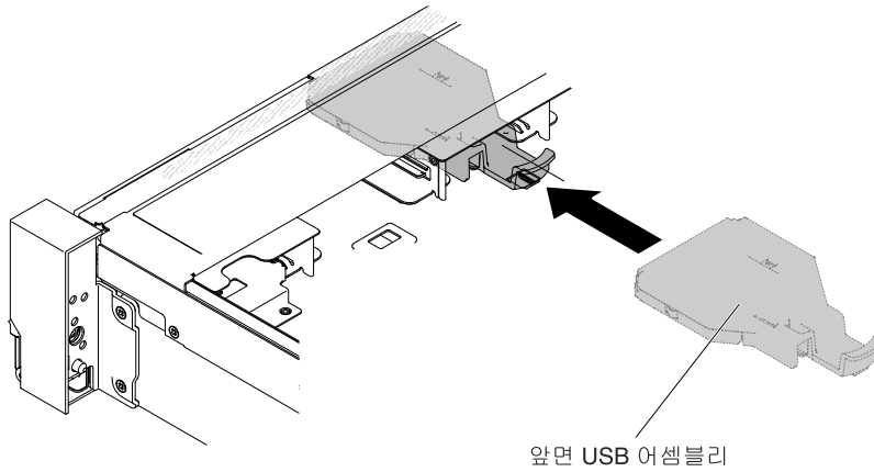
그림 78. 앞면 USB 어셈블리 설치
