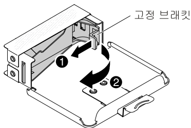
그림 209. 고정 브래킷 제거
