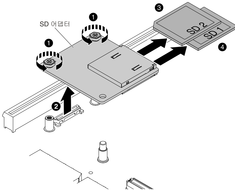
그림 206. SD 어댑터 제거
