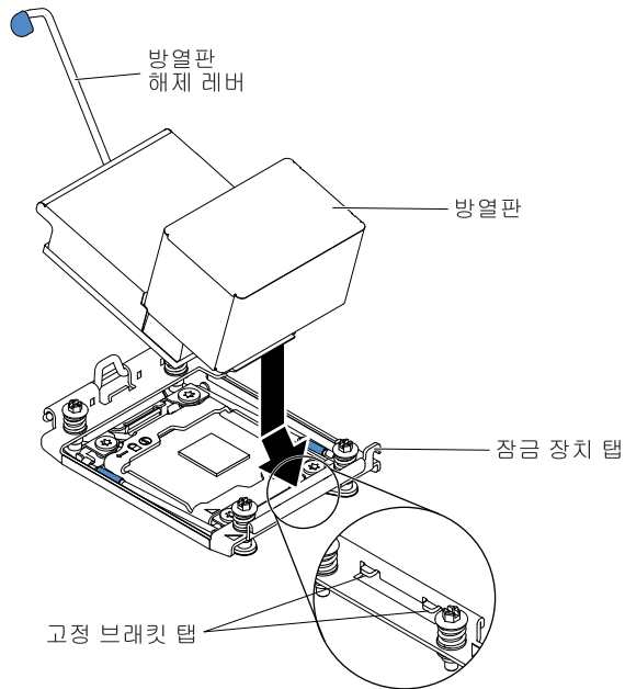
그림 252. 방열판 설치
