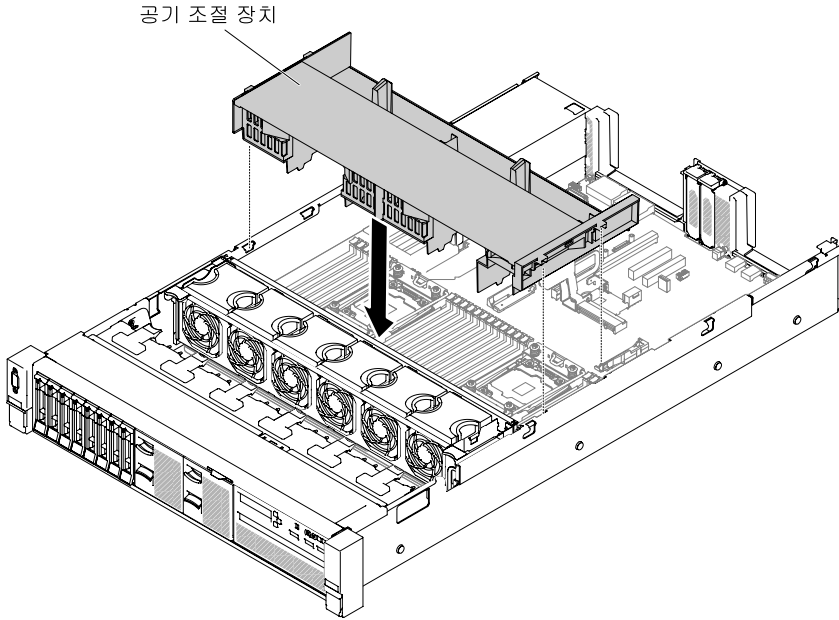
그림 74. 공기 조절 장치 설치
