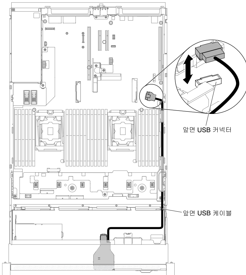
그림 79. 앞면 USB 어셈블리 케이블 배선
