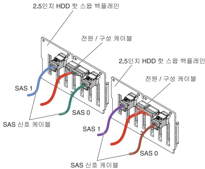
그림 268. 케이블 연결
