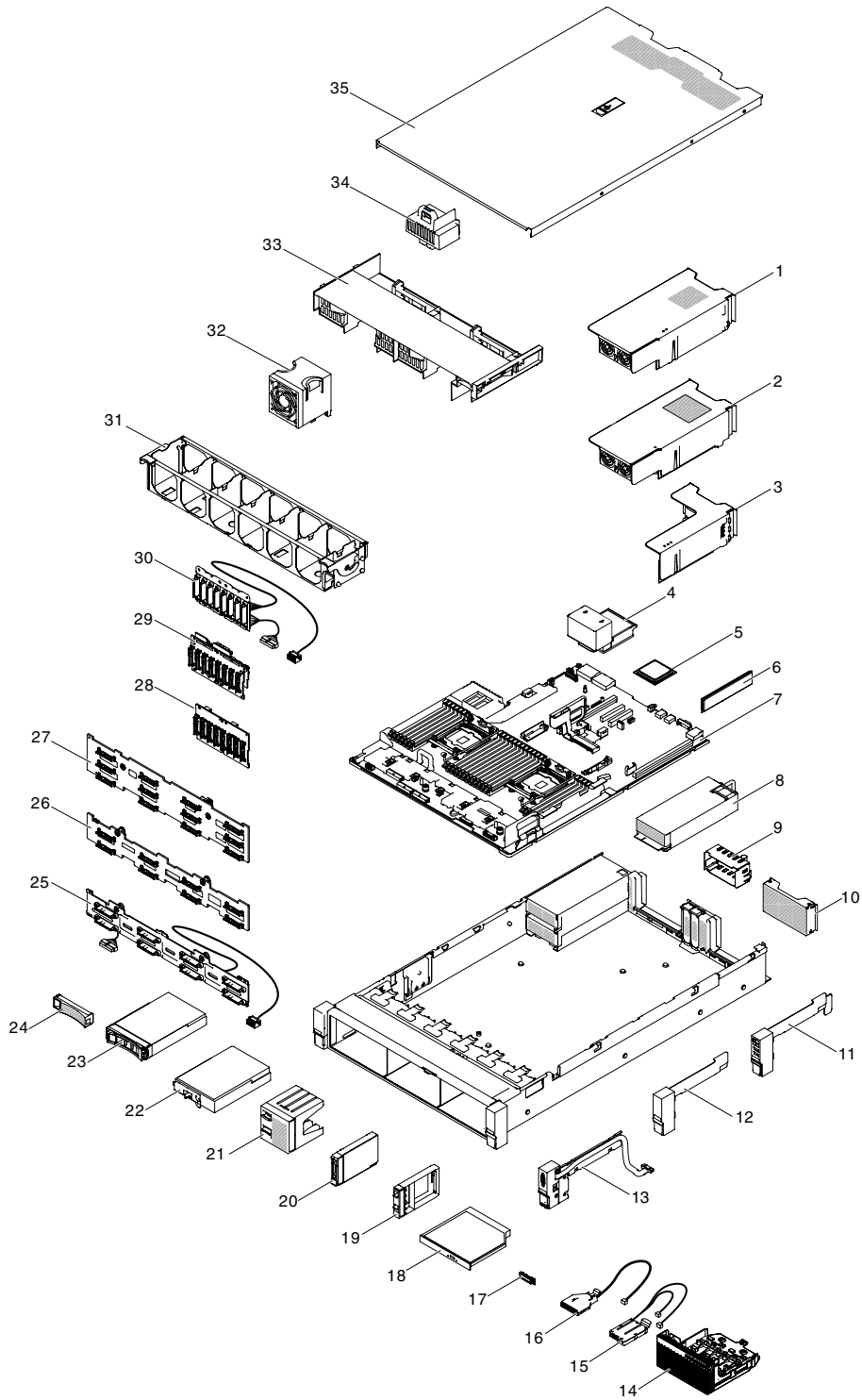
그림 50. 서버 구성 요소
