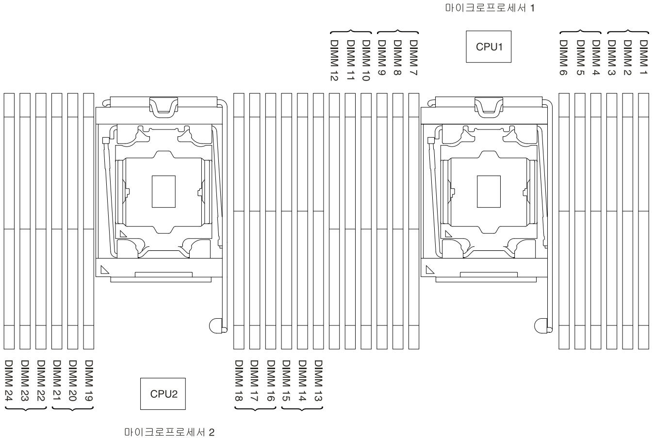
그림 97. DIMM 커넥터 위치
