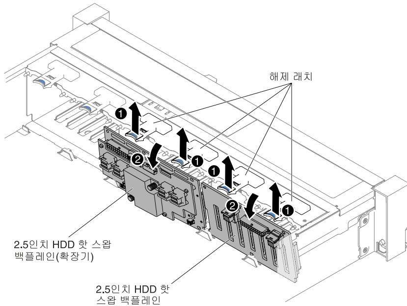
그림 194. 2.5인치 심플 스왑 백플레이트 어셈블리/핫 스왑 하드 디스크 드라이브 백플레인 제거
