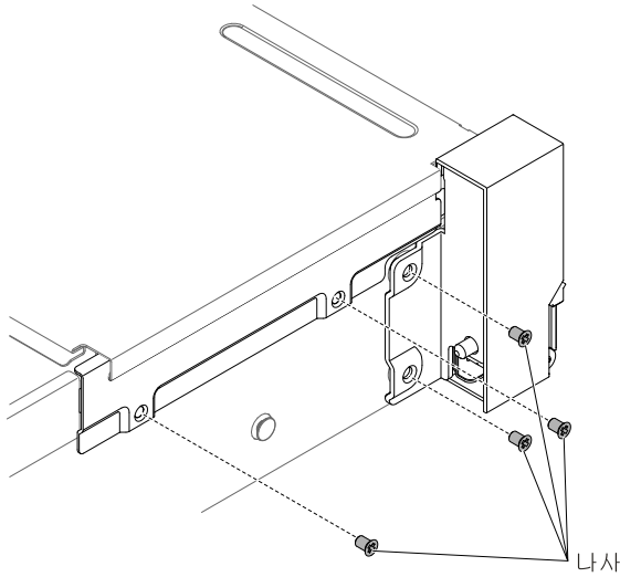
그림 185. 나사 설치
