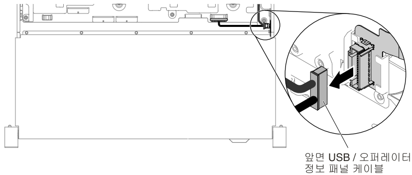
그림 156. 앞면 USB/오퍼레이터 정보 패널 케이블 제거
