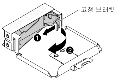
그림 213. 고정 브래킷 제거
