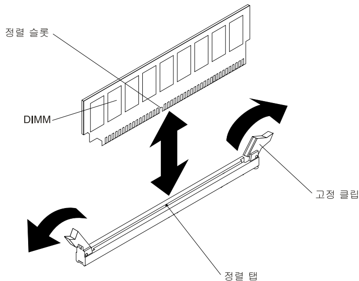
그림 100. DIMM 설치
