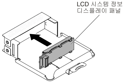
그림 214. LCD 시스템 정보 디스플레이 패널 설치
