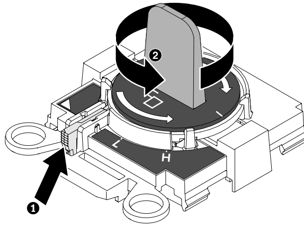
그림 236. 설치 도구 손잡이 조정
