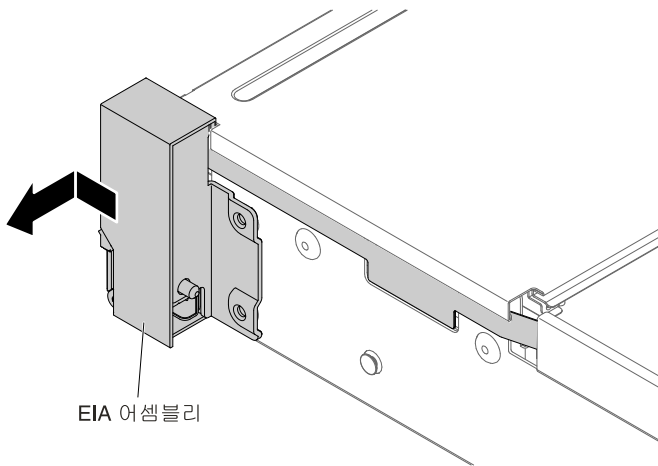
그림 159. EIA 어셈블리 제거
