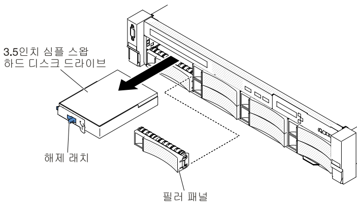
그림 85. 3.5인치 심플 스왑 하드 디스크 드라이브 제거
