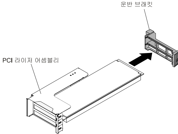
그림 120. 전체 높이, 전체 길이 어댑터
