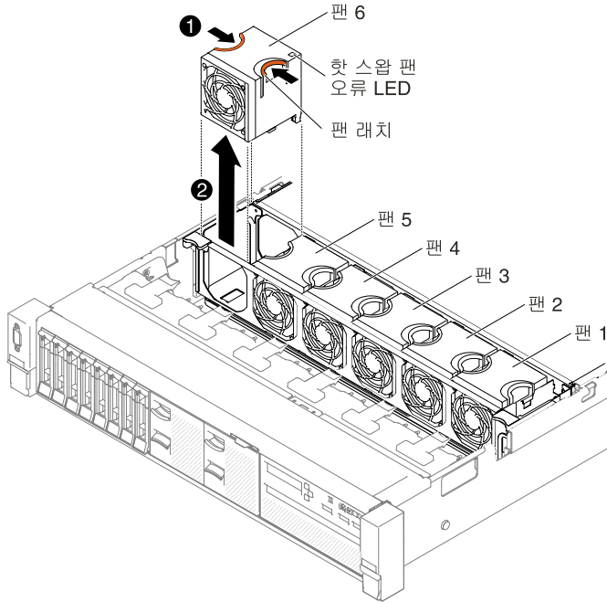
그림 103. 팬 제거
