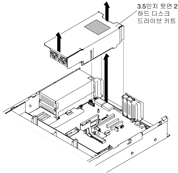
그림 137. 3.5인치 뒷면 2 하드 디스크 드라이브 키트 제거
