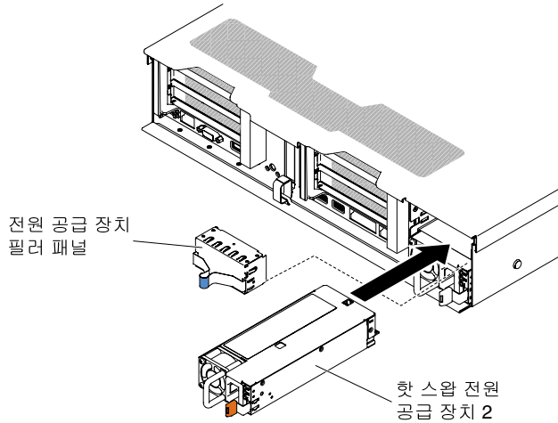
그림 188. 전원 공급 장치 설치
