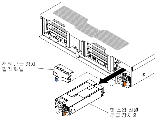
그림 190. 전원 공급 장치 제거
