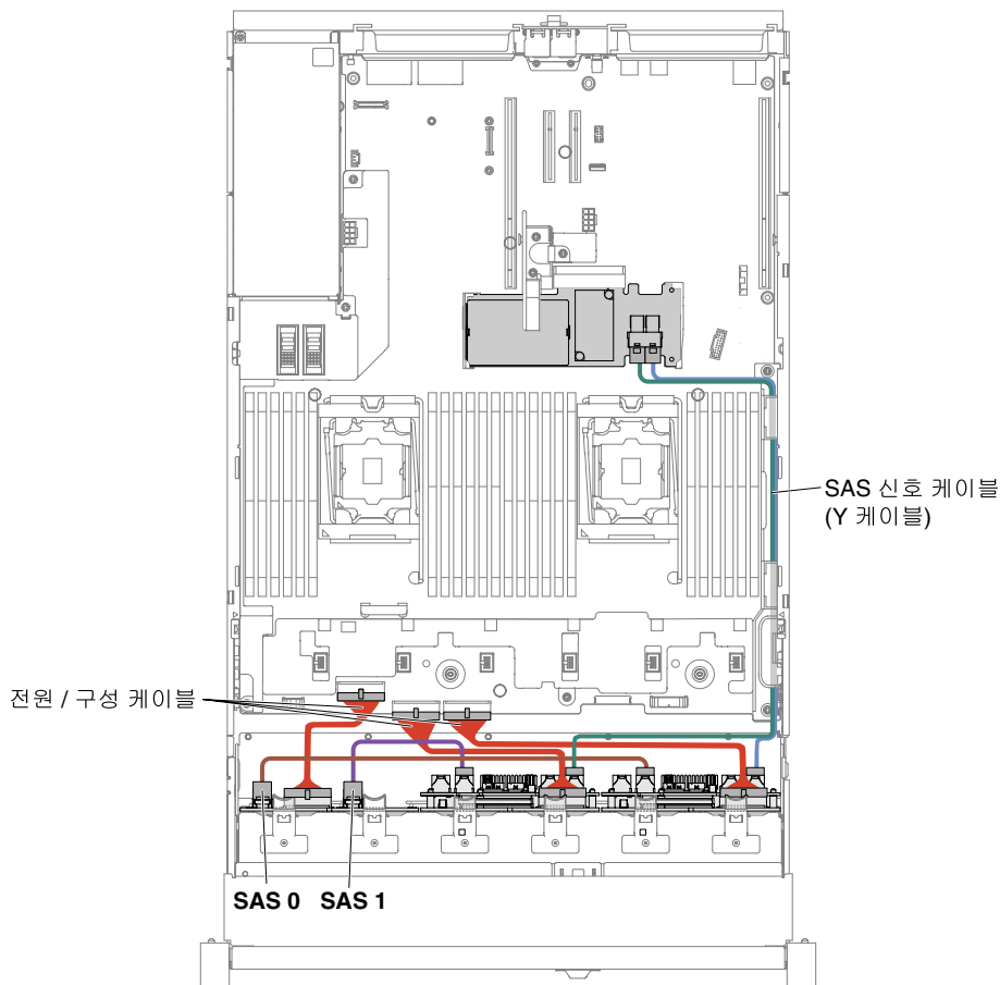
그림 65. 24x2.5인치 핫 스왑 하드 디스크 드라이브 케이블 연결
