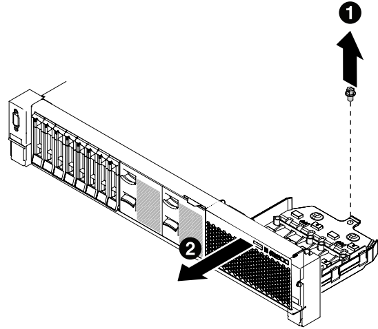
그림 289. 앞면 제어판 어셈블리 제거
