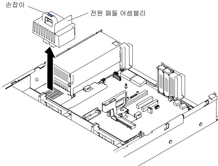
그림 75. 전원 패들 모듈 제거
