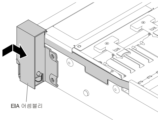
그림 167. EIA 어셈블리 설치
