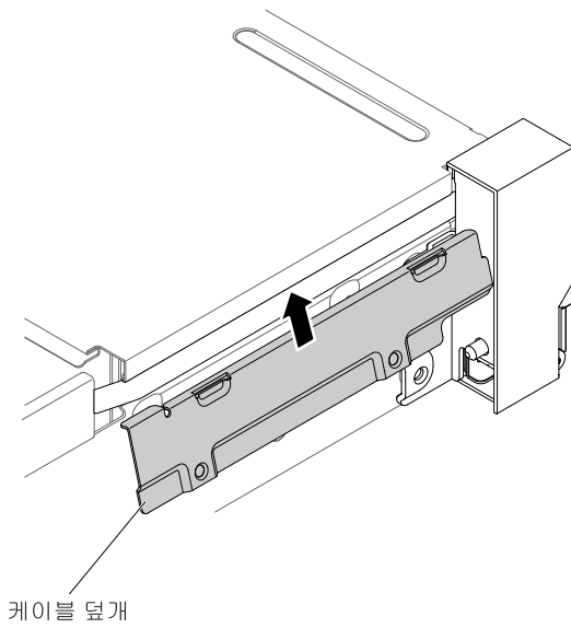
그림 184. 케이블 덮개 설치
