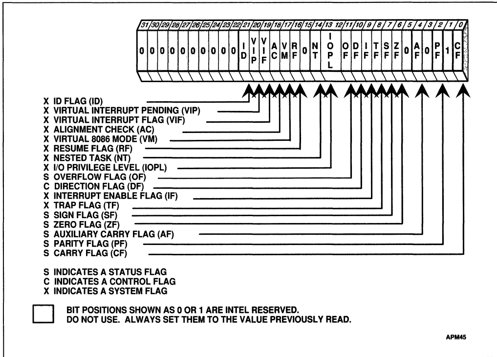
Figure 3-9. EFLAGS Register
