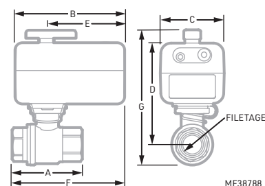
Fig. 1. Schéma dimensionnel.
