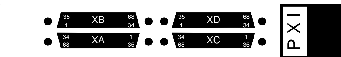
Abbildung 2-3: Frontplatte PXI 31128 mit Anordnung der Steckverbinder
