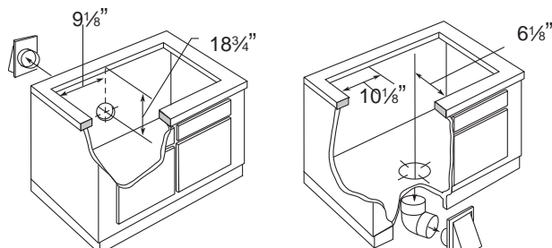
Ventilation par le mur arrière
