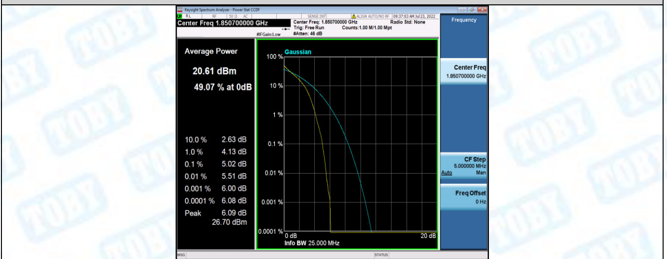
Band25-1.4MHz-QPSK-26365-1RB#0
