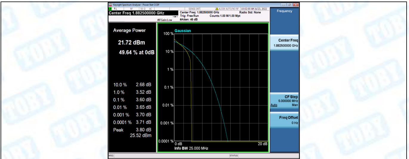
Band25-3MHz-QPSK-26365-15RB#0
