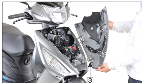
(3) Lugs
